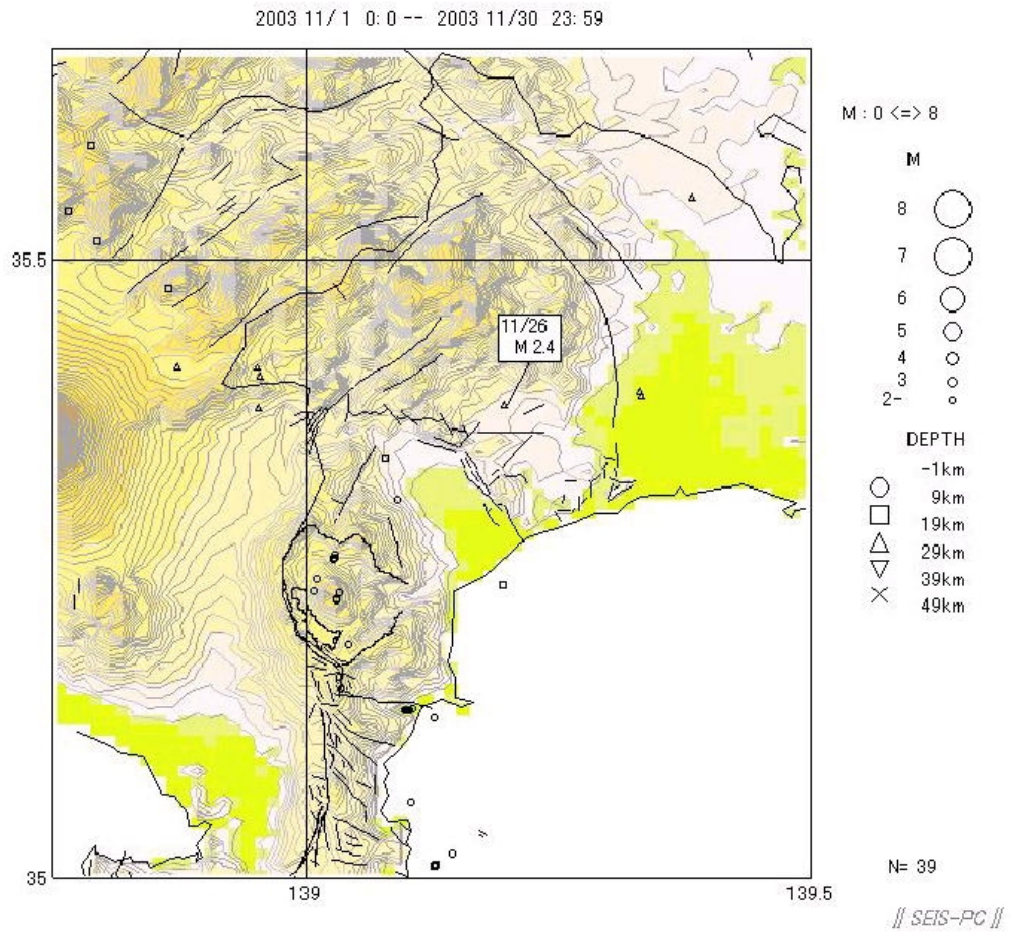
図1 箱根及び県西部地域の地震活動（11月分） （作図には、SEIS-PC for Windows95を用いた）
