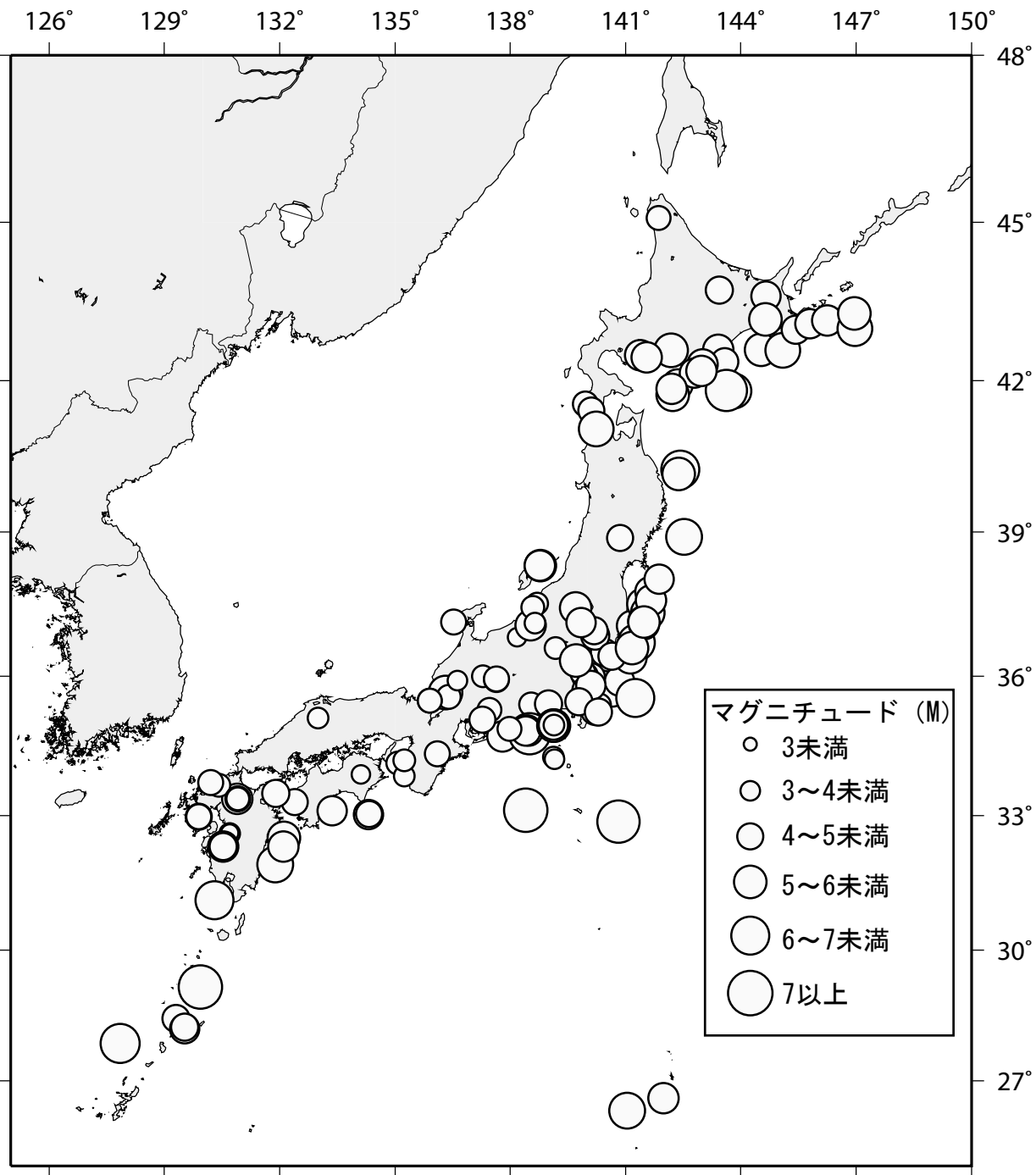
図1 震源分布 (平成21年1月1日~12月31日)
