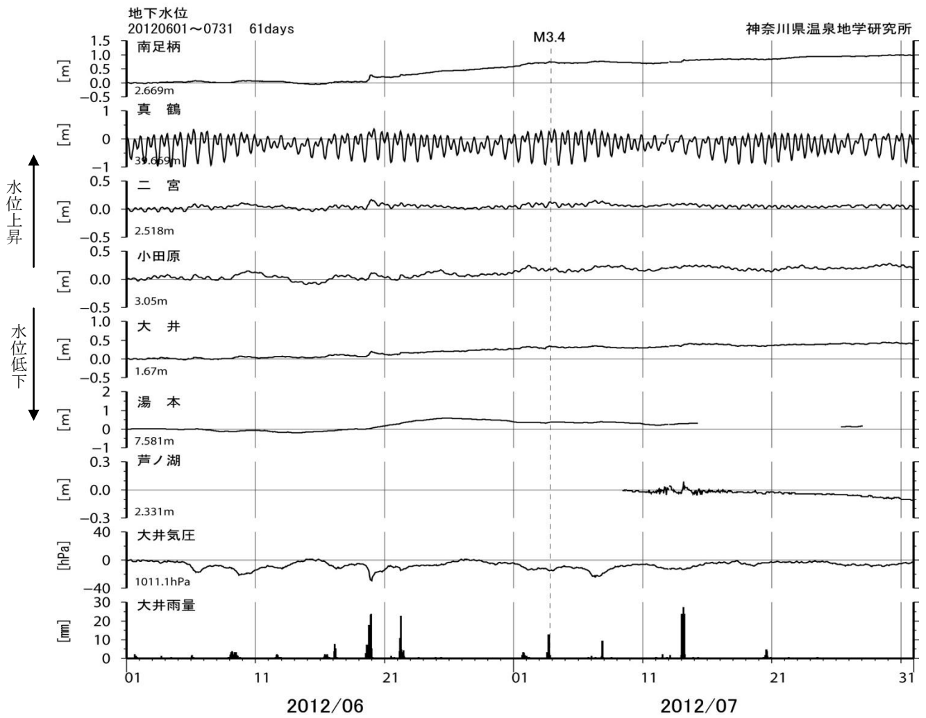
図6 地下水水位観測結果(2012年6~7月)
