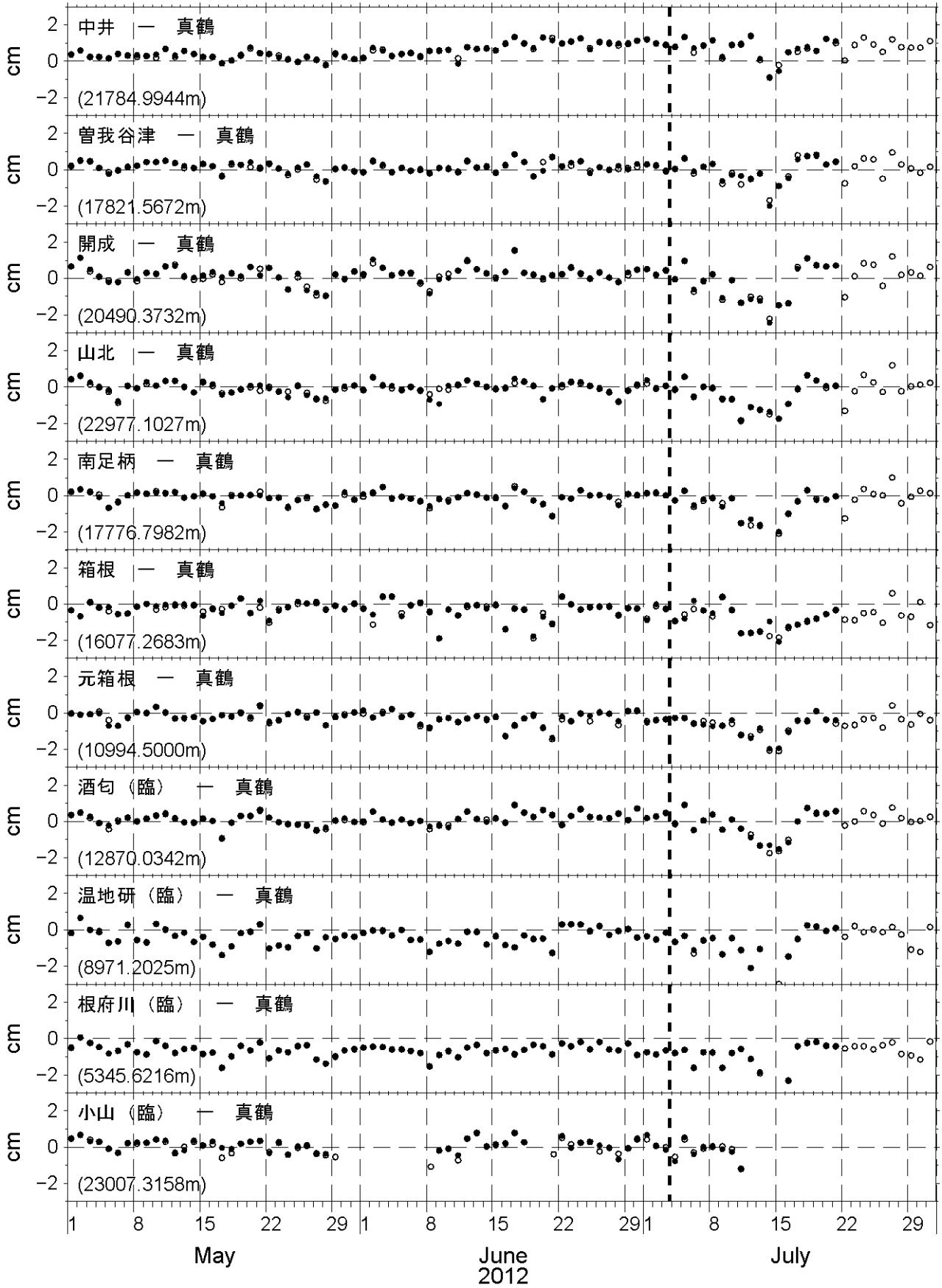
図4 GPS測量観測結果 (2012年05月01日~07月31日)
