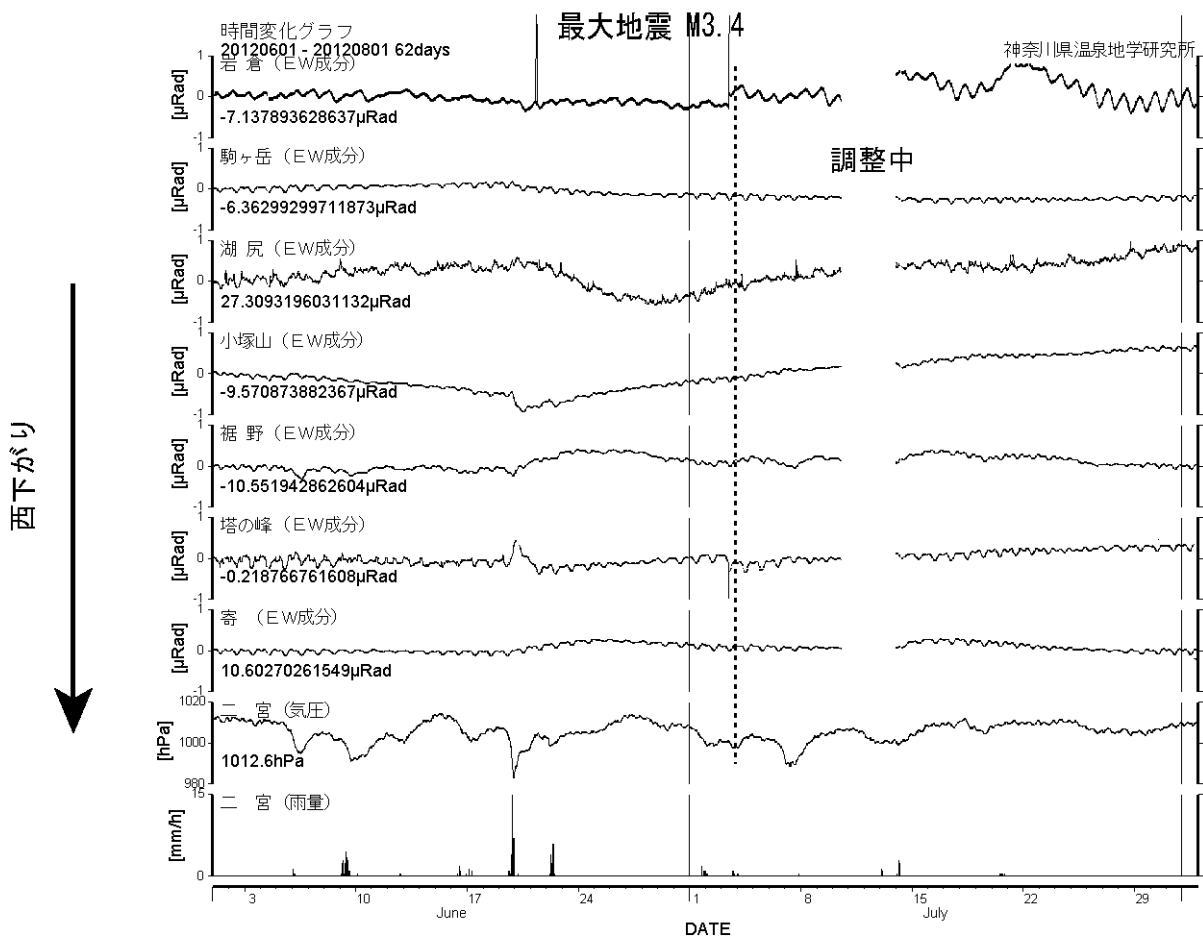
図3 傾斜計記録 (2012年6月1日から8月1日) 上: 南北成分 下: 東西成分 最大地震 [1] 012年7月03日22時20分 深さ14.91 km M3.4 (足柄平野)
