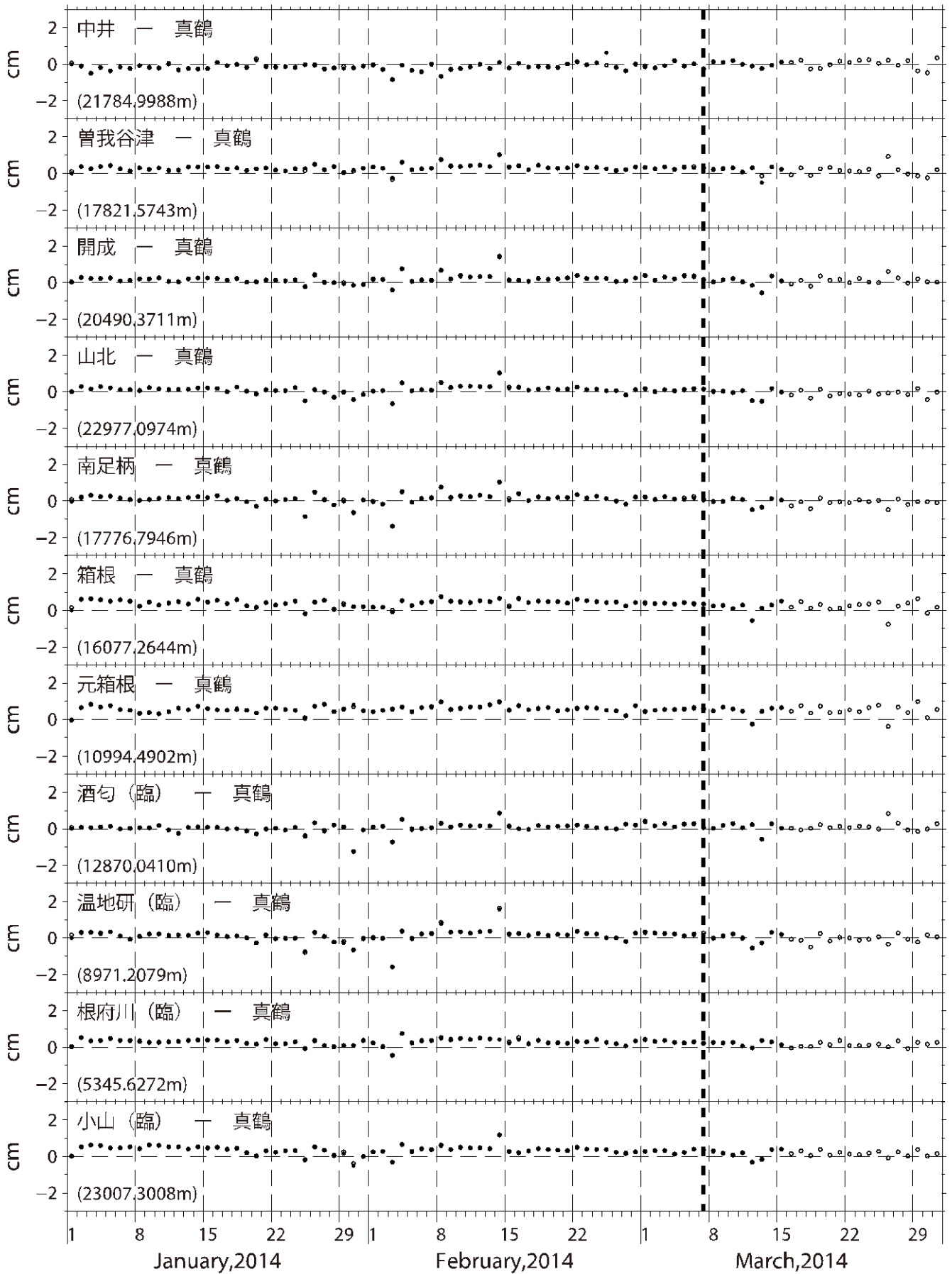
図4 GPS測量観測結果 (2014年 1月 1日~2014年 3月31日)
