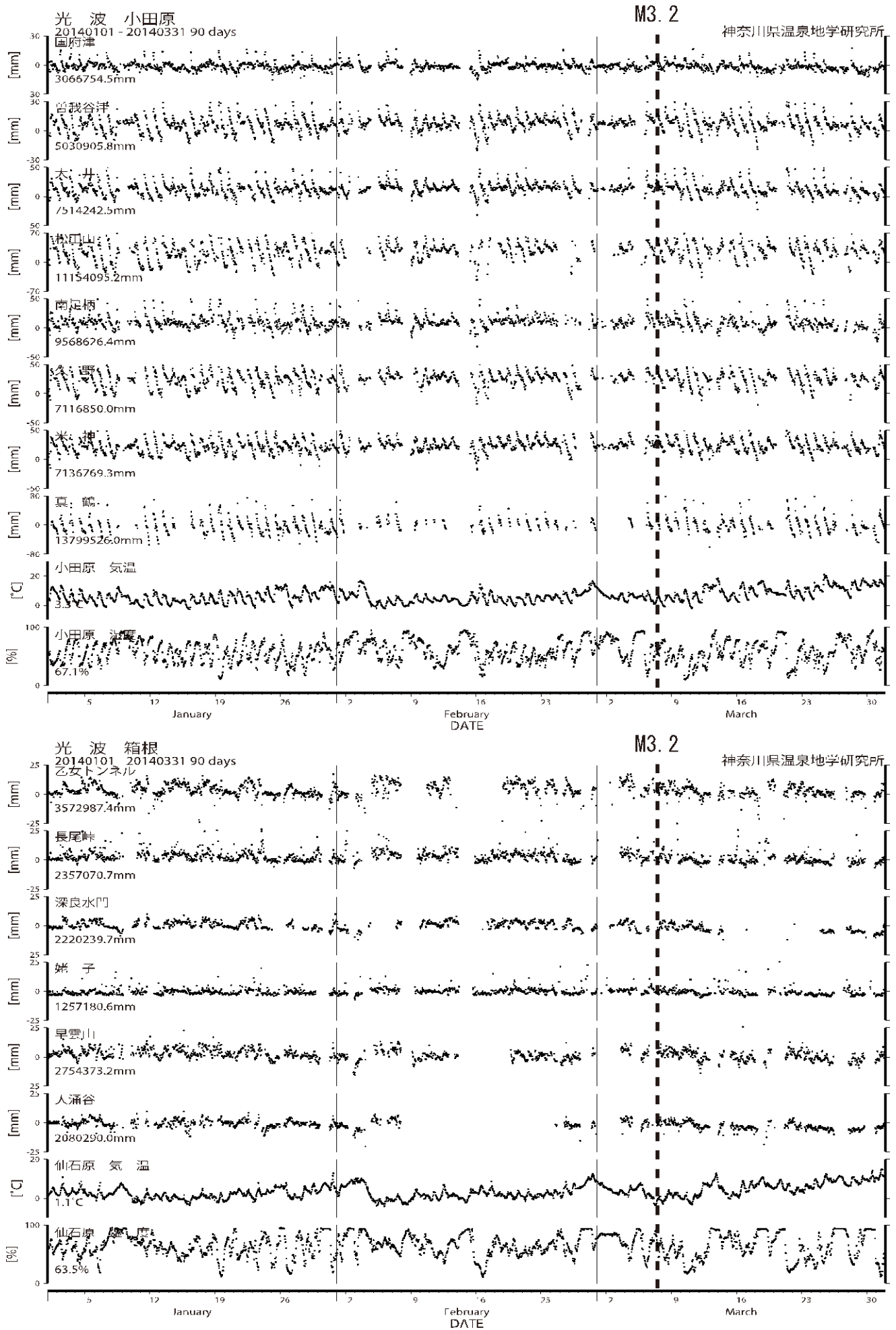
図5 光波測量観測結果 (2014年 1月 1日~2014年 3月31日) 上：小田原観測網、下：箱根観測網
