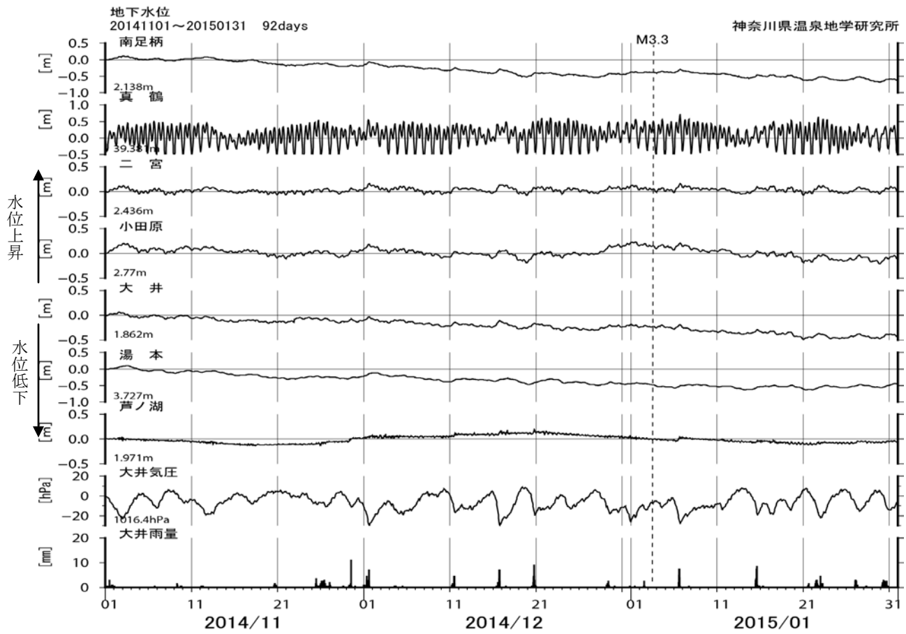
図6 地下水位観測結果(2014年11月~2015年1月)
