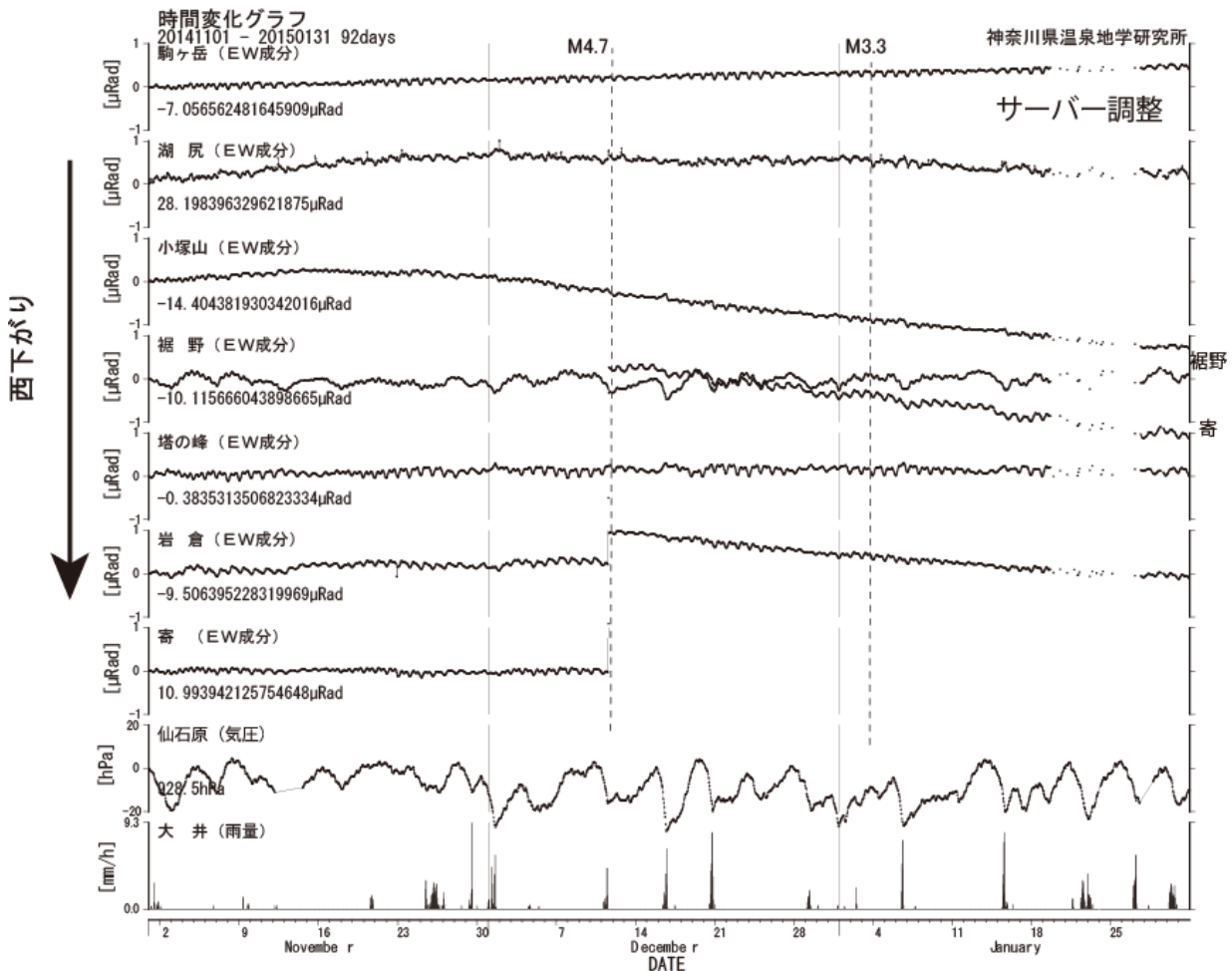
図3 傾斜計記録(2014年11月1日から2015年1月31日) 上:南北成分 下:東西成分
