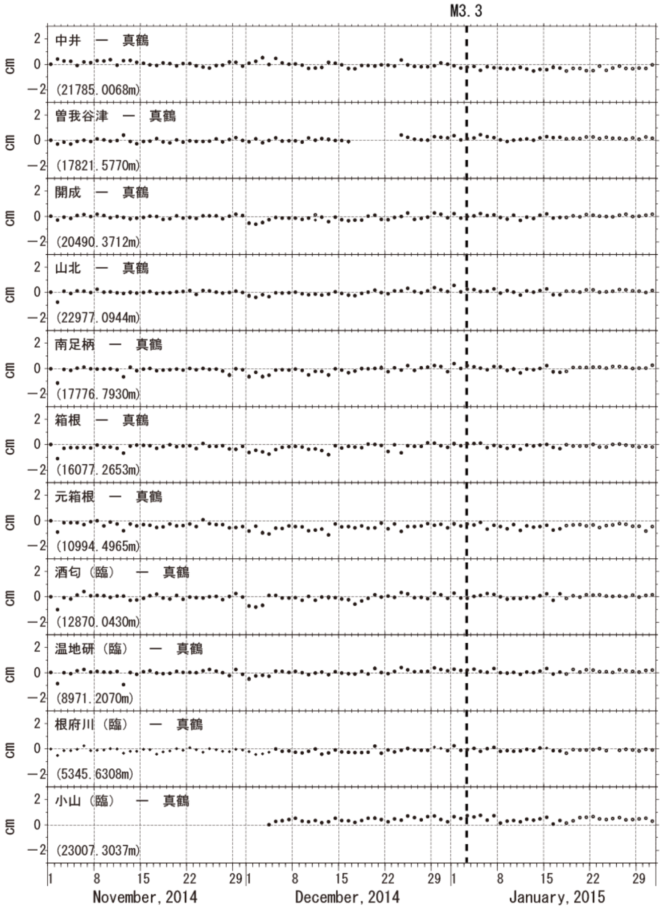
図4 GPS測量観測結果（2014年11月01日～2015年01月31日）
