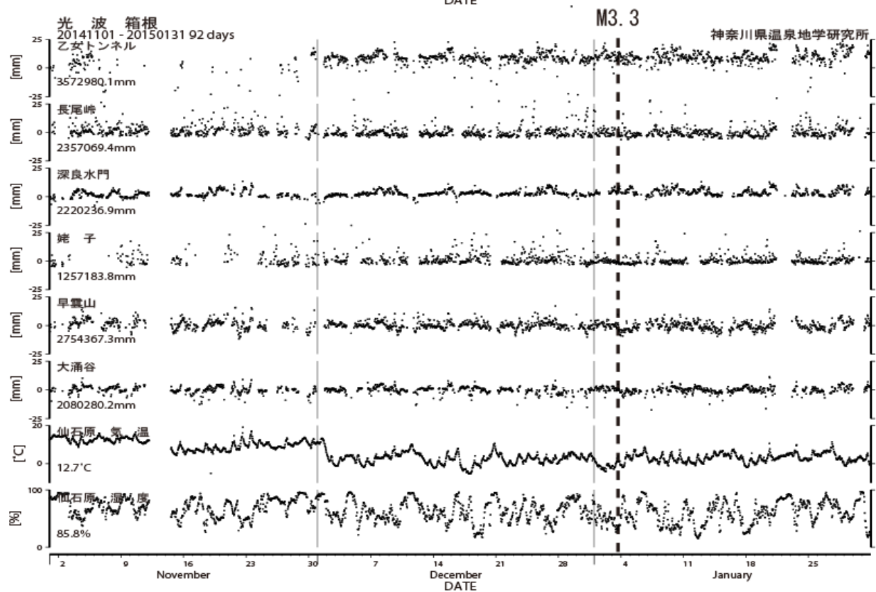
図5 光波測量観測結果 (2014年11月01日~2015年01月31日) 上: 小田原観測網、下: 箱根観測網
