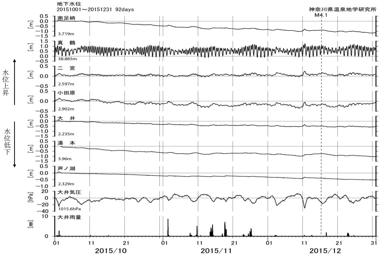
図6 地下水位観測結果(2015年10月~2015年12月)
