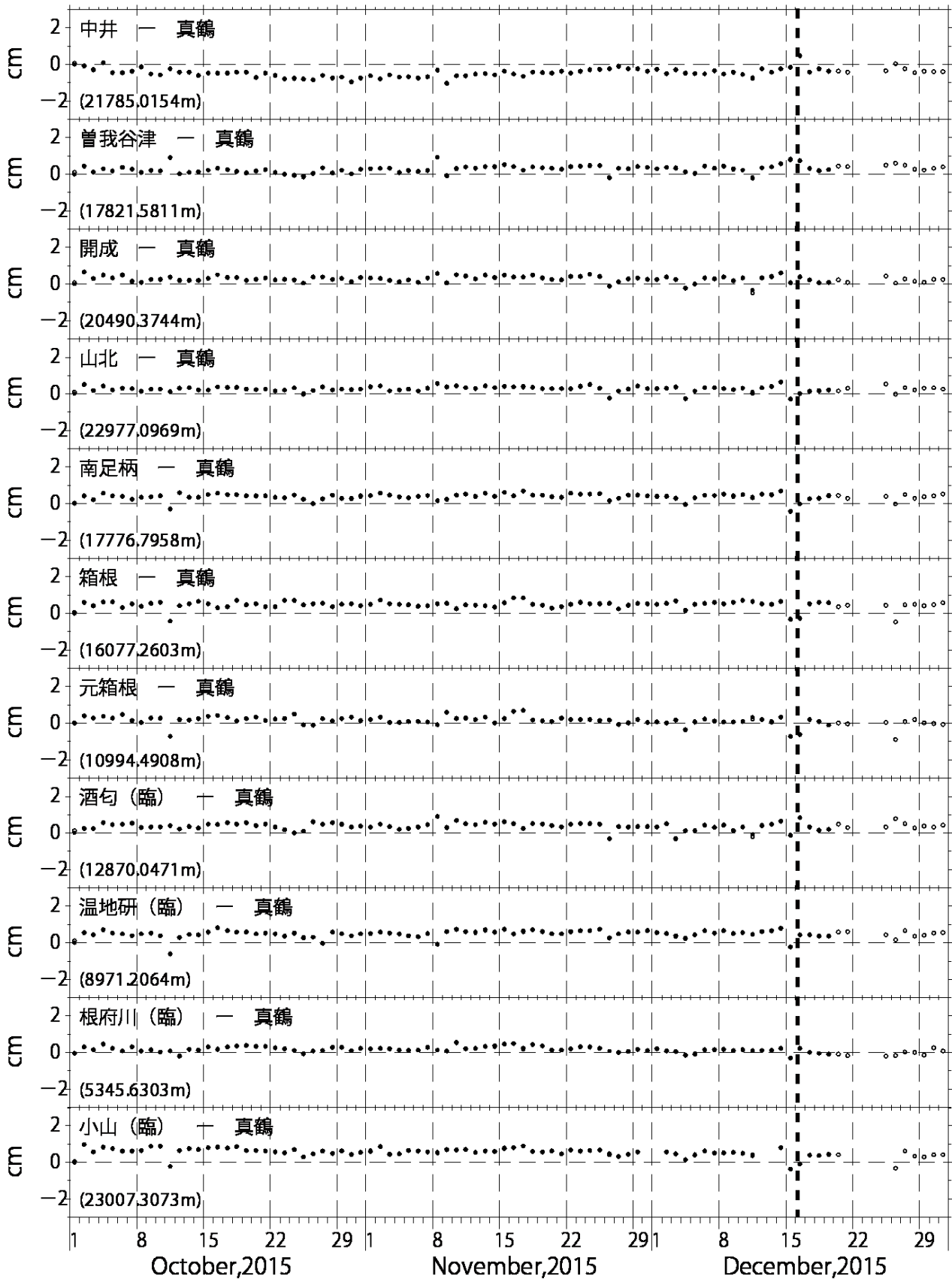
図4 GPS測量観測結果 (2015年10月01日~2015年12月31日)
