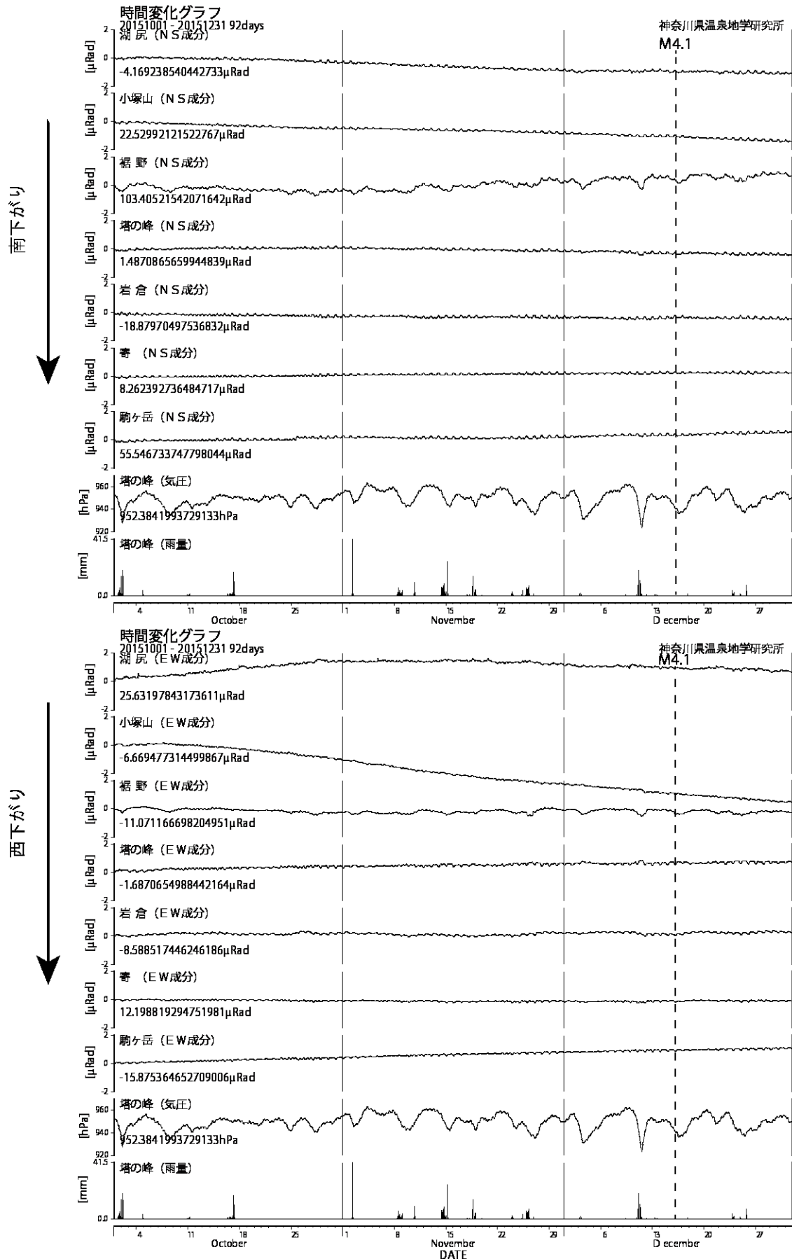
図3 傾斜計記録(2015年10月1日から2015年12月31日) 上:南北成分 下:東西成分
