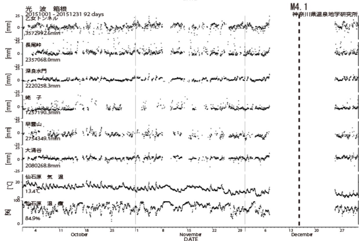
図5 光波測量観測結果 (2015年10月01日~2015年12月31日) 上: 小田原観測網、下: 箱根観測網
