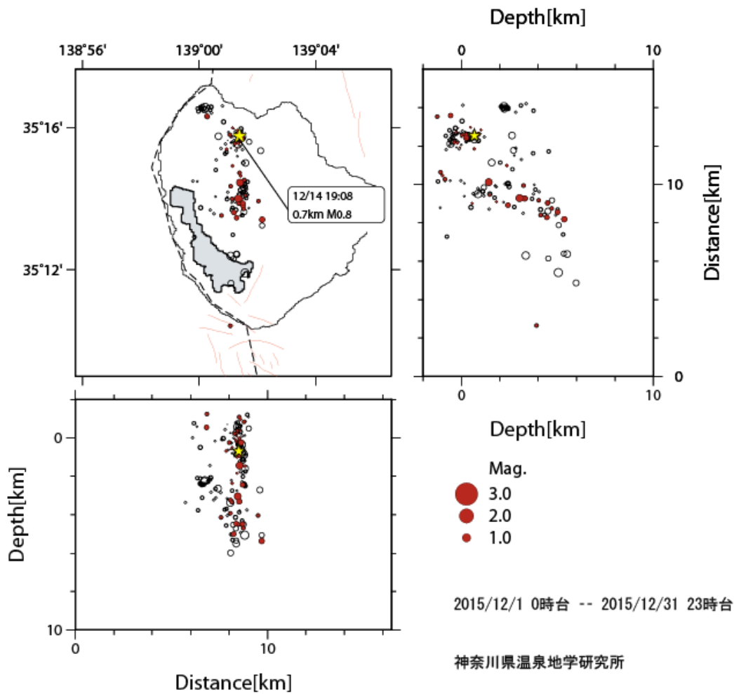
図 1-2 箱根火山の 12 月の地震活動（白丸は過去 3 ヶ月の震源、赤丸は今月の震源を示す。）
