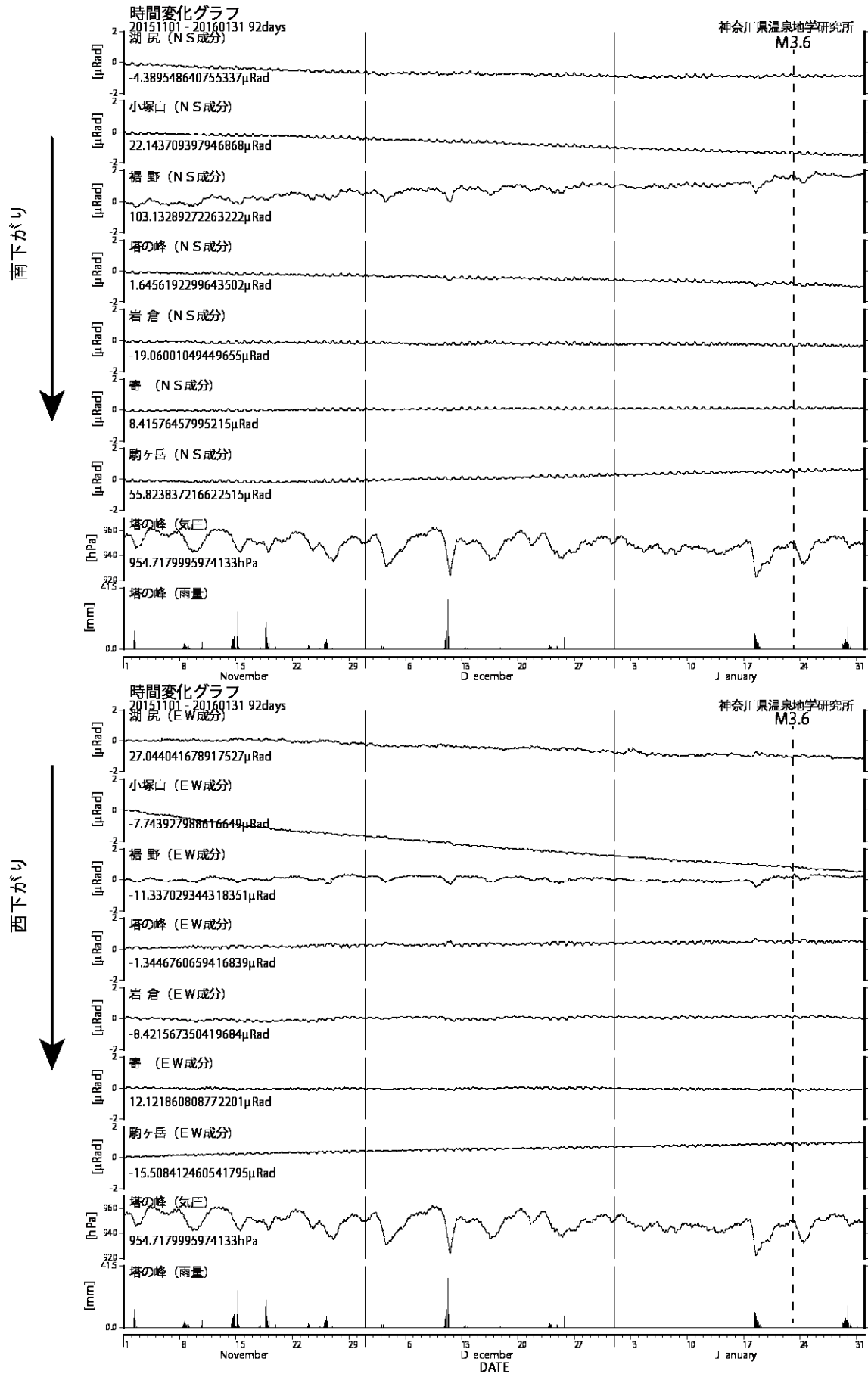
図3 傾斜計記録(2015年11月1日から2016年1月31日) 上:南北成分 下:東西成分
