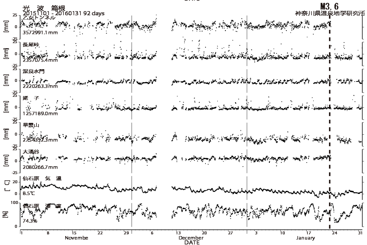
図5 光波測量観測結果 (2015年11月01日~2016年01月31日) 上: 小田原観測網、下: 箱根観測網
