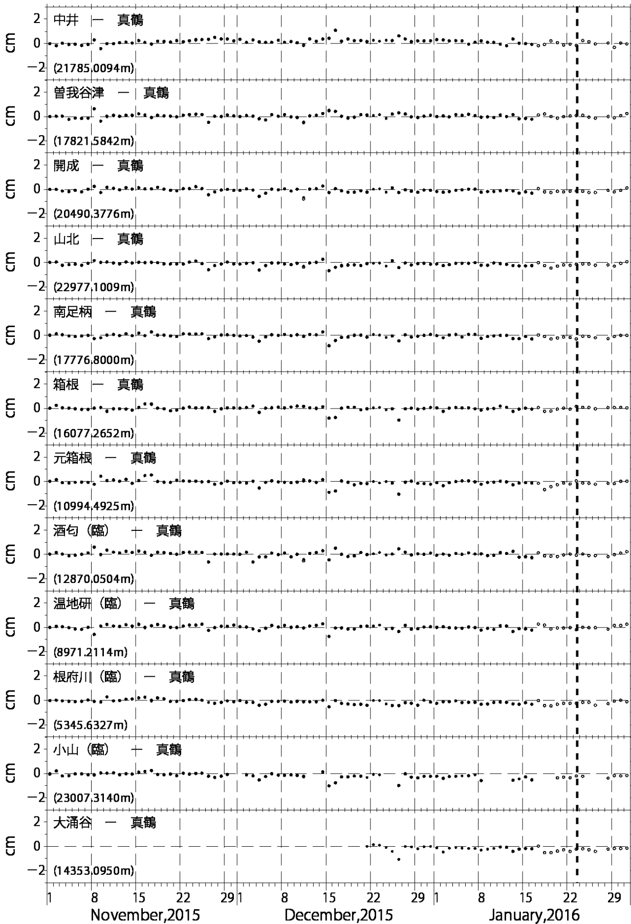
図4 GPS測量観測結果 (2015年11月01日~2016年01月31日)
