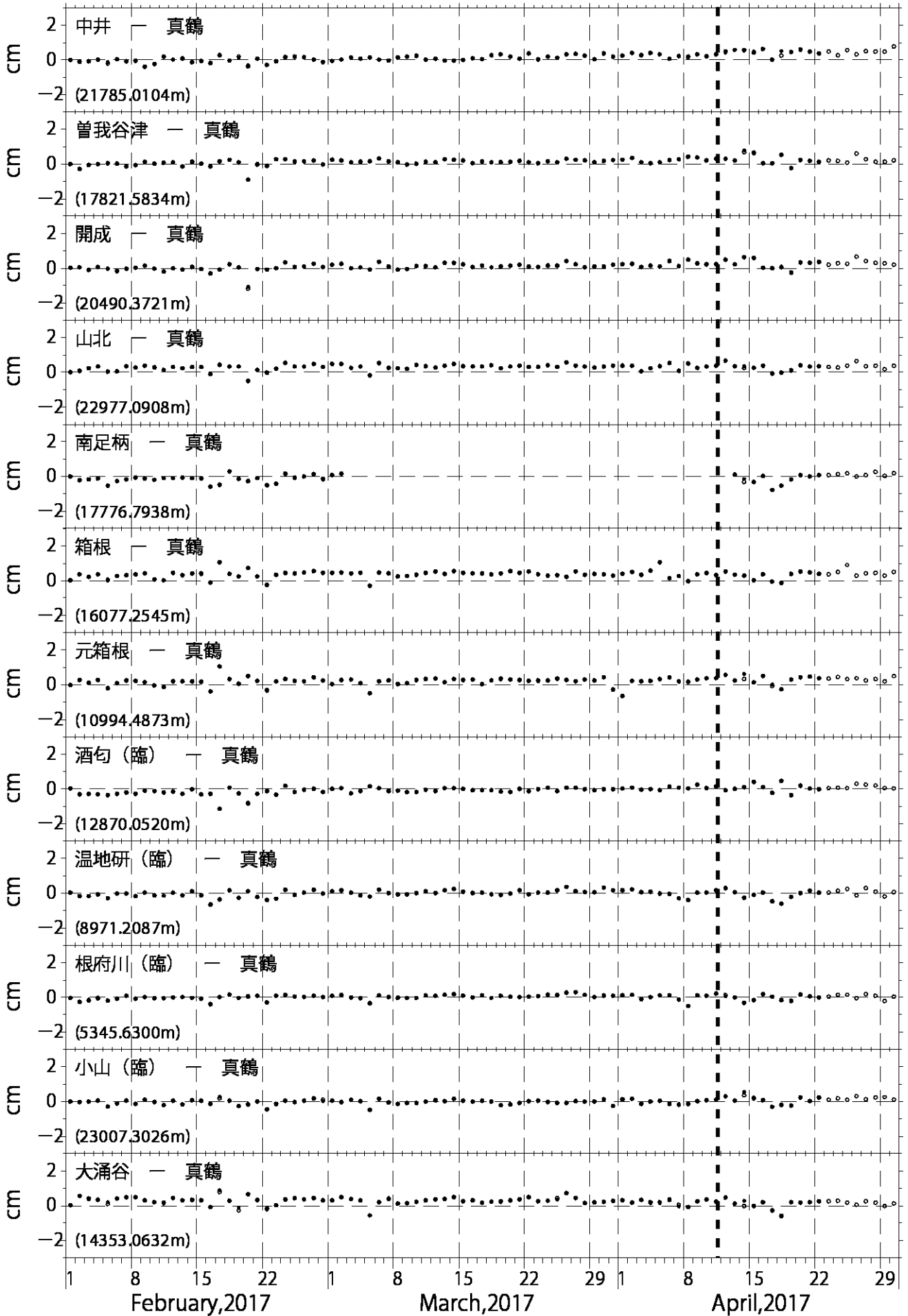
図4 GPS測量観測結果 (2017年02月01日~2017年04月30日) 真鶴観測点を中心とした、各観測点の基線長変化。●は精密暦、○は超速報暦による解を示す。
