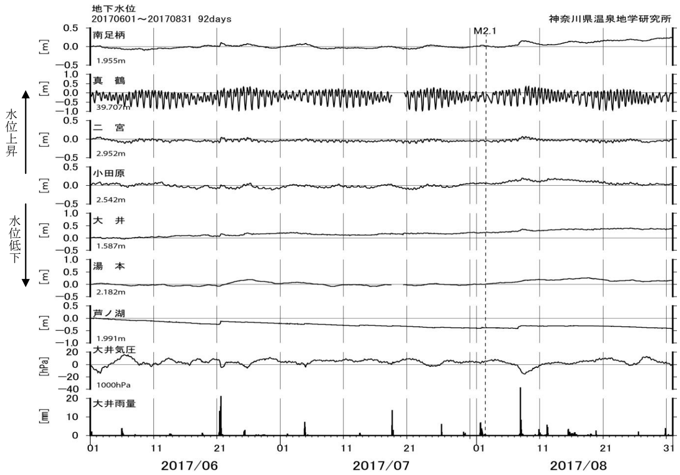
図6 地下水位観測結果(2017年6月~8月)
