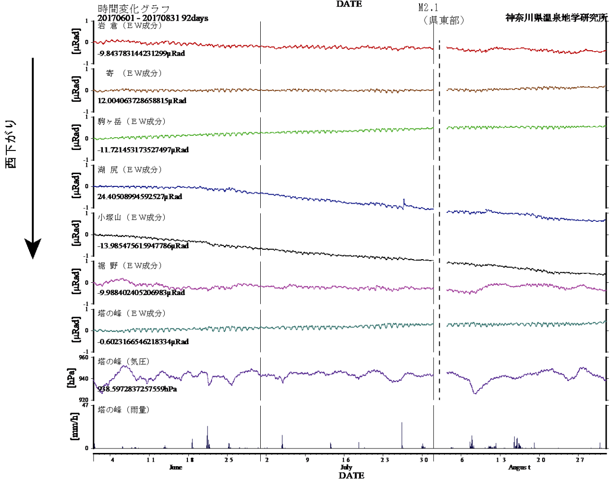
図3 傾斜計記録(2017年6月1日から2017年8月31日) 上:南北成分 下:東西成分
