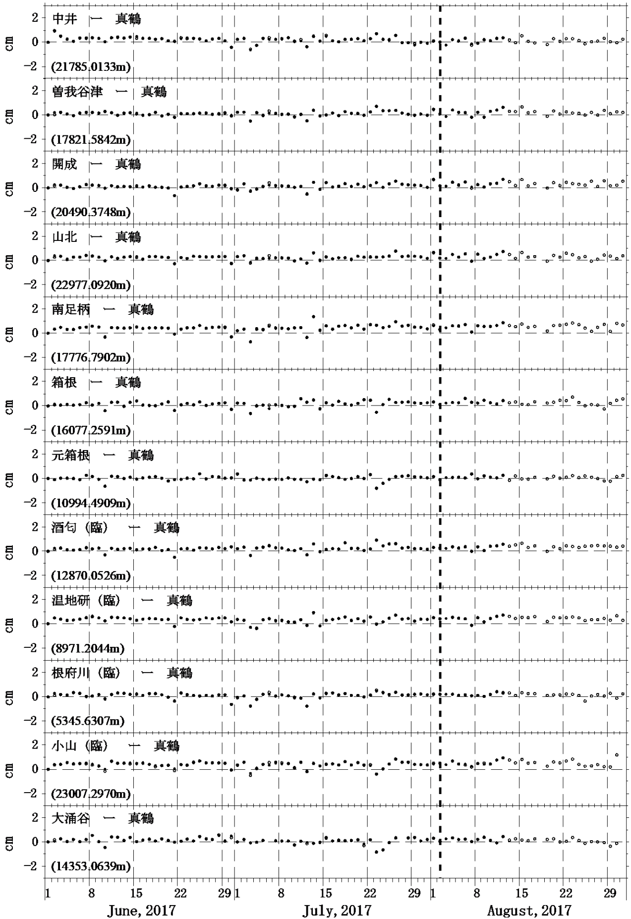
図4 GPS測量観測結果 (2017年06月01日~2017年08月31日) 真鶴観測点を中心とした、各観測点の基線長変化。●は精密暦、○は超速報暦による解を示す。
