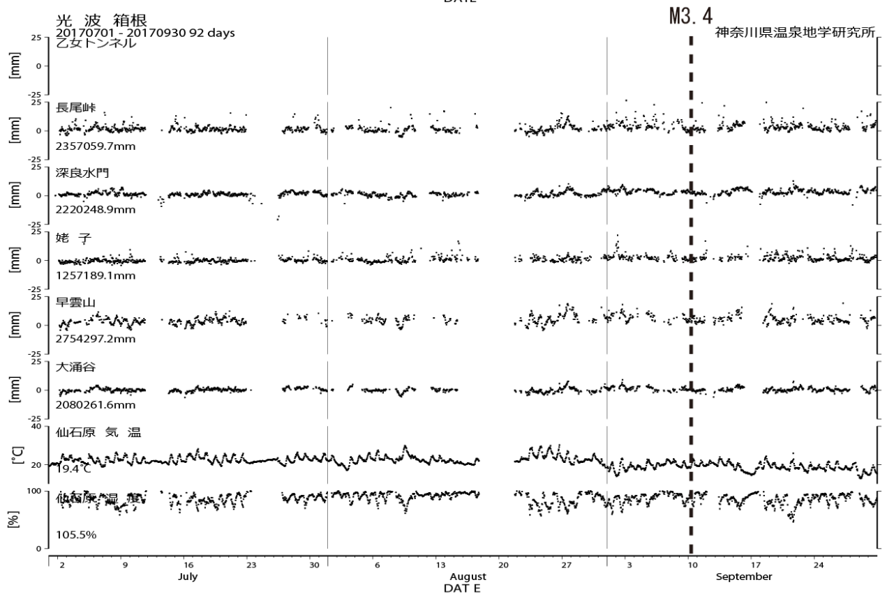
図5 光波測量観測結果 (2017年7月1日~2017年9月30日) 上: 小田原観測網、下: 箱根観測網
