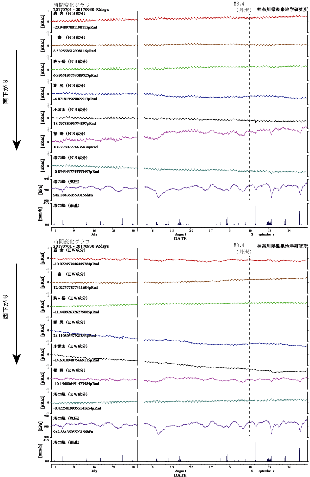
図3 傾斜計記録(2017年7月1日から2017年9月30日) 上:南北成分 下:東西成分
