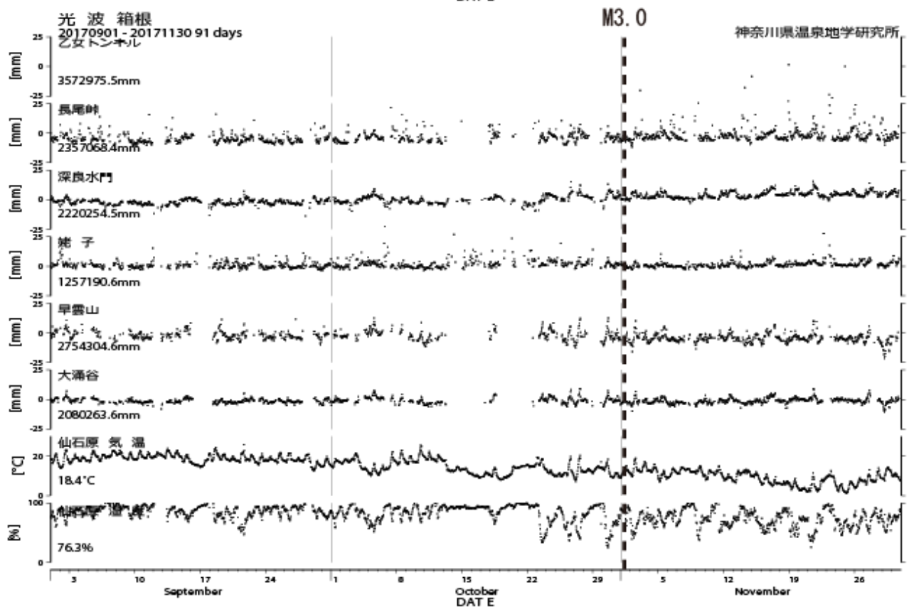
図5 光波測量観測結果 (2017年9月1日~2017年11月30日) 上: 小田原観測網、下: 箱根観測網
