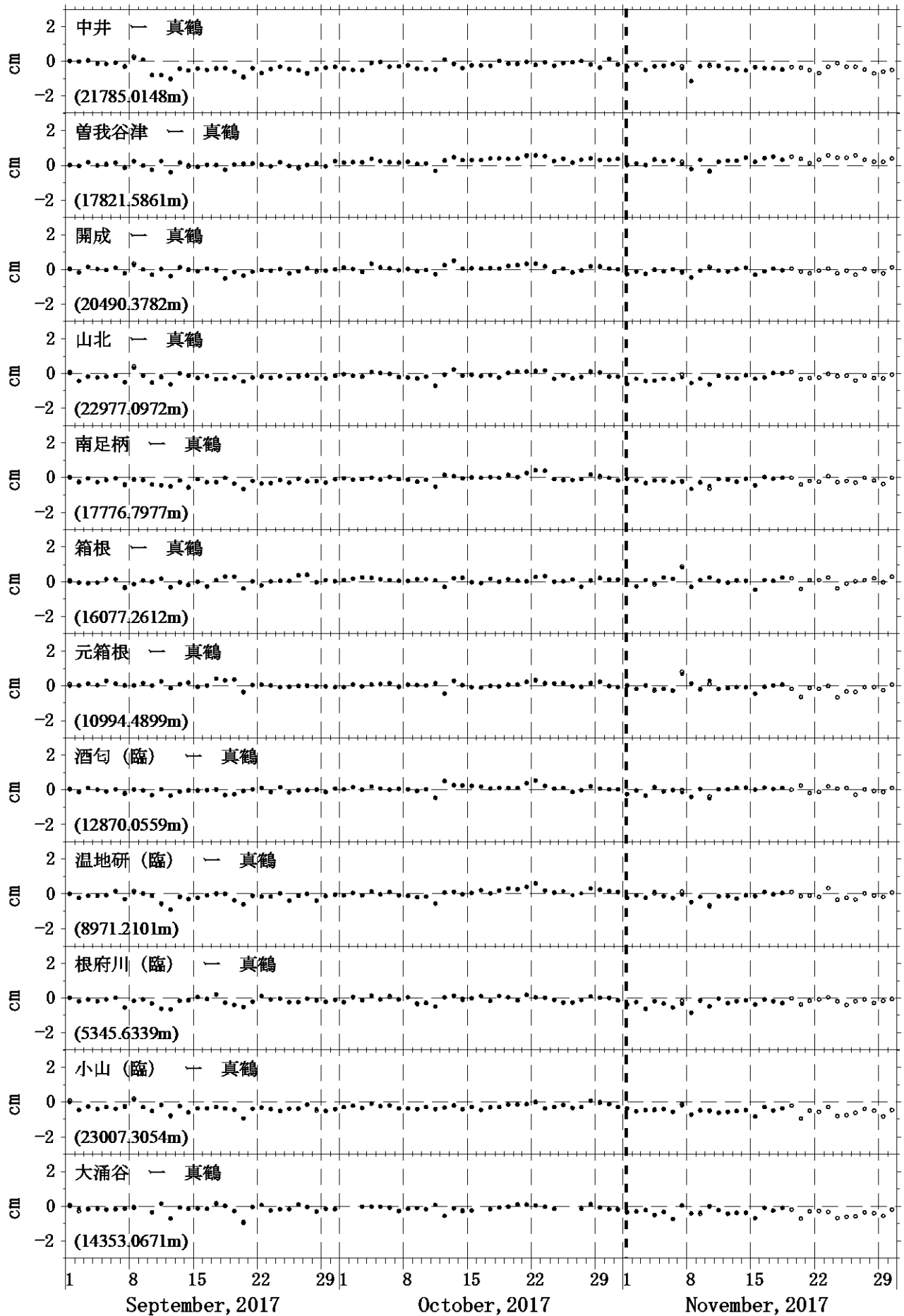
図4 GPS測量観測結果(2017年09月01日~2017年11月30日) 真鶴観測点を中心とした、各観測点の基線長変化。●は精密層、○は超速報層による解を示す。
