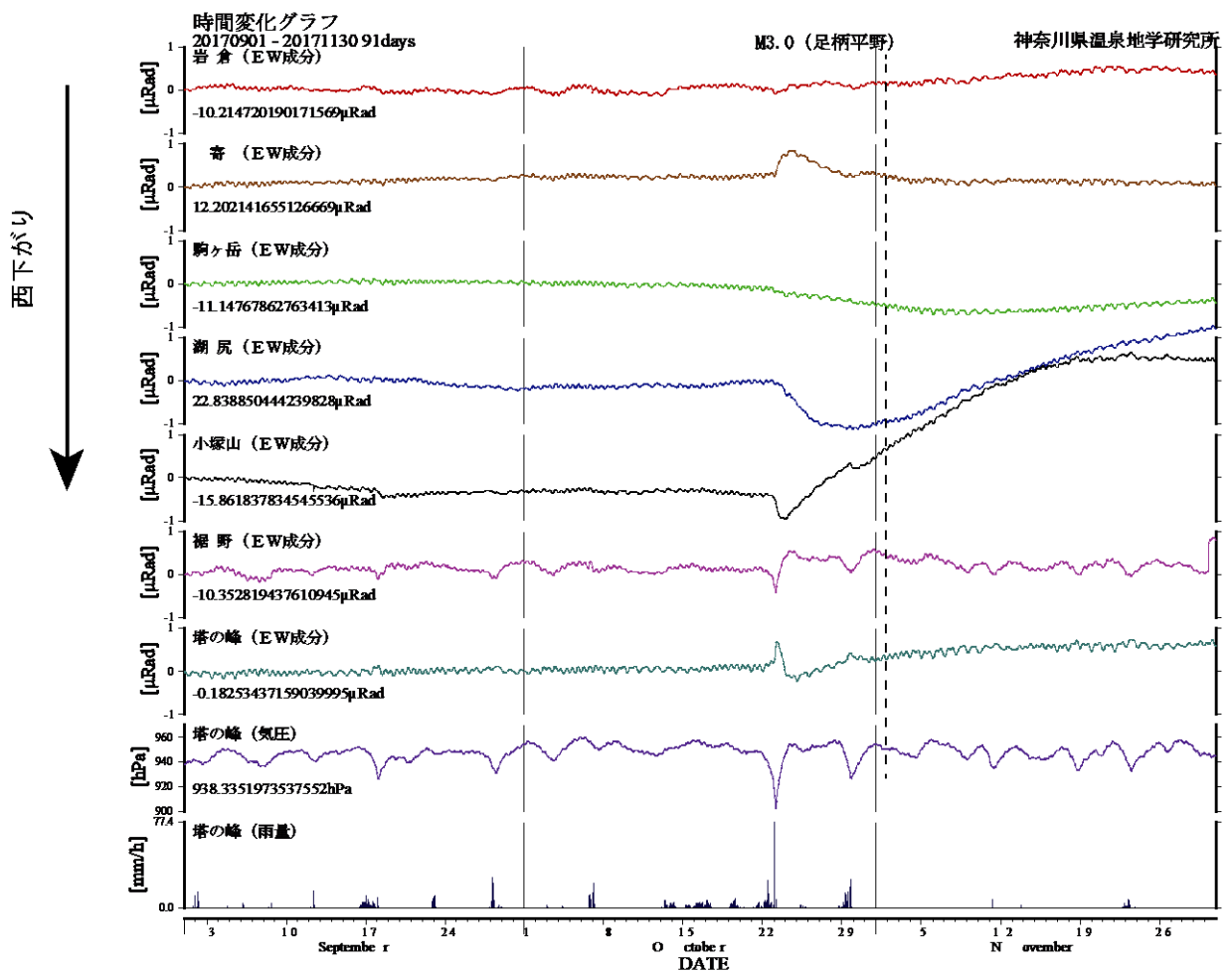
図3 傾斜計記録(2017年9月01日から2017年11月30日) 上:南北成分 下:東西成分
