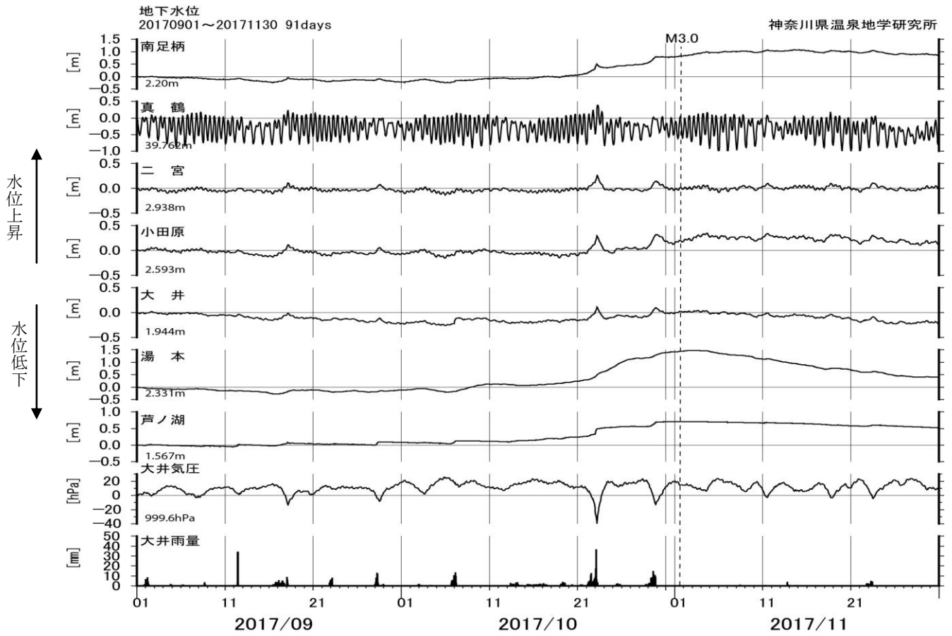
図6 地下水位観測結果(2017年9月~11月)
