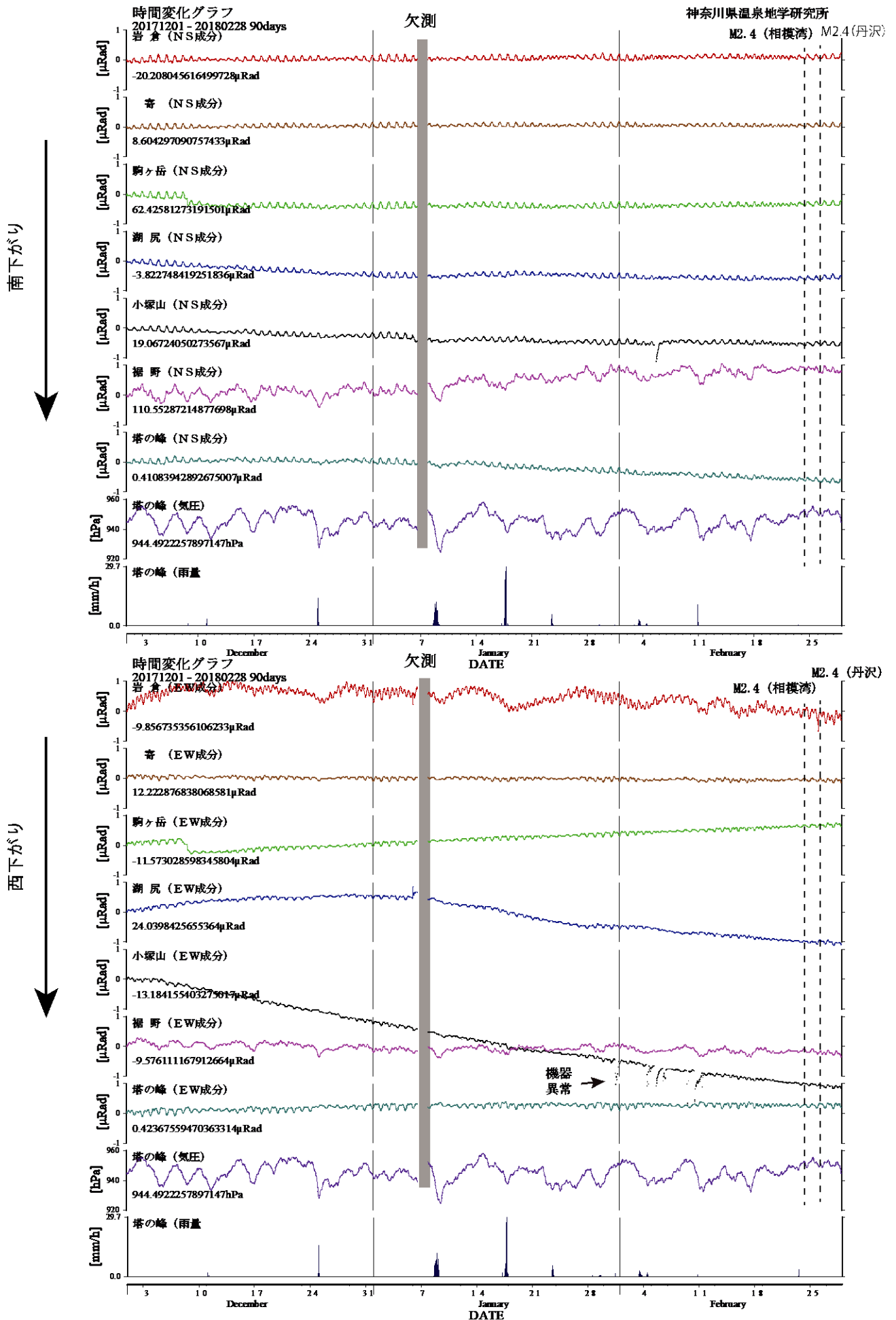
図3 傾斜計記録(2017年12月01日から2018年2月28日) 上:南北成分 下:東西成分
