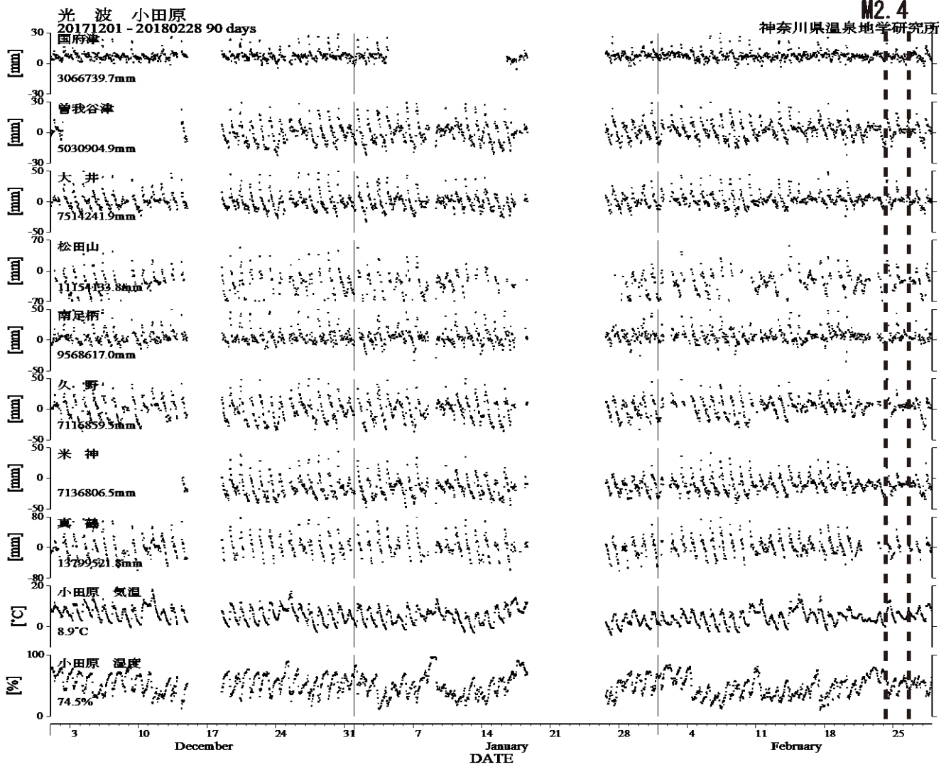
図5 光波測量（小田原観測網）観測結果（2017年12月01日～2018年02月28日）
