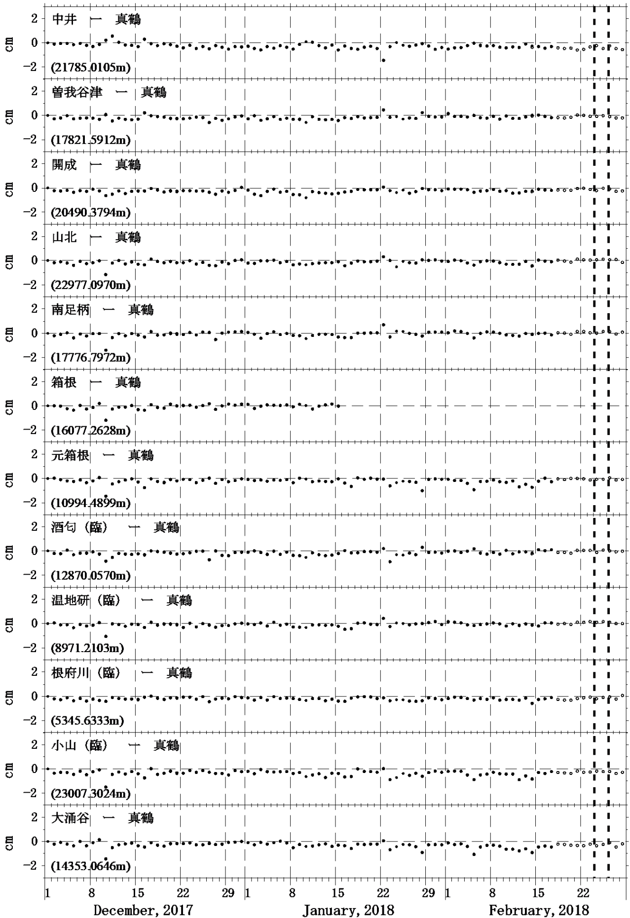
図4 GPS測量観測結果（2017年12月01日～2018年02月28日） 真鶴観測点を中心とした、各観測点の基線長変化。●は精密層、○は超速報層による解を示す。
