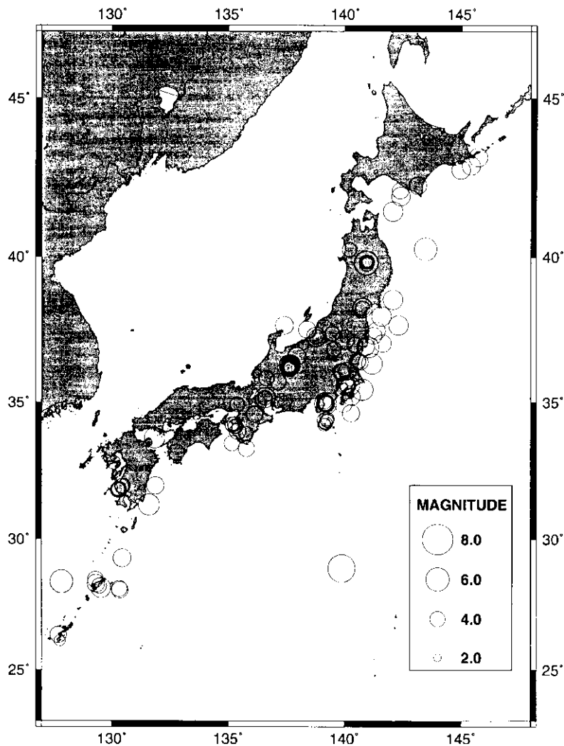
図1 震源分布図 (平成10年1月1日~12月31日)
