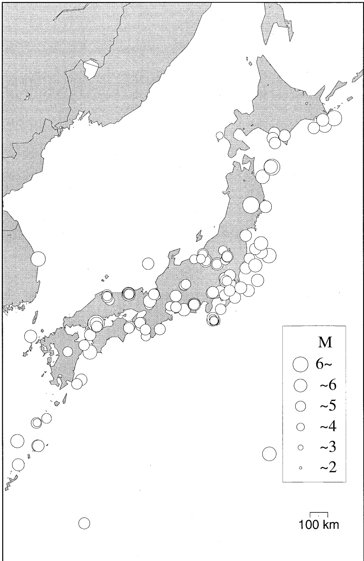
図1 震源分布(平成13年1月1日~12月31日)
