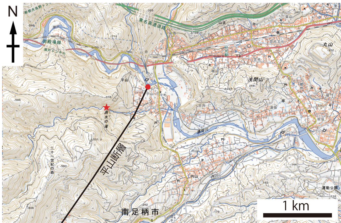
図 1 洒水の滝周辺の地形図。★印は洒水の滝、●印は平山断層露頭の位置。地理院地図 ( https://maps.gsi.go.jp/ ) に加筆。
