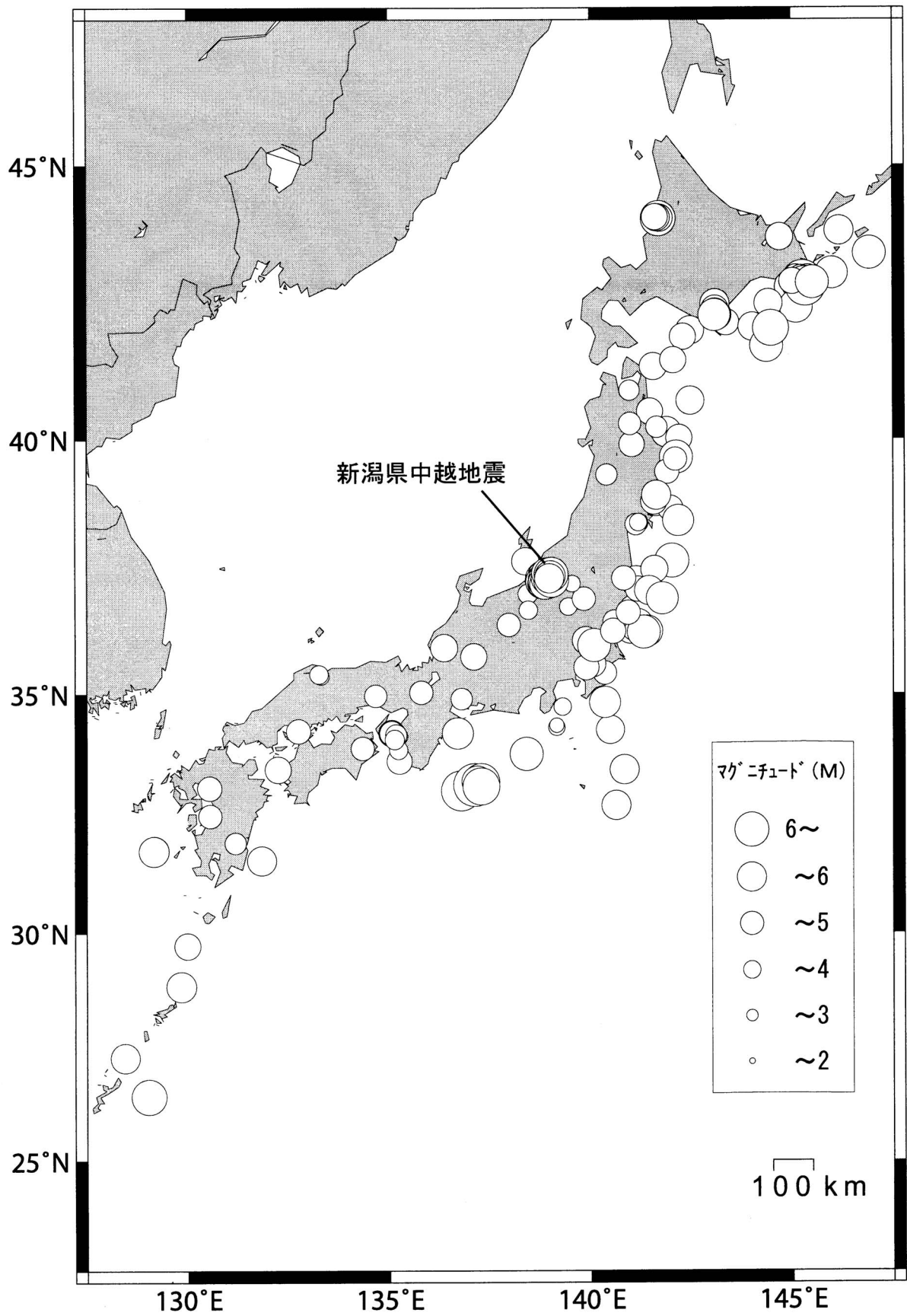
図1 震源分布(平成16年1月1日~12月31日)
