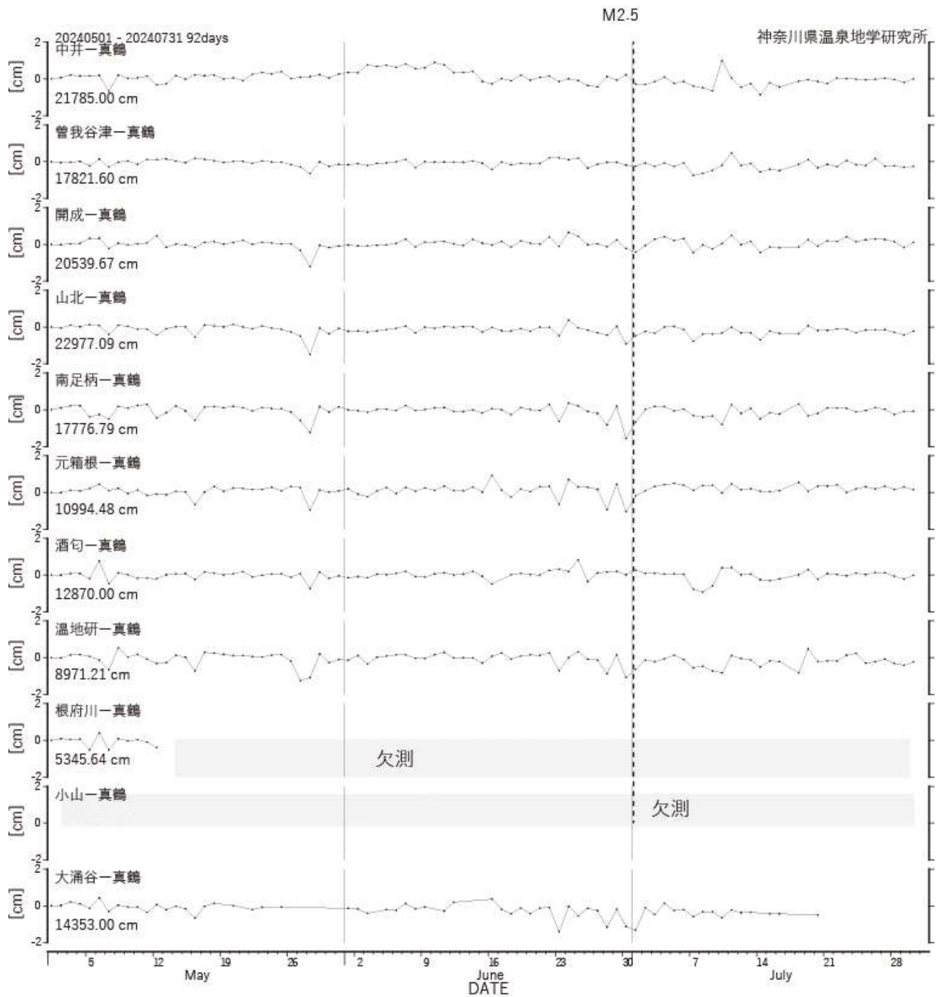
図4 GNSS測量観測結果(2024年05月01日～2024年07月31日) 真鶴観測点を基準とした、各観測点の基線長変化。 根府川・小山は通信に不具合のため一部欠測。
