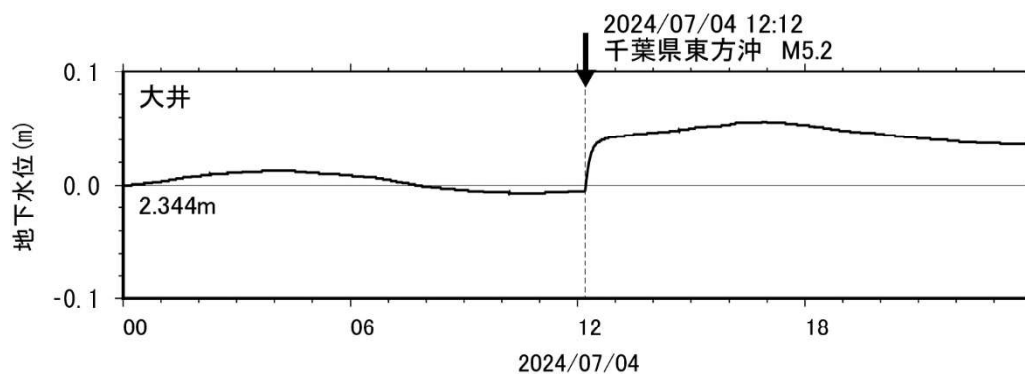
図 6 - 2 コサイスミックな地下水位の変化 (2024年07月04日)
