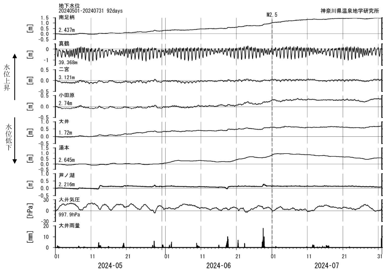
図 6 - 1 地下水位観測結果 (2024年05月01日～2024年07月31日)
