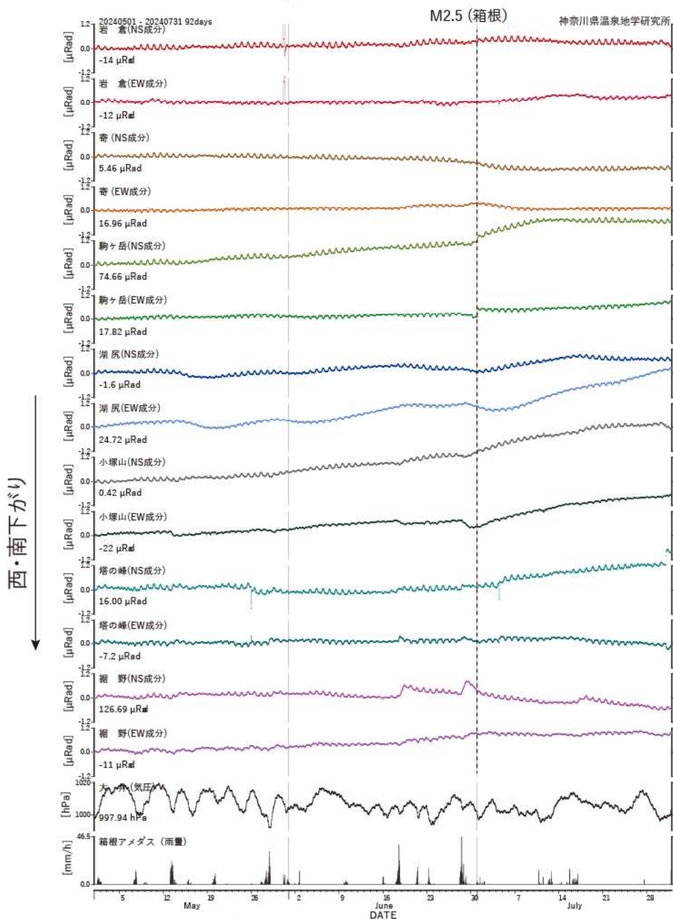
図 3 傾斜計記録 (2024年05月01日から2024年07月31日)
