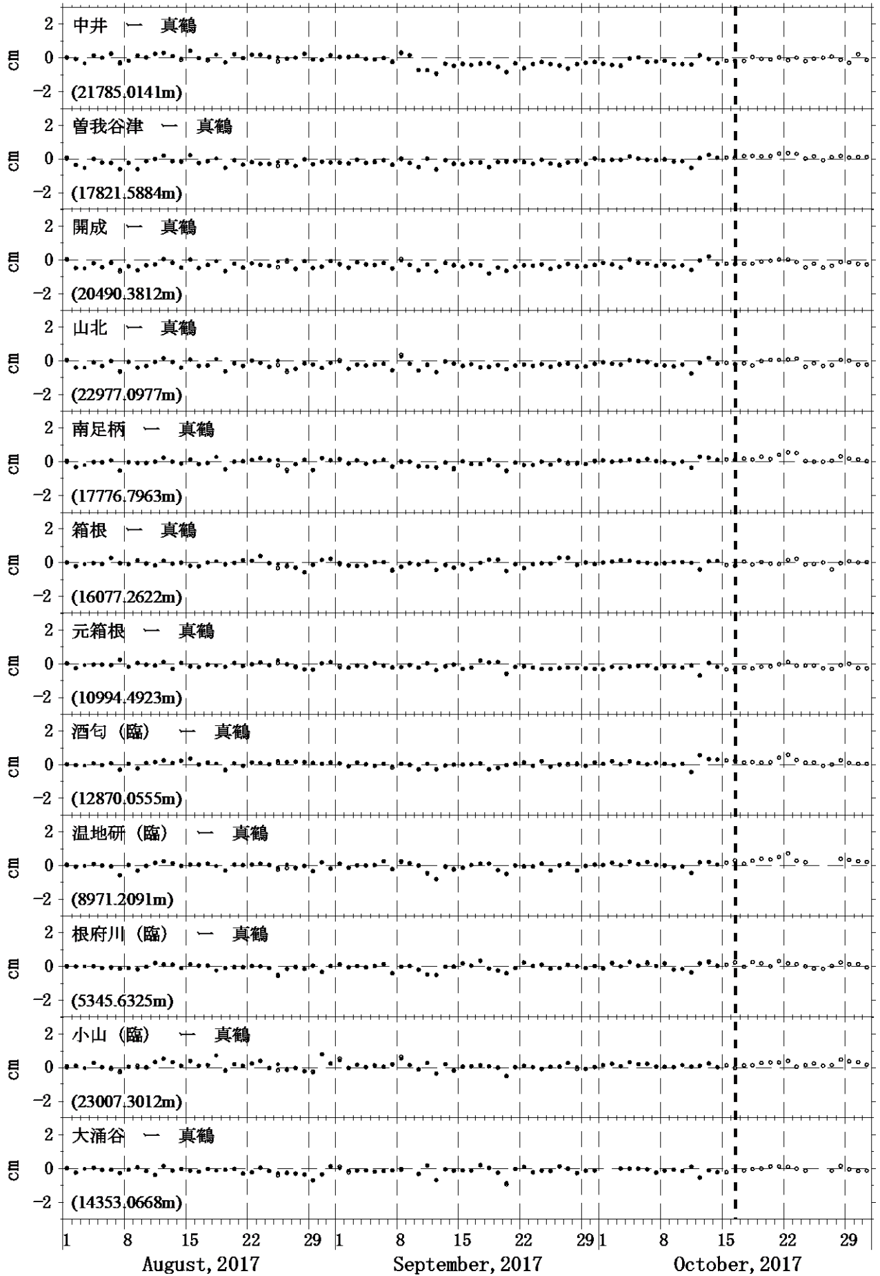
図4 GPS測量観測結果 (2017年08月01日~2017年10月31日) 真鶴観測点を中心とした、各観測点の基線長変化。●は精密暦、○は超速報暦による解を示す。
