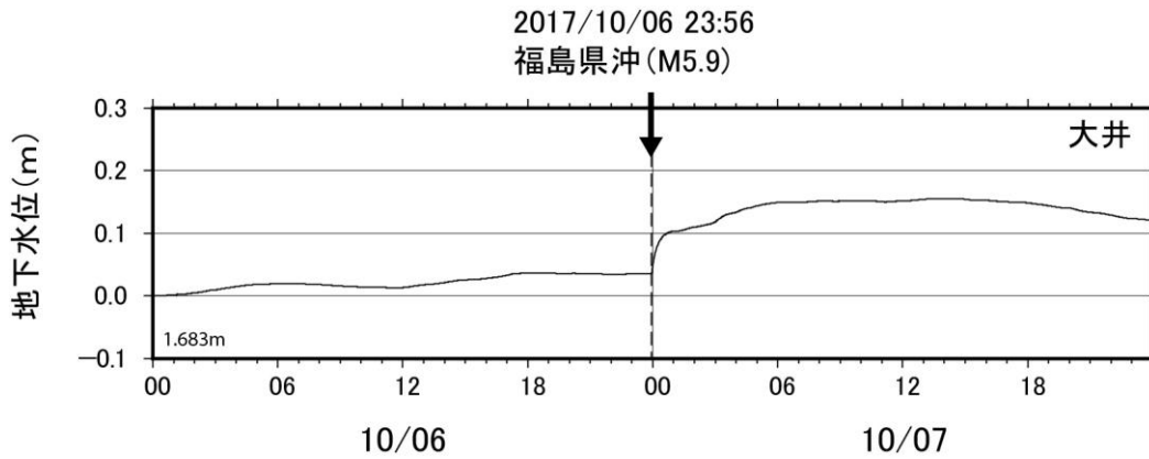
図6-2 地震の影響とみられる水位変化(2017年10月6日)
