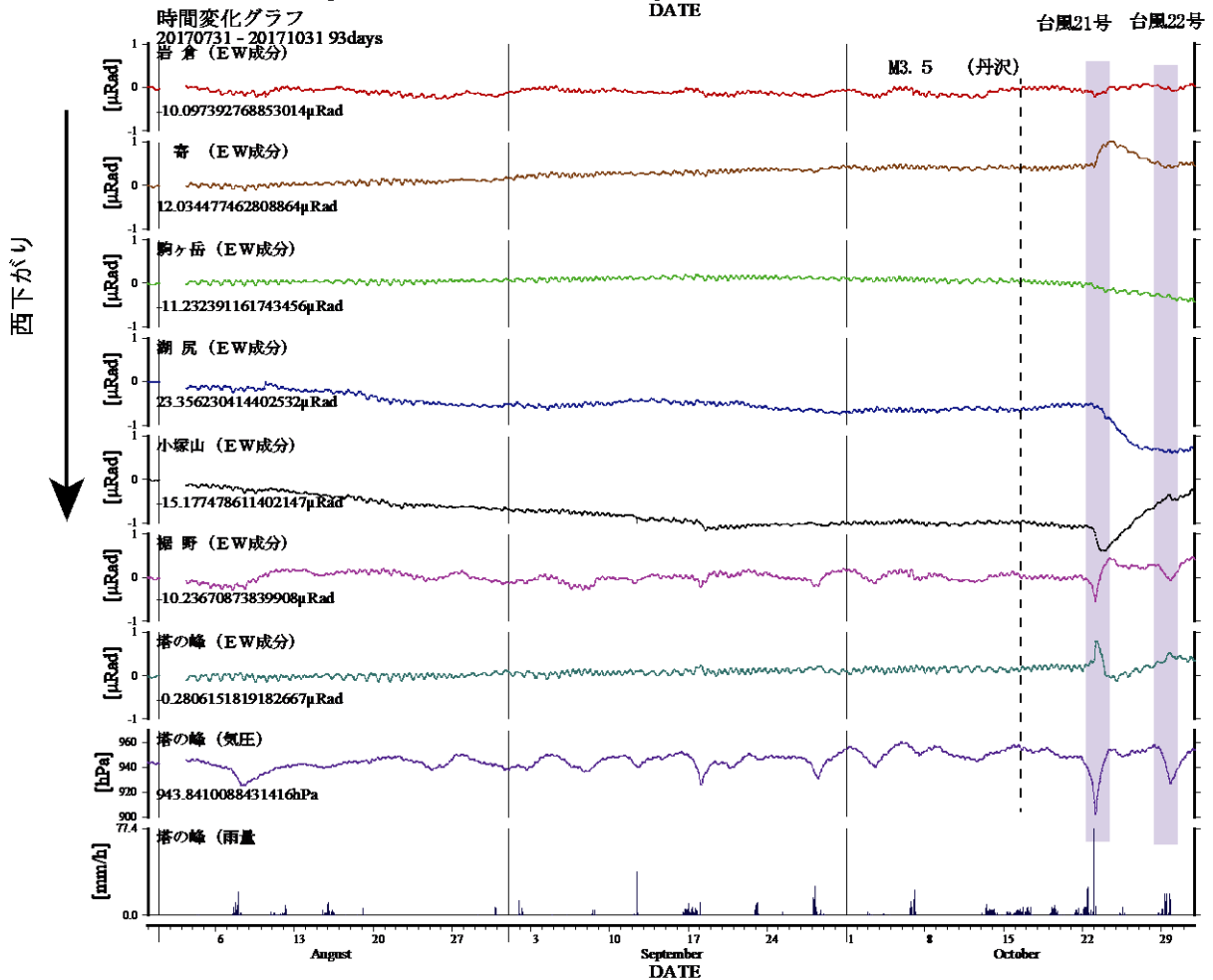
図3 傾斜計記録(2017年7月31日から2017年10月31日) 上:南北成分 下:東西成分
