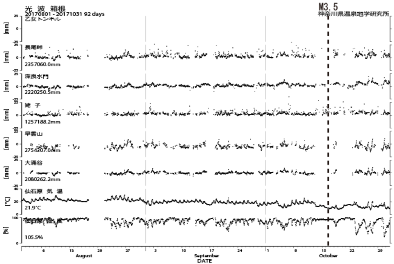
図5 光波測量観測結果 (2017年8月1日~2017年10月31日) 上: 小田原観測網、下: 箱根観測網
