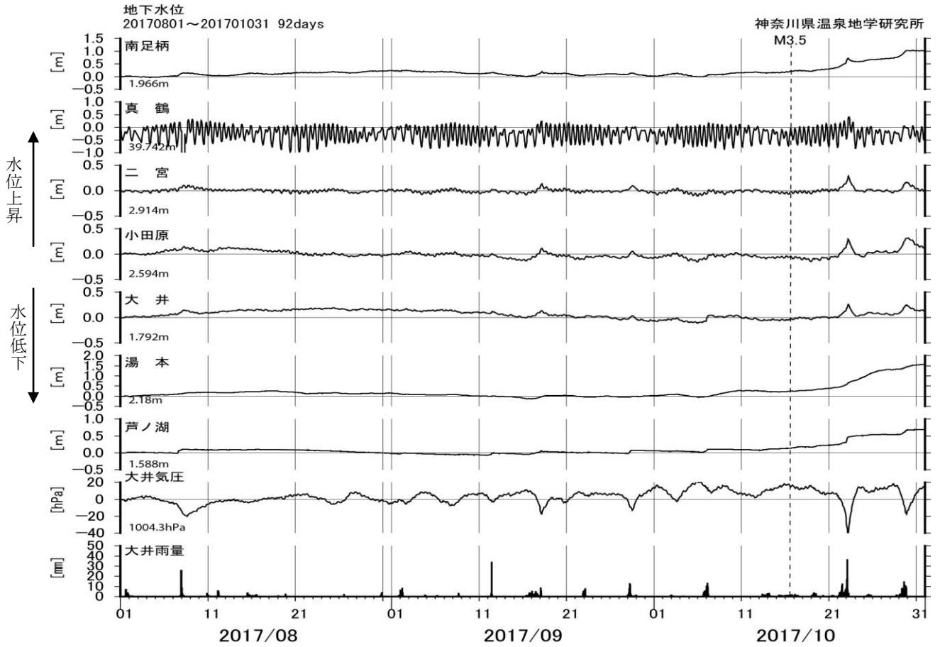
図6-1 地下水位観測結果(2017年8月~10月)
