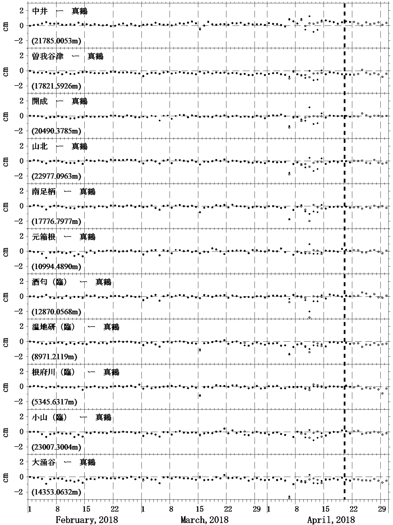
図4 GPS測量観測結果 (2018年02月01日~2018年04月30日) 真鶴観測点を中心とした、各観測点の基線長変化。●は精密暦、○は超速報暦による解を示す。
