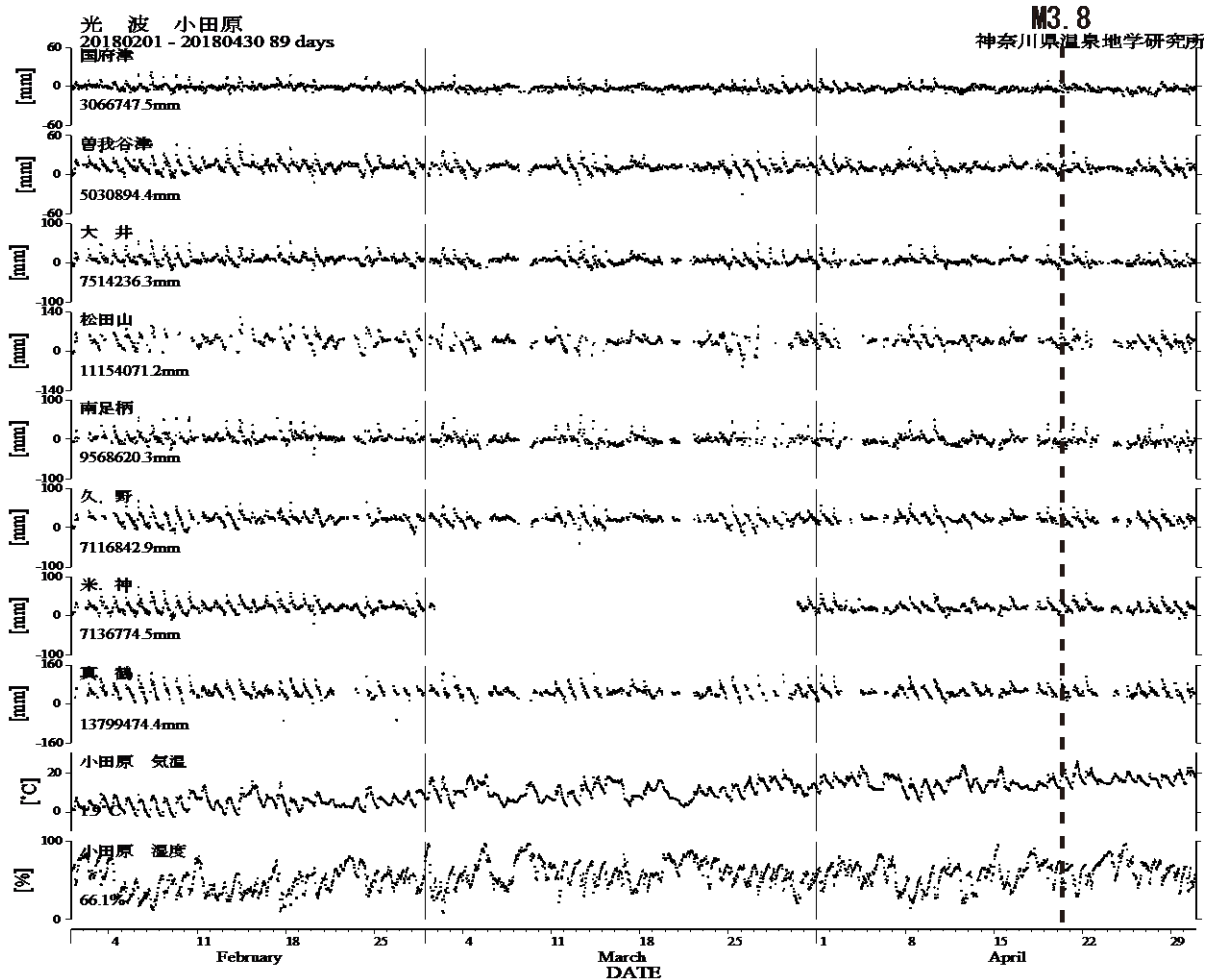
図5 光波測量（小田原観測網）観測結果（2018年02月01日～2018年04月30日）
