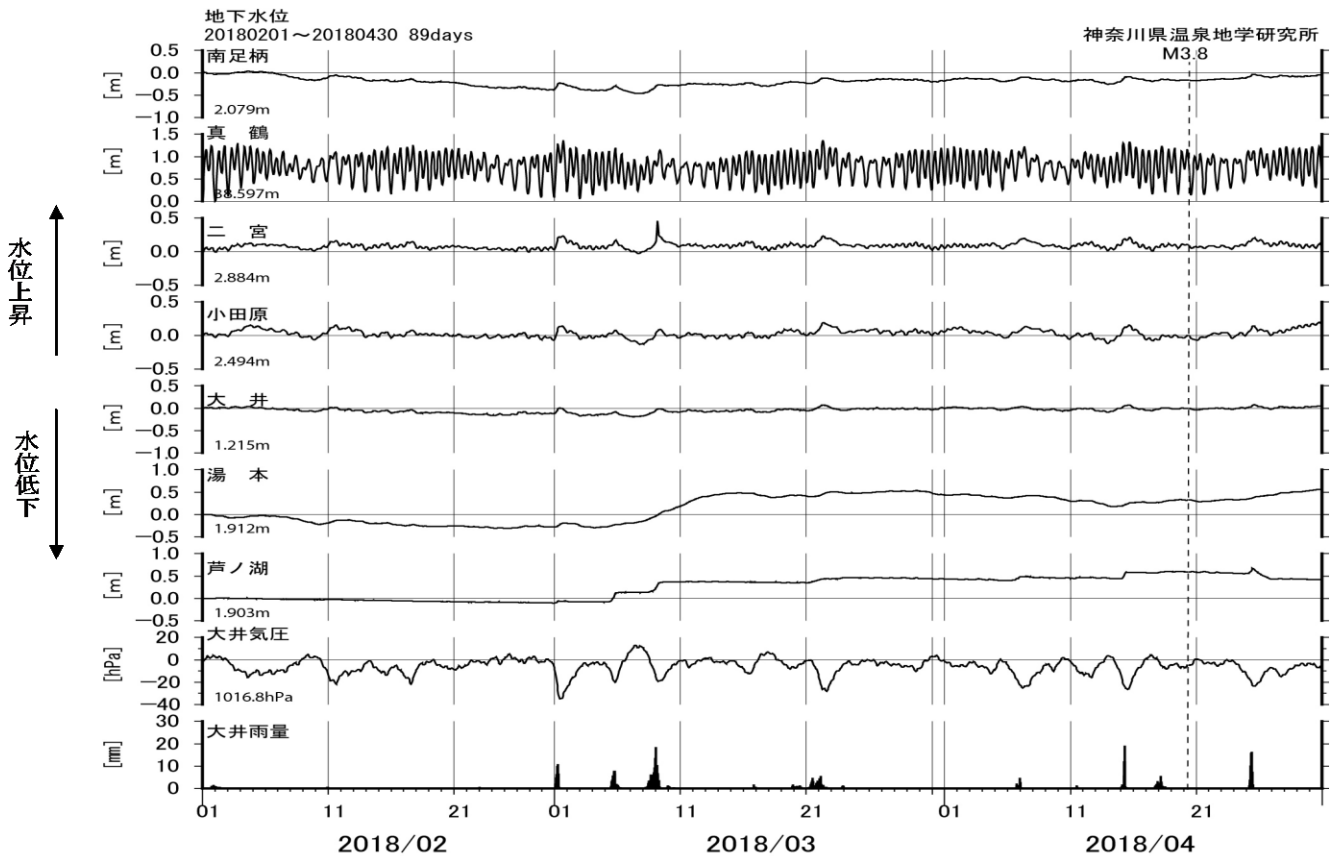
図6 地下水位観測結果(2018年02月01日～04月30日)
