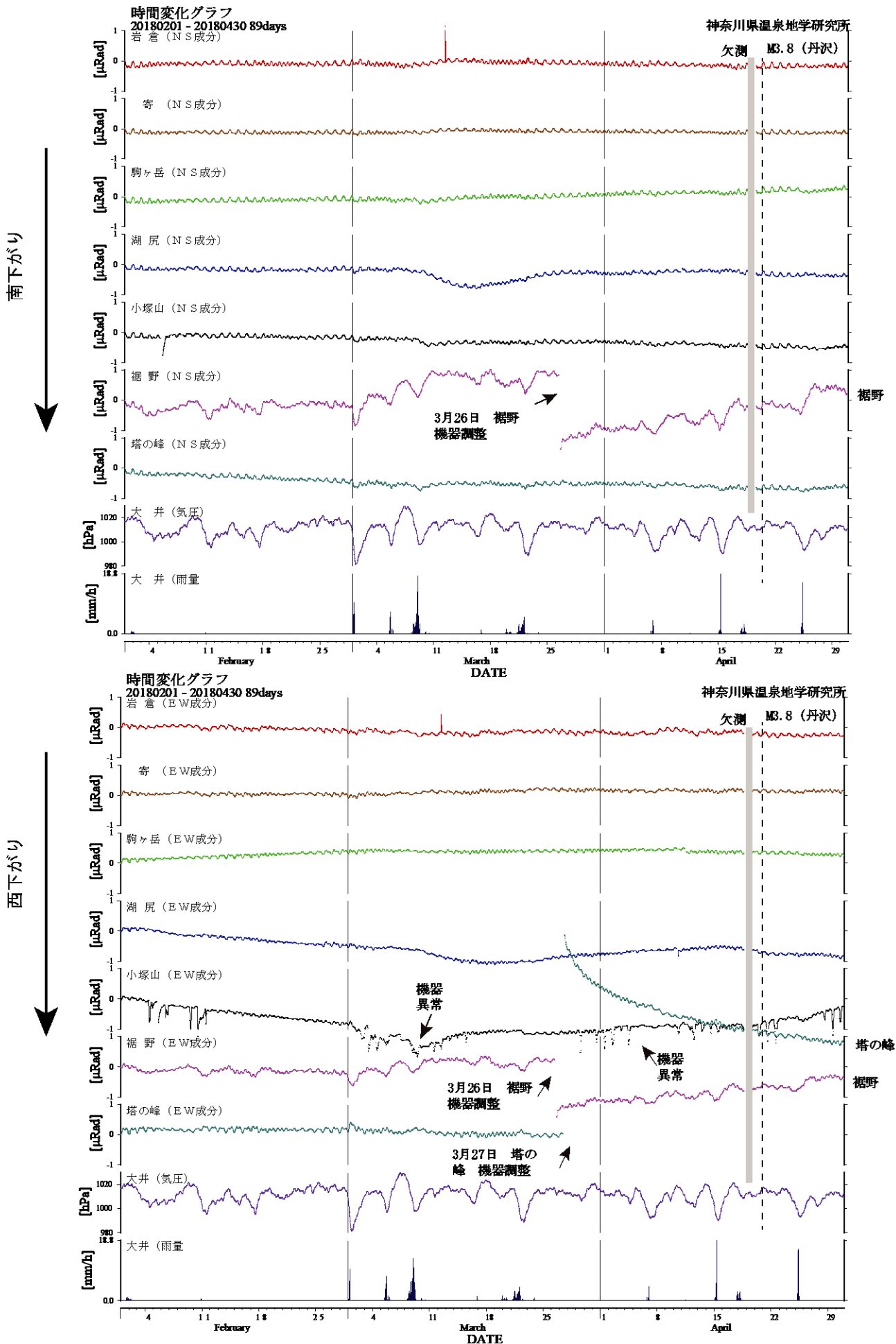
図3 傾斜計記録(2018年2月1日から2018年4月30日) 上:南北成分 下:東西成分
