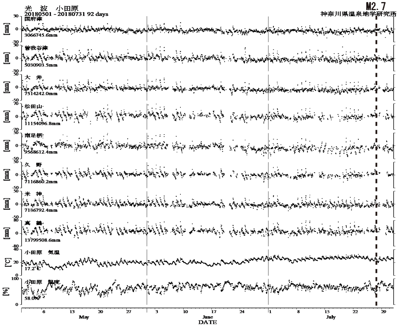
図5 光波測量 (小田原観測網) 観測結果 (2018年05月01日~2018年07月31日)
