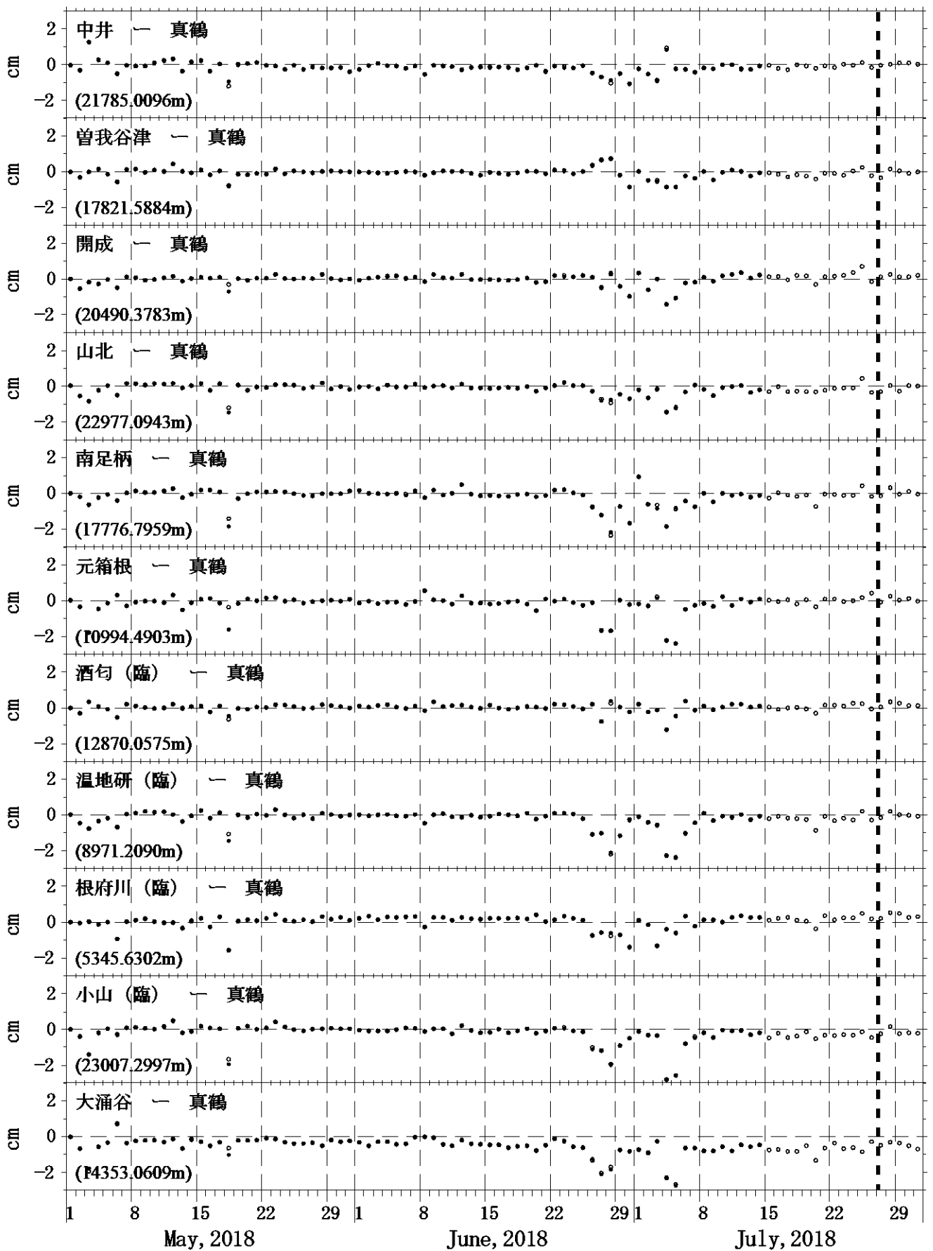
図4 GPS測量観測結果（2018年05月01日～2018年07月31日） 真鶴観測点を中心とした、各観測点の基線長変化。●は精密暦、○は超速報暦による解を示す。
