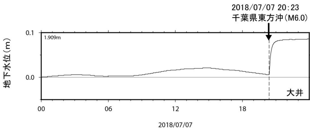
図6-2 地震の影響とみられる水位変化(7月7日)
