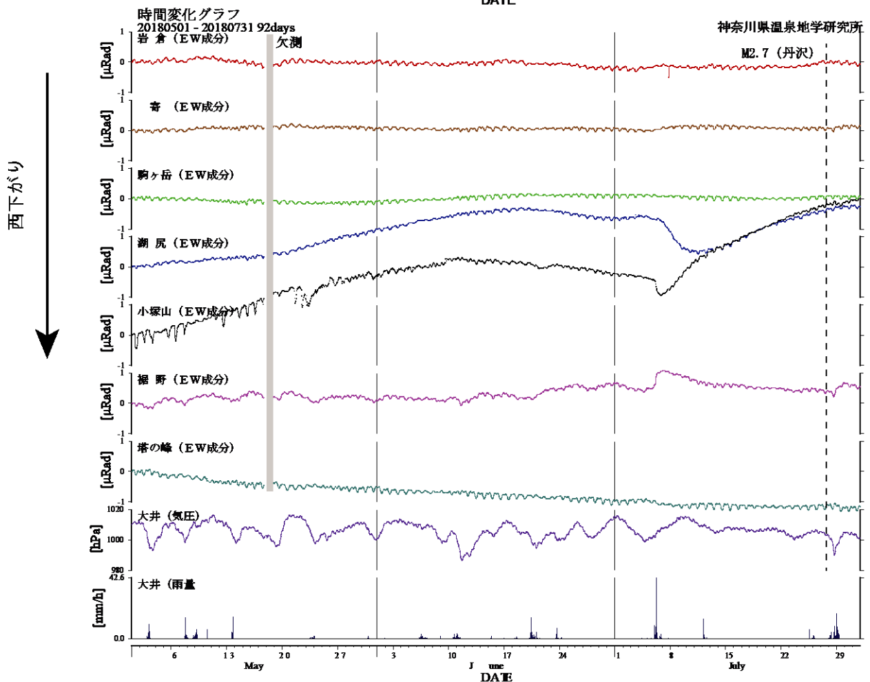
図3 傾斜計記録(2018年5月1日から2018年7月31日) 上:南北成分 下:東西成分
