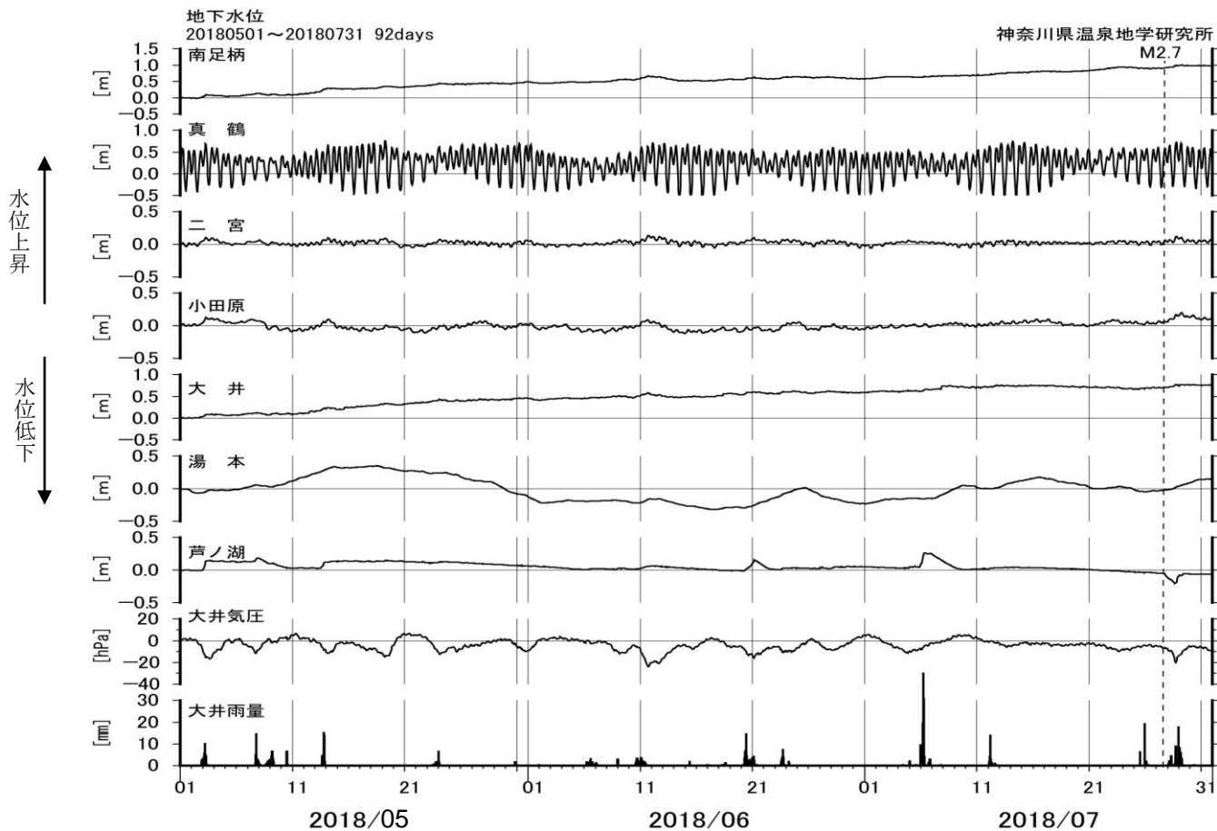
図6-1 地下水位観測結果(2018年5月~7月)
