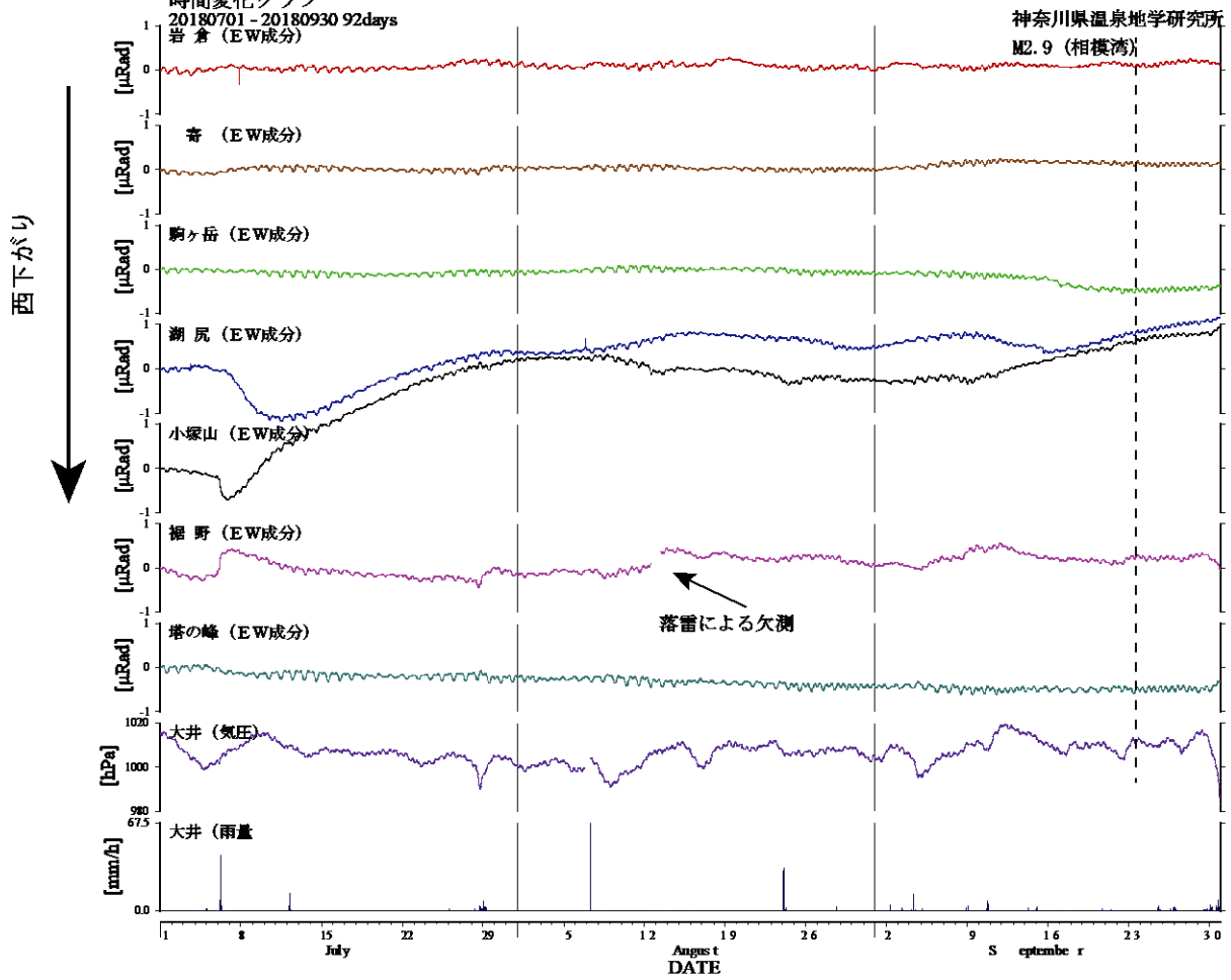
図3 傾斜計記録(2018年07月01日から2018年09月30日) 上:南北成分 下:東西成分
