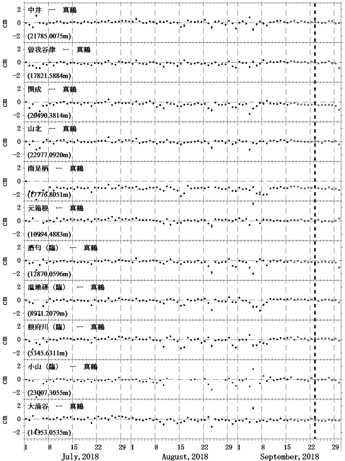
図4 GPS測量観測結果 (2018年07月01日~2018年09月30日) 真鶴観測点を中心とした、各観測点の基線長変化。●は精密暦、○は超速報暦による解を示す。
