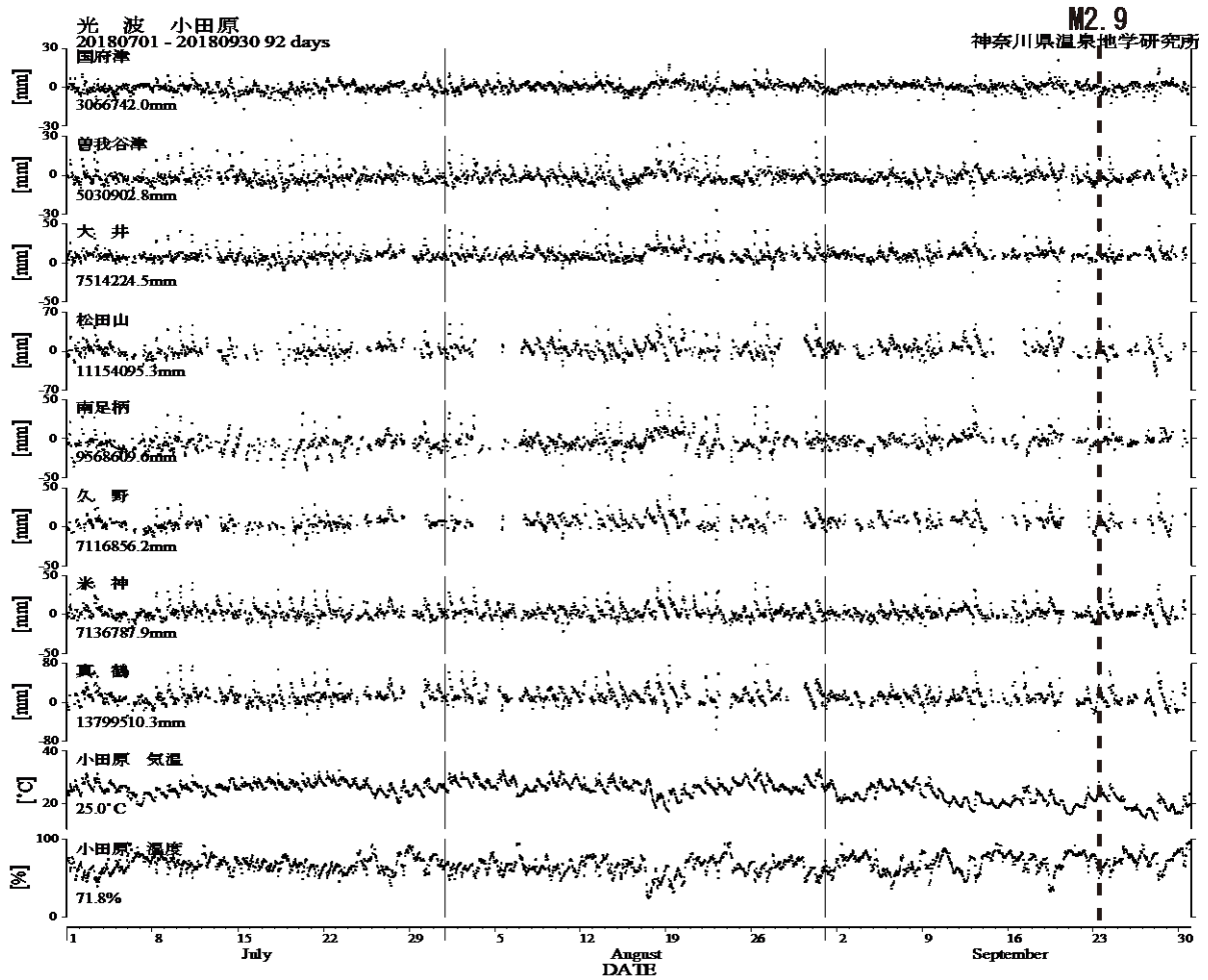
図5 光波測量（小田原観測網）観測結果（2018年07月01日～2018年09月30日）
