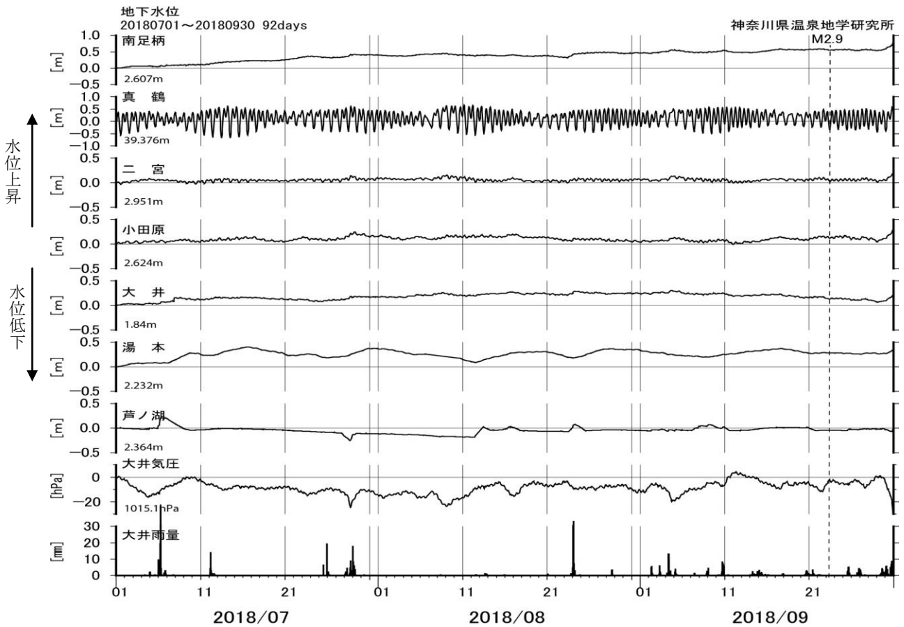
図6 地下水位観測結果（2018年07月01日～09月30日）
