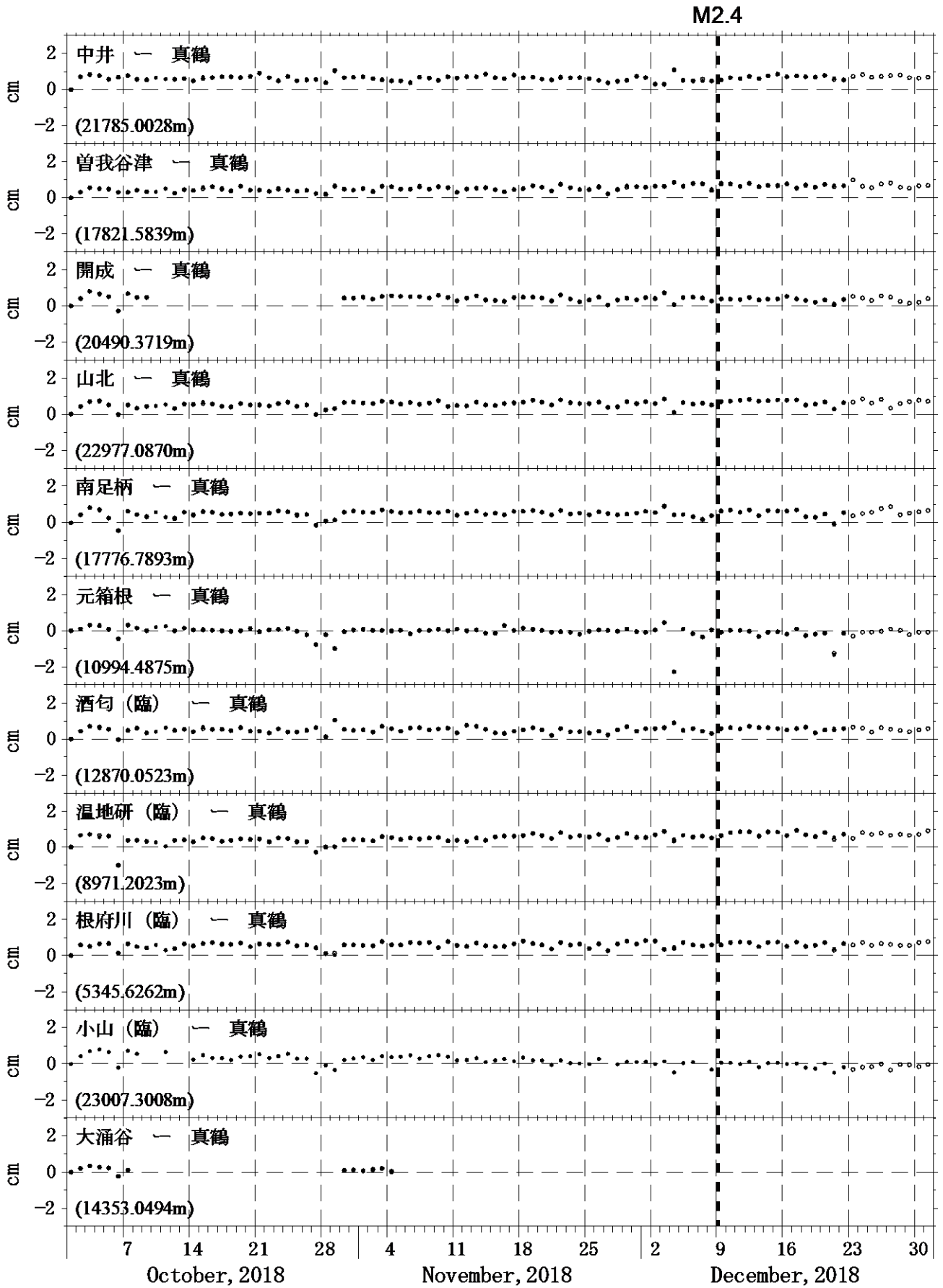
図4 GPS測量観測結果 (2018年10月01日~2018年12月31日)
