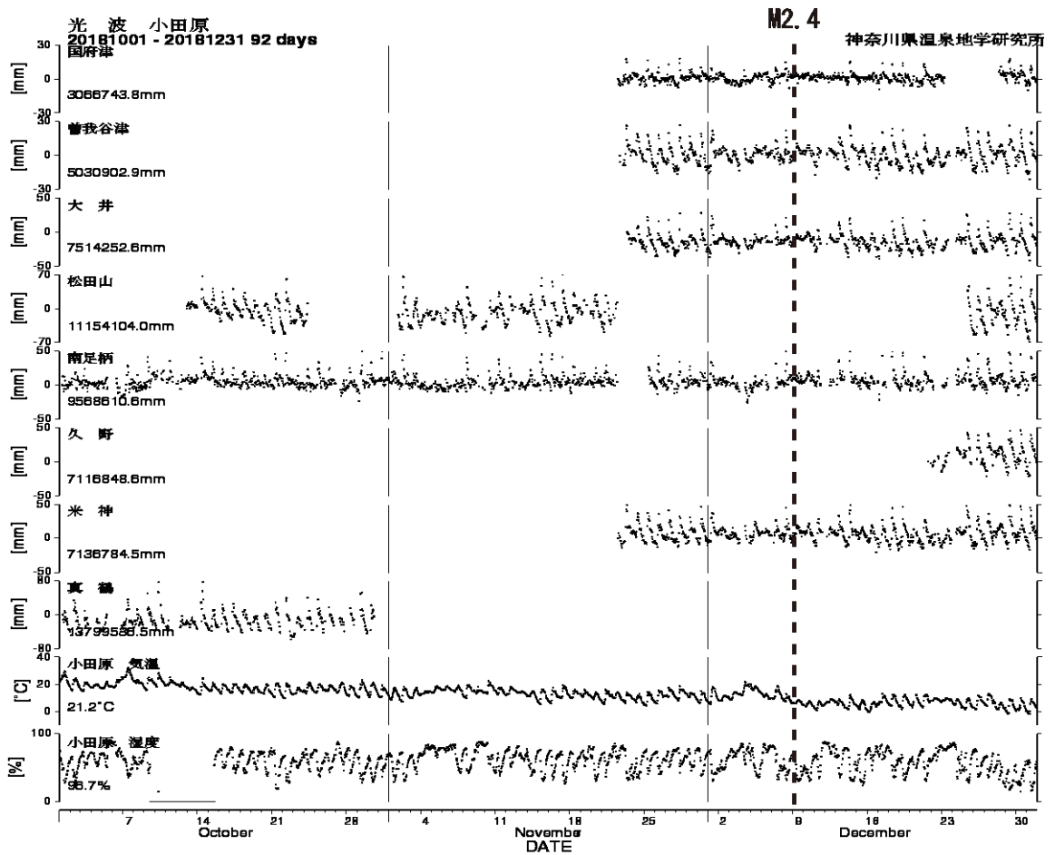
図5 光波測量（小田原観測網）観測結果（2018年10月01日～2018年12月31日） 計測システムの不調により、欠測している基線がある。
