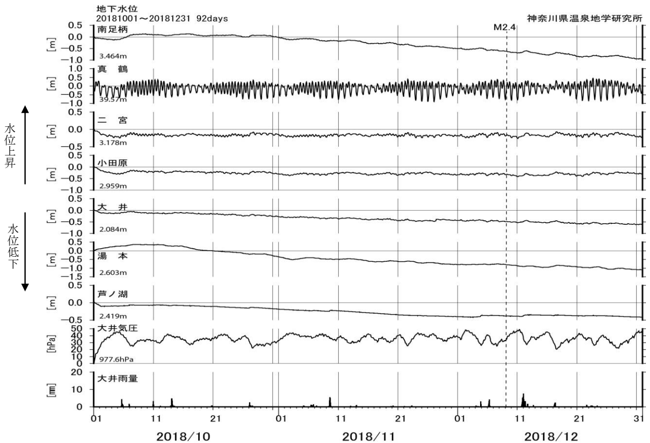
図6 地下水位観測結果（2018年10月～12月）
