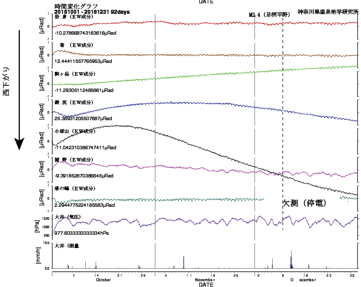
図3 傾斜計記録(2018年10月01日から2018年12月31日) 上:南北成分 下:東西成分
