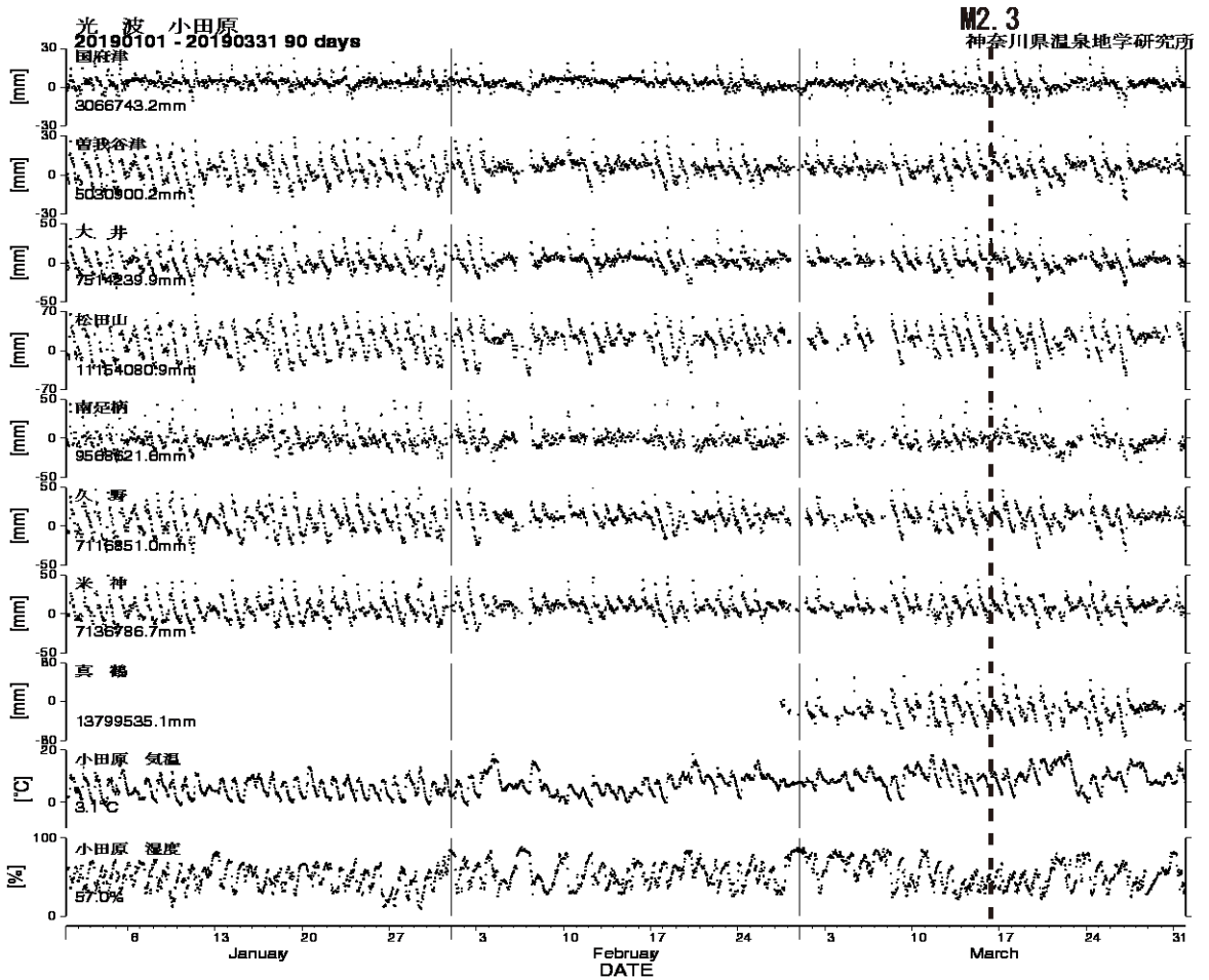
図5 光波測量（小田原観測網）観測結果（2019年01月01日～2019年03月31日）
