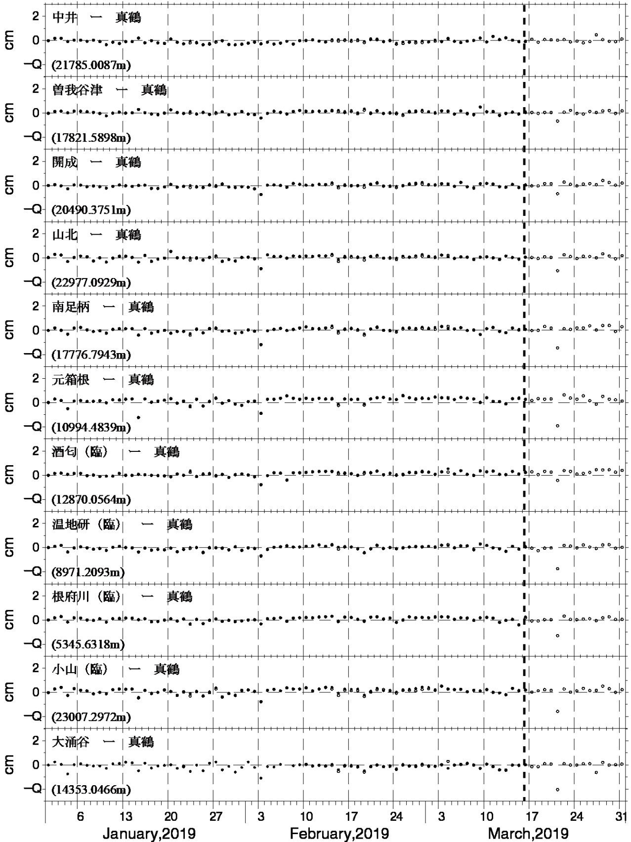
図4 GPS測量観測結果 (2019年01月01日~2019年03月31日) 真鶴観測点を中心とした、各観測点の基線長変化。●は精密暦、○は超速報暦による解を示す。
