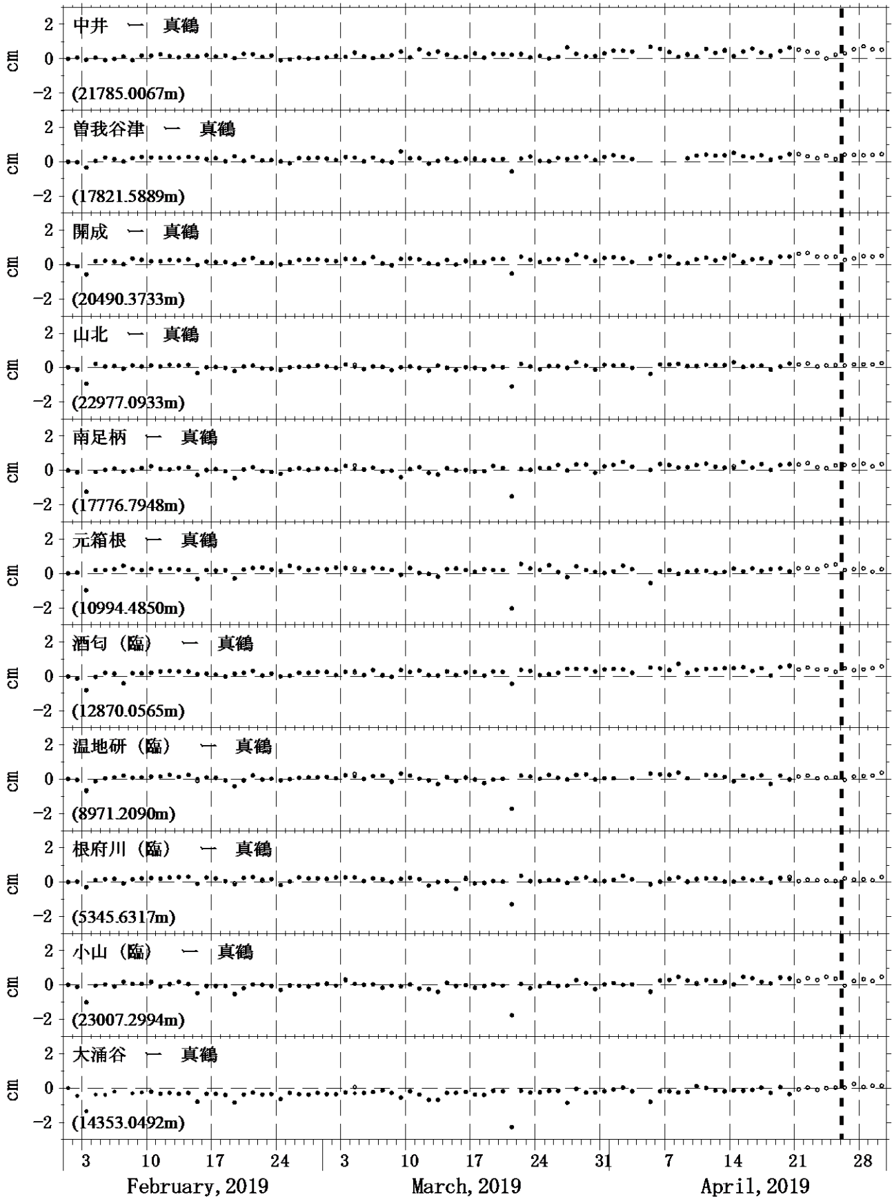
図4 GPS測量観測結果 (2019年02月01日~2019年04月30日)
