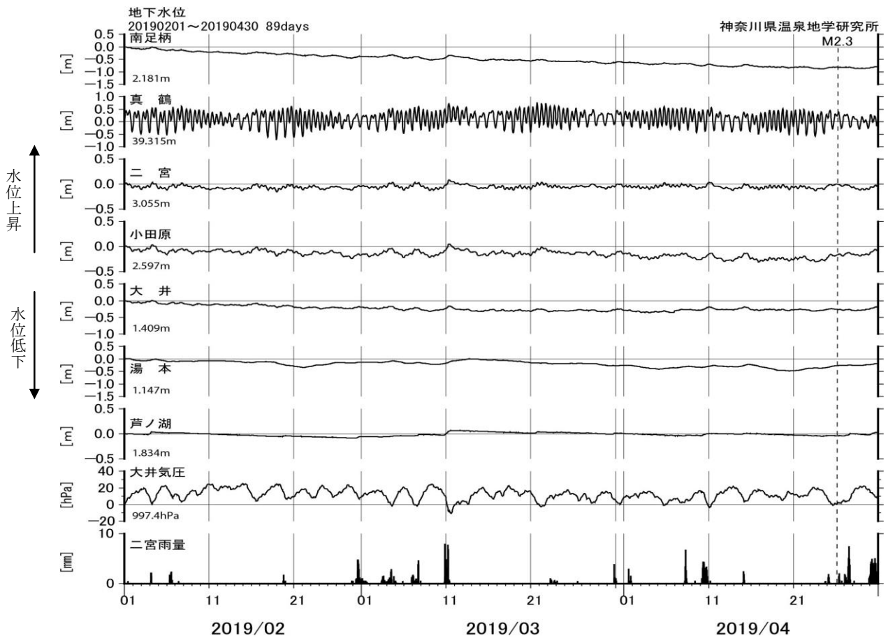
図6 地下水位観測結果（2019年02月01日～04月30日）
