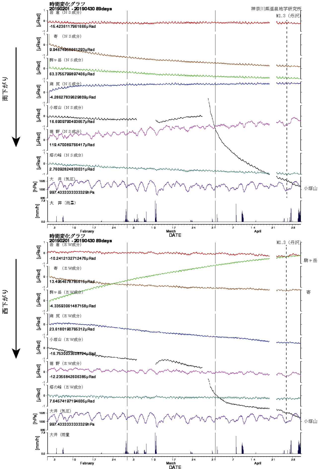
図3 傾斜計記録(2019年02月01日から2019年04月30日) 上:南北成分 下:東西成分 3月6日から9日までと、27日から29日まで小塚山のセンサー入れ替え作業。 4月20日から21日にかけて、サーバートラブルのため欠測。
