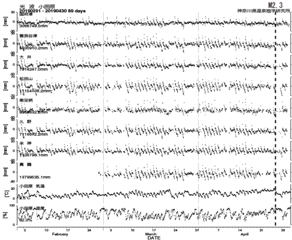
図5 光波測量（小田原観測網）観測結果（2019年02月01日～2019年04月30日）
