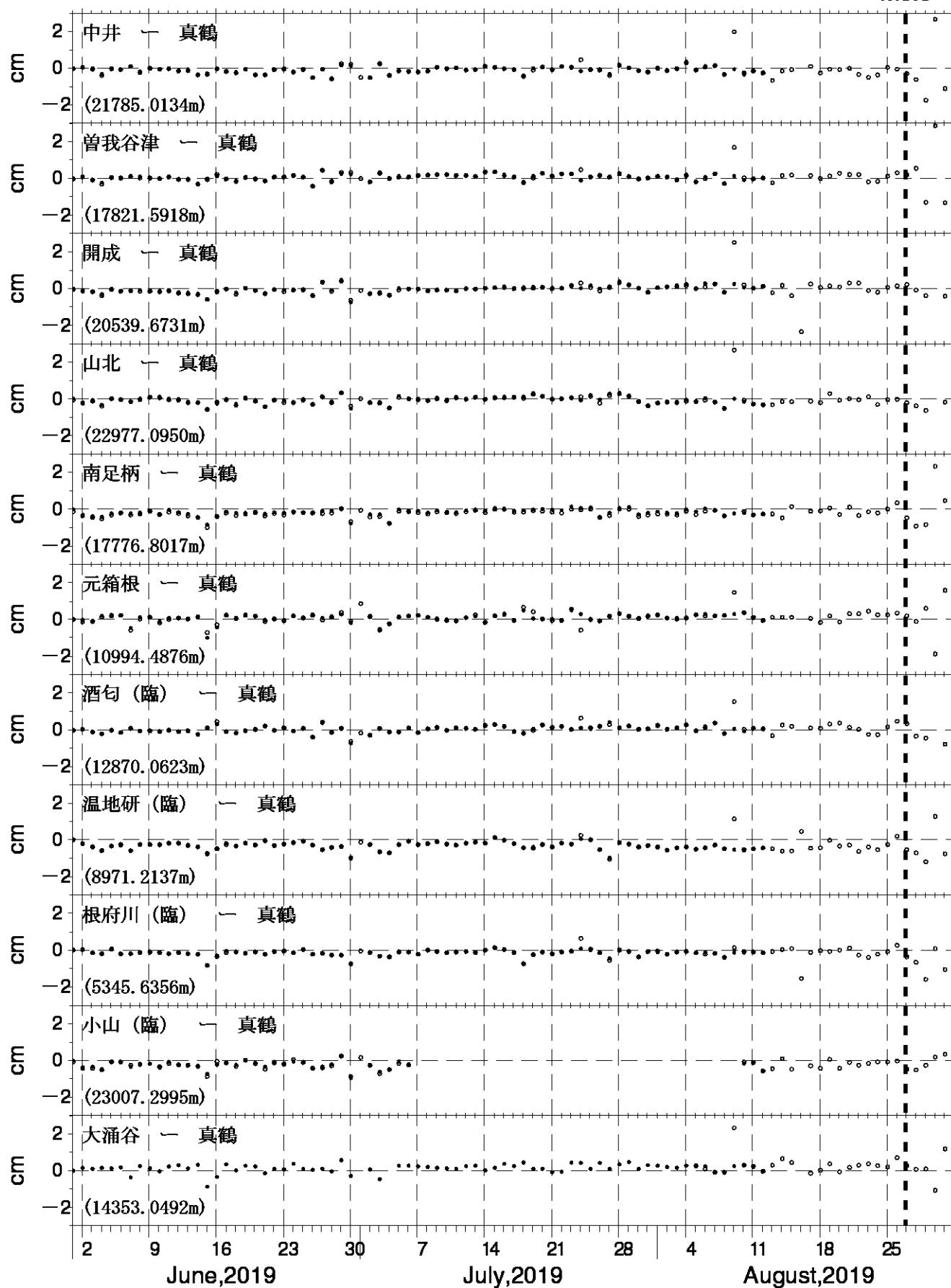
図4 GPS測量観測結果 (2019年06月01日～2019年08月31日) 真鶴観測点を中心とした、各観測点の基線長変化。●は精密暦、○は超速報暦による解を示す。
