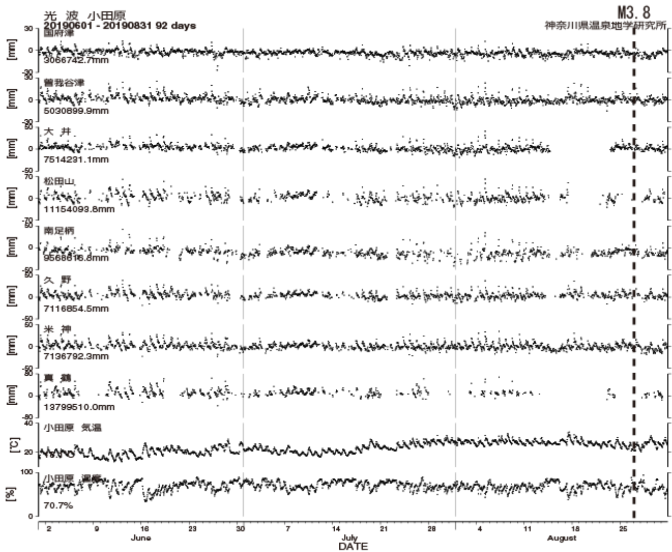
図5 光波測量（小田原観測網）観測結果（2019年06月01日～2019年08月31日）
