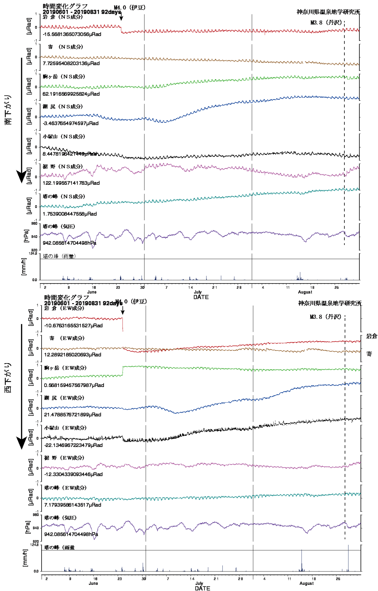
図3 傾斜計記録(2019年06月01日から2019年08月31日) 上:南北成分 下:東西成分
