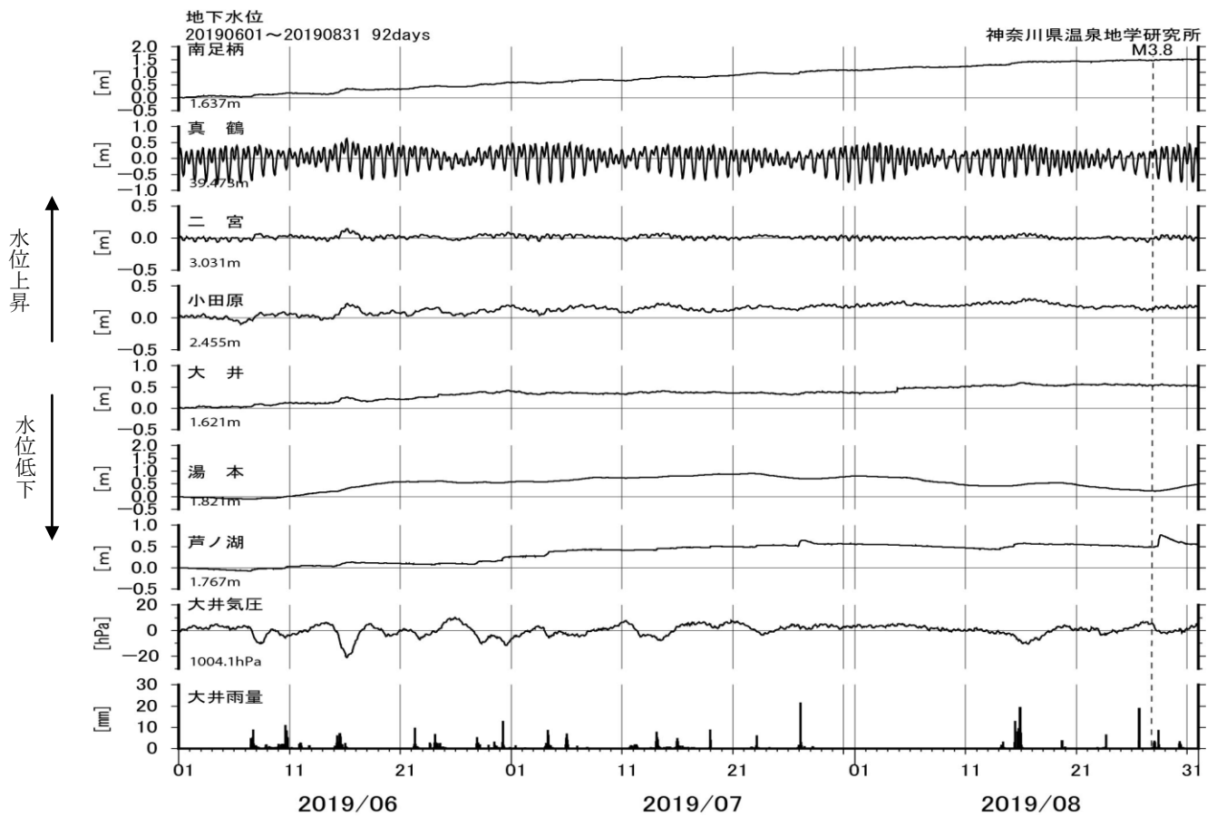
図6-1 地下水位観測結果(2019年06月01日~2019年08月31日)
