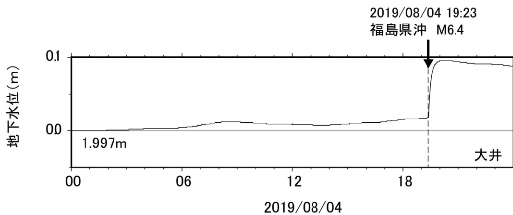
図6-2 地震の影響とみられる水位の変化(2019年8月4日)
