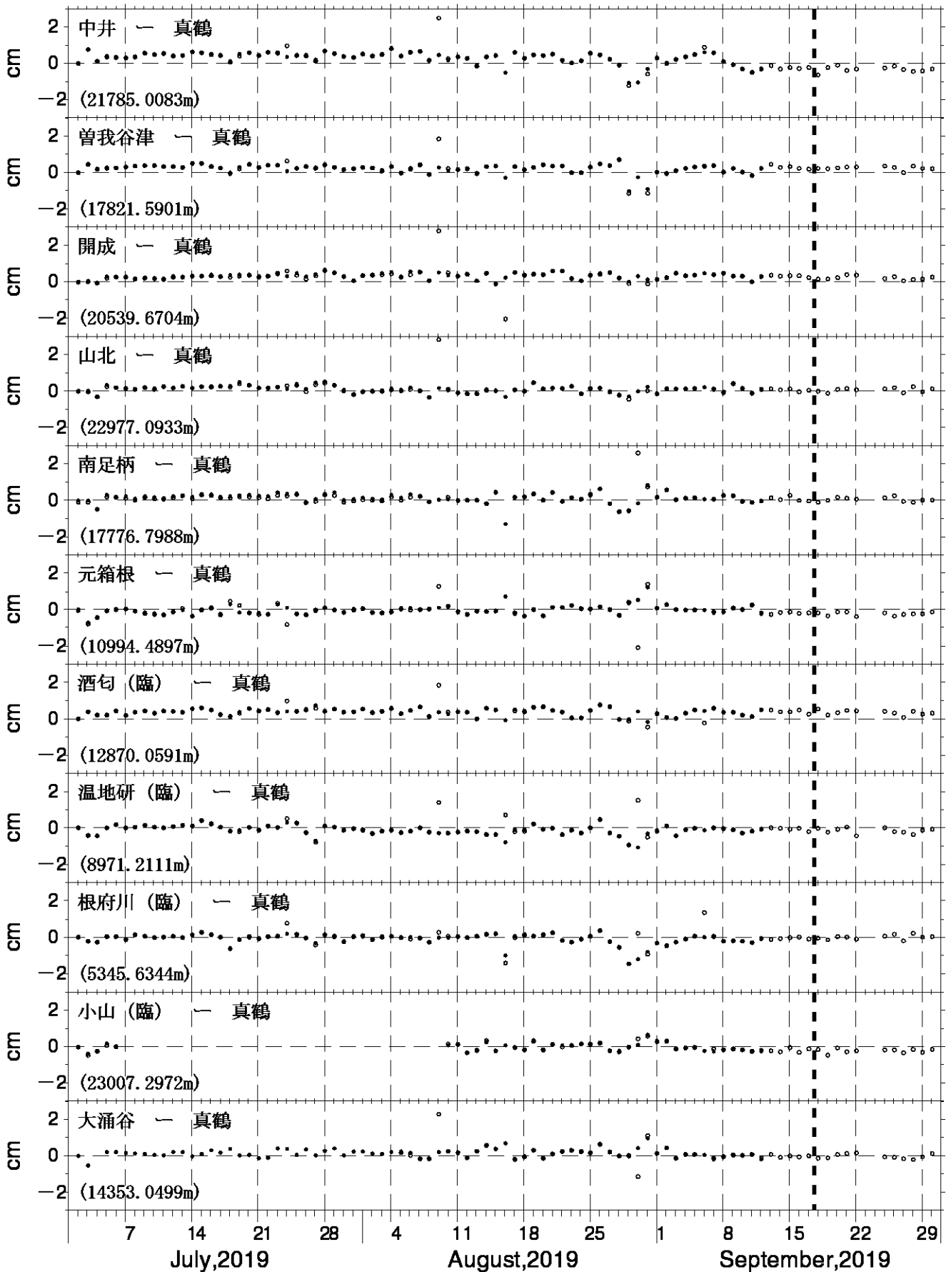
図4 GPS測量観測結果 (2019年07月01日~2019年09月30日)
