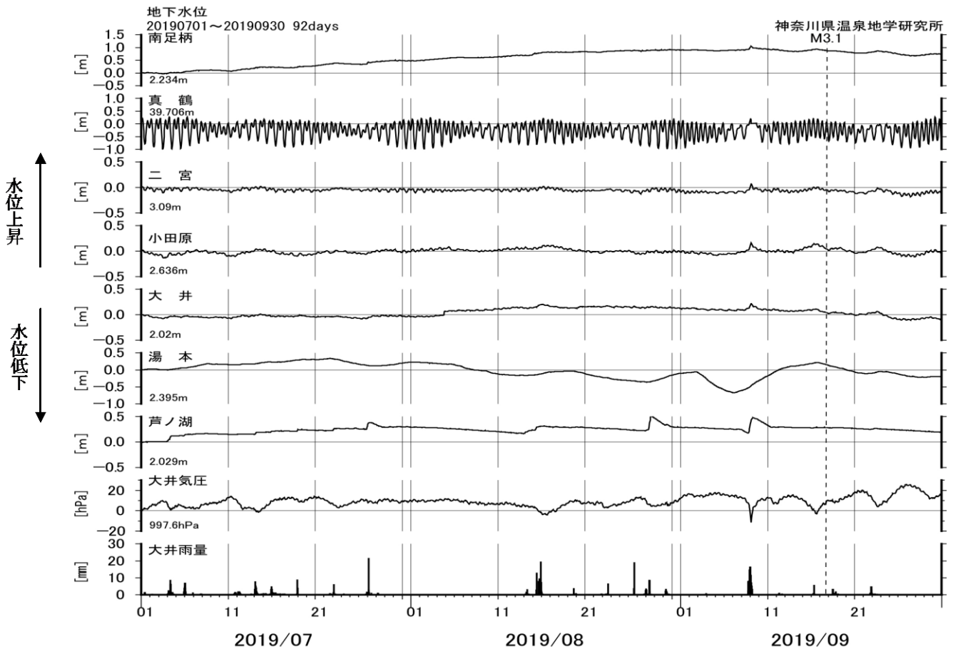
図6 地下水水位観測結果（2019年07月01日～2019年09月30日）
