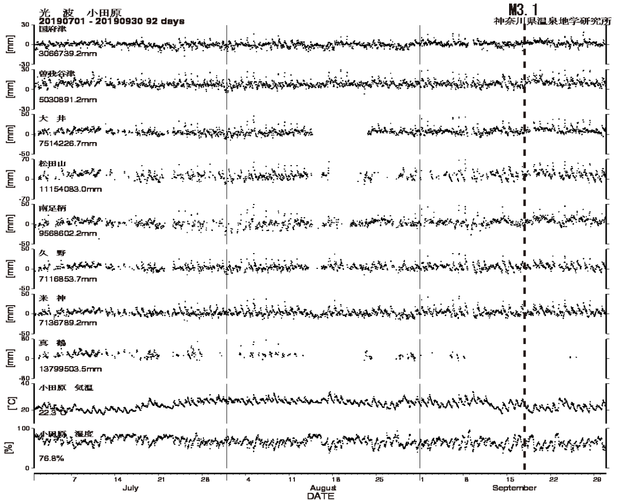
図5 光波測量（小田原観測網）観測結果（2019年07月01日～2019年09月30日）
