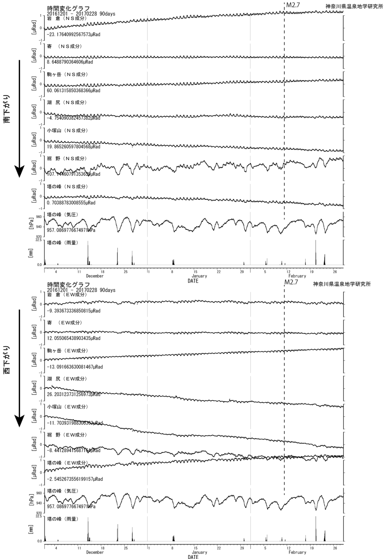
図3 傾斜計記録(2016年12月1日から2017年2月28日) 上:南北成分 下:東西成分
