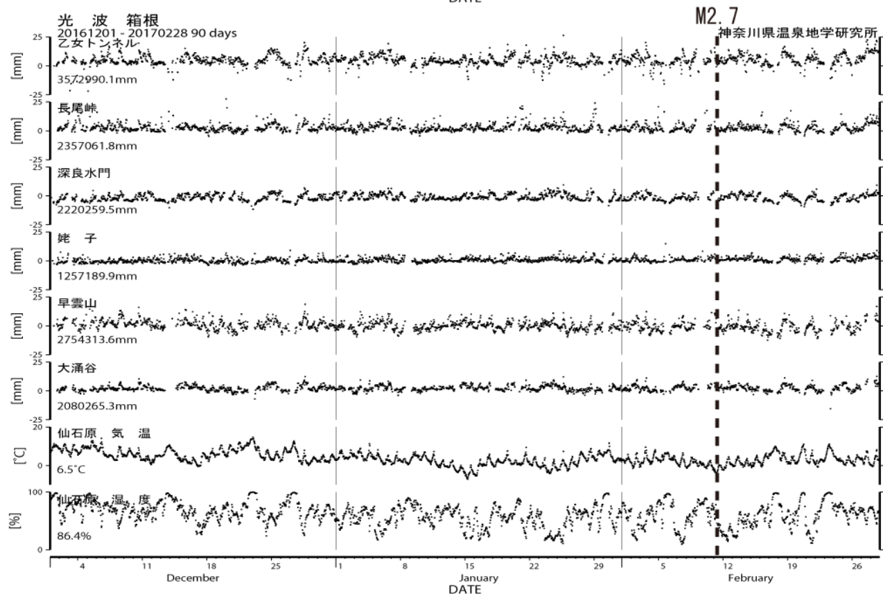
図5 光波測量観測結果 (2016年12月01日~2017年02月28日) 上: 小田原観測網、下: 箱根観測網
