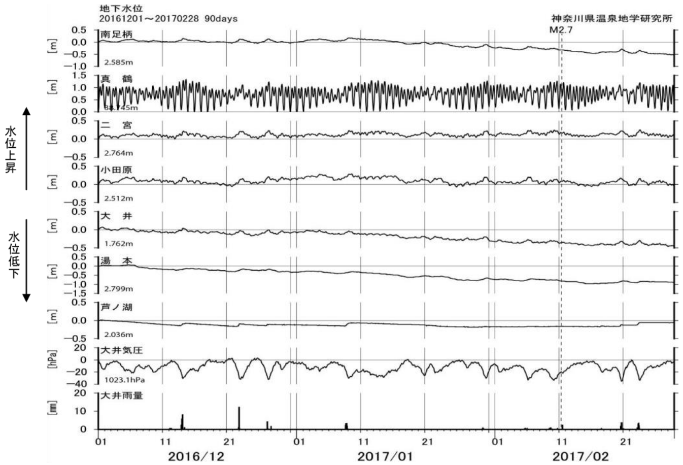
図 6-1 地下水位観測結果 (2016年12月～2017年2月)
