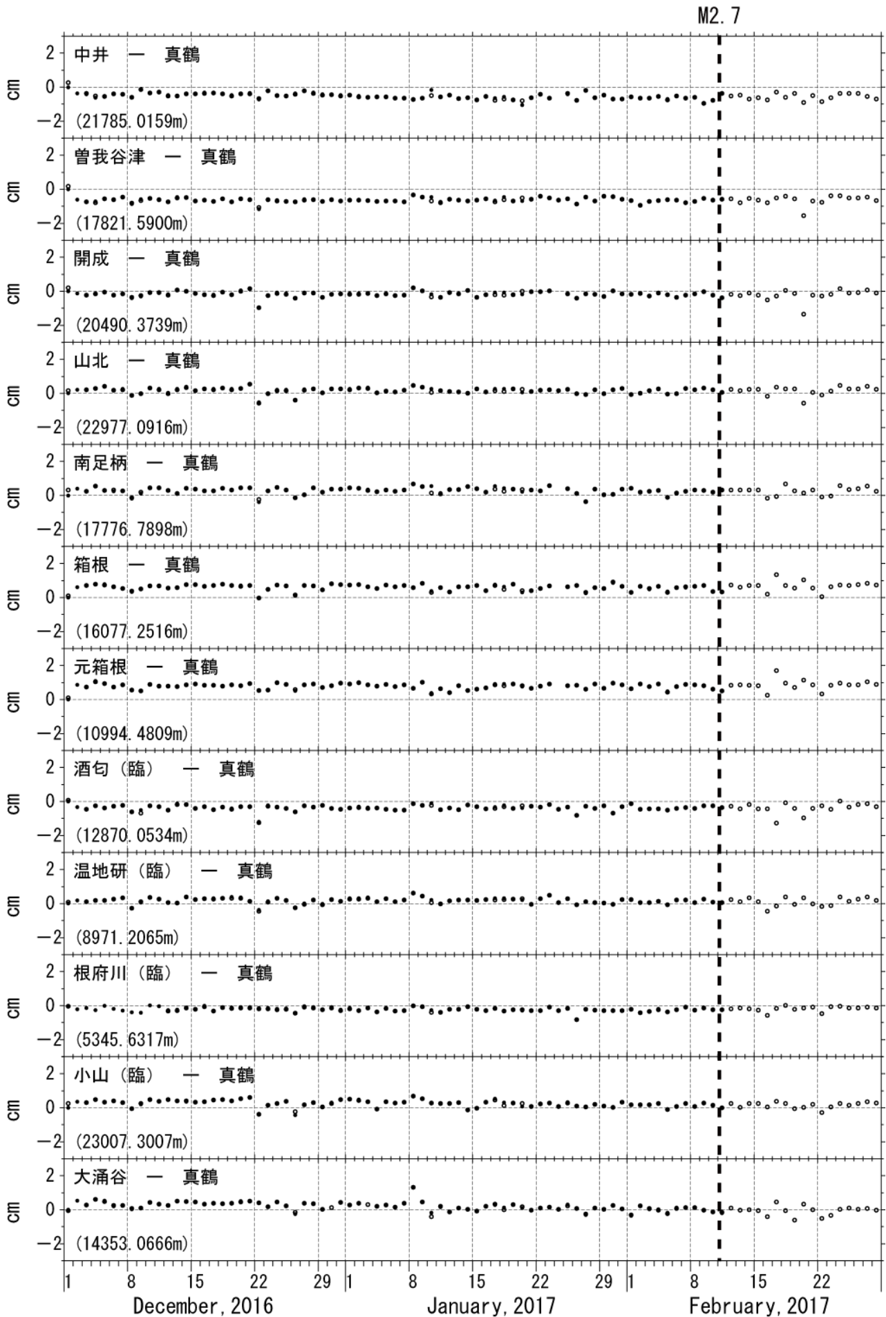
図4 GPS測量観測結果 (2016年12月01日~2017年02月28日) 真鶴観測点を中心とした、各観測点の基線長変化。●は精密暦、○は超速報暦による解を示す。
