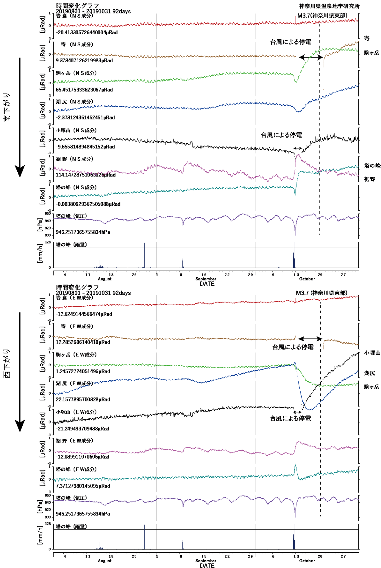
図3 傾斜計記録(2019年08月01日から2019年10月31日) 上:南北成分 下:東西成分
