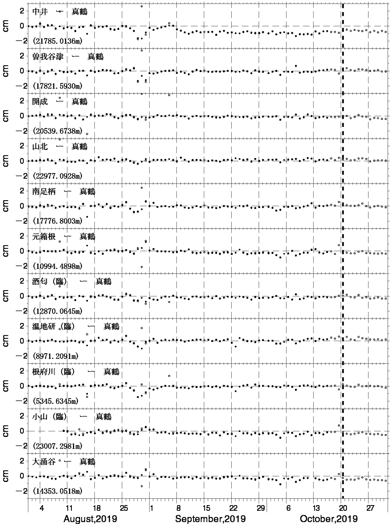
図4 GPS測量観測結果 (2019年08月01日~2019年10月31日)
