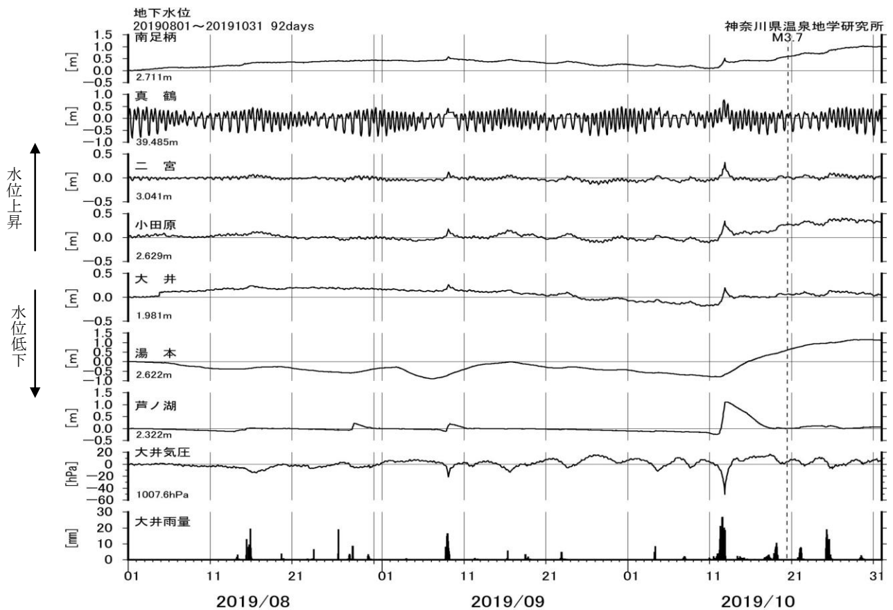
図6-1 地下水位観測結果(2019年08月01日～2019年10月31日)
