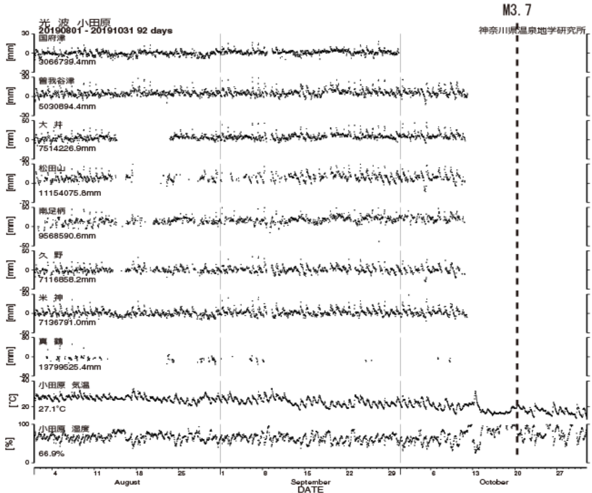
図5 光波測量（小田原観測網）観測結果（2019年08月01日～2019年10月31日）
