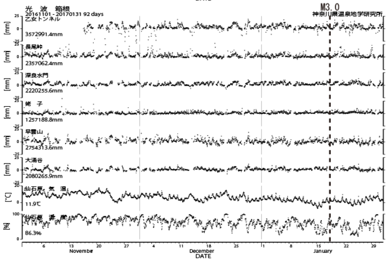
図5 光波測量観測結果 (2016年11月01日~2017年01月31日) 上: 小田原観測網、下: 箱根観測網
