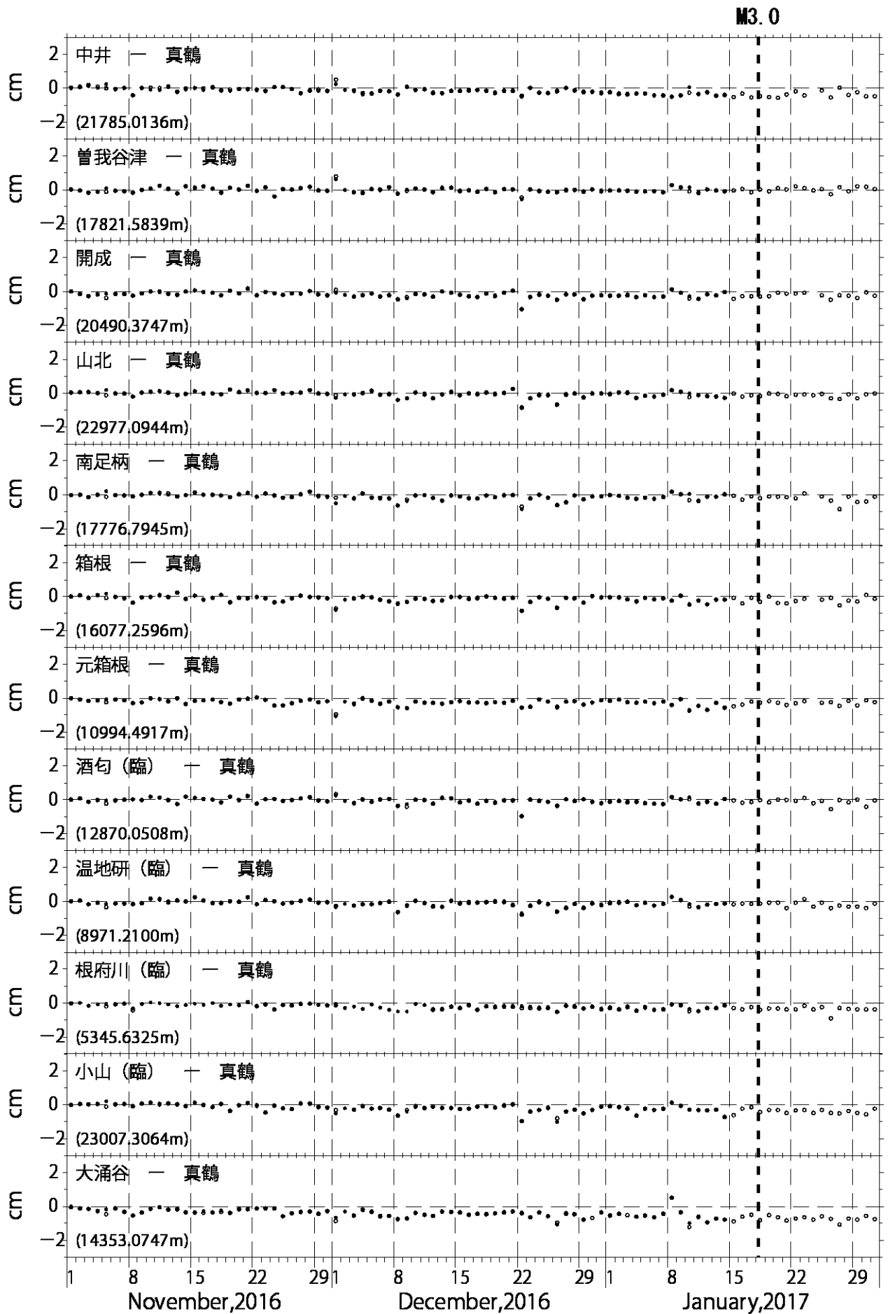
図4 GPS測量観測結果 (2016年11月01日~2017年01月31日) 真鶴観測点を中心とした、各観測点の基線長変化。●は精密暦、○は超速報暦による解を示す。
