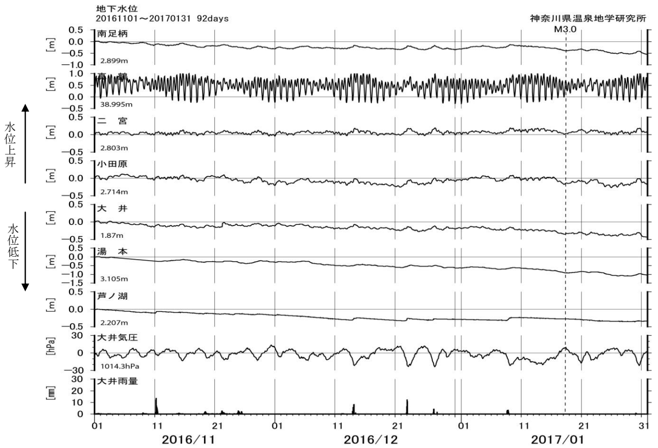
図6 地下水位観測結果(2016年11月~2017年1月)
