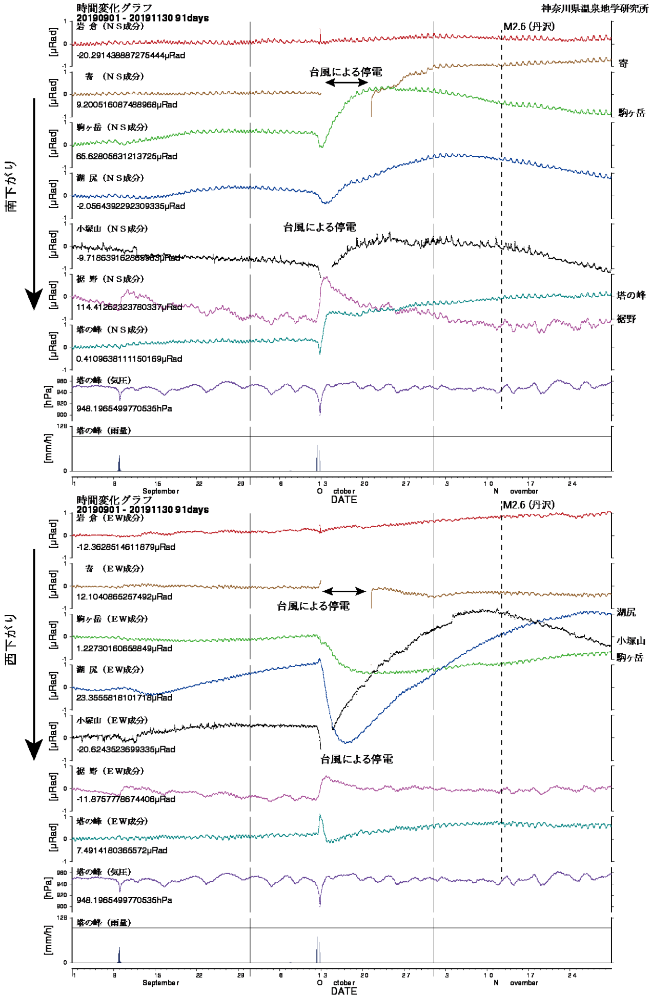
図3 傾斜計記録(2019年09月01日から2019年11月30日) 上:南北成分 下:東西成分
