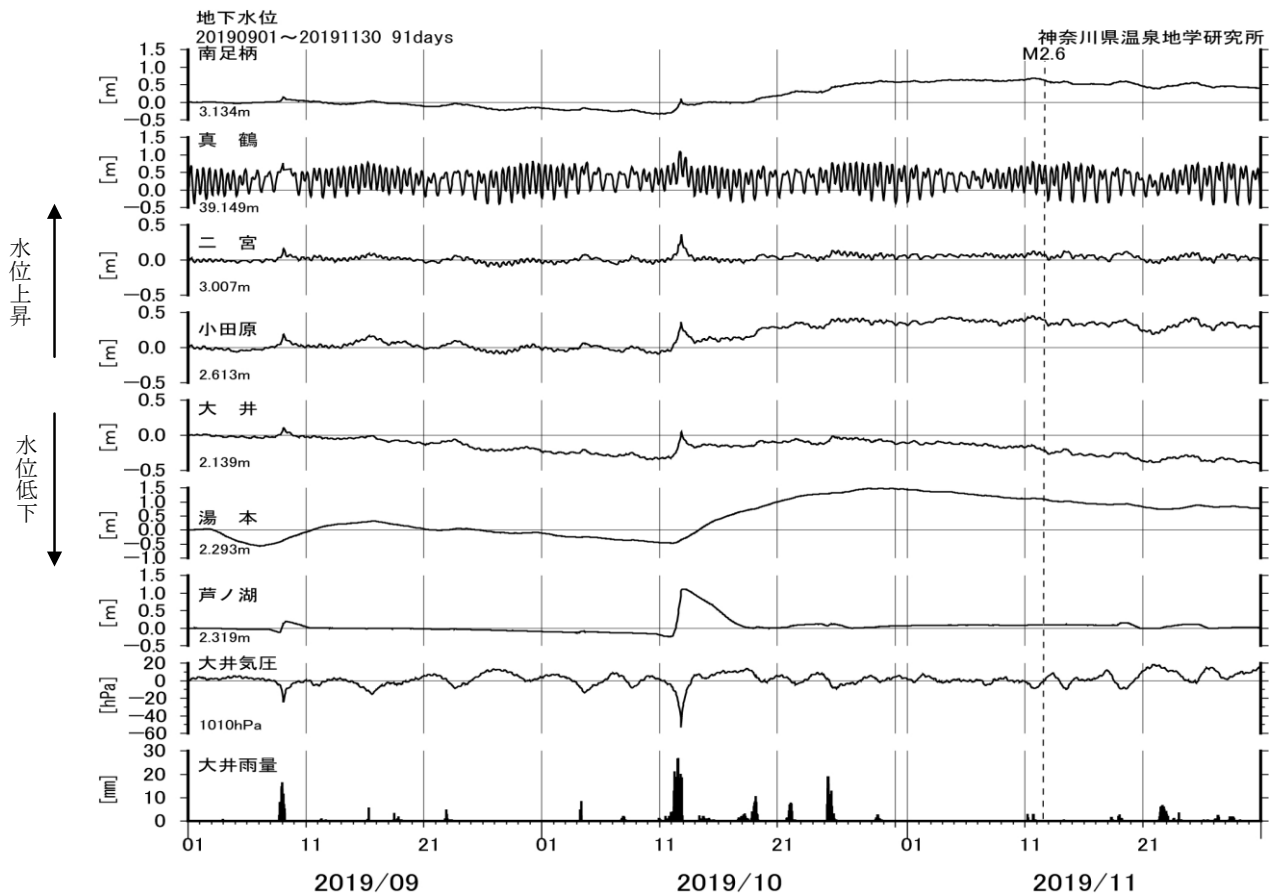
図6 地下水位観測結果(2019年09月01日～2019年11月30日)
