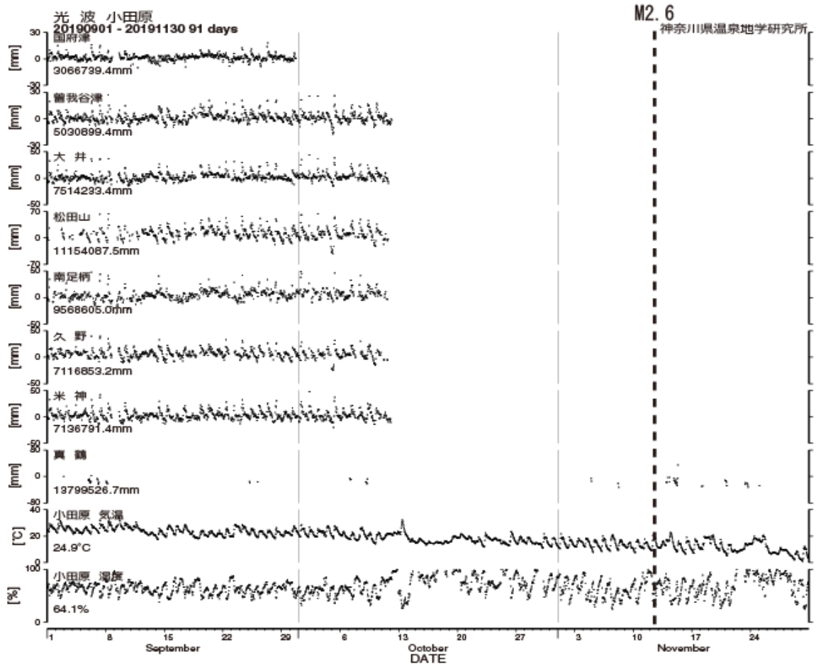
図5 光波測量（小田原観測網）観測結果（2019年09月01日～2019年11月30日） （台風19号の影響により欠測中）
