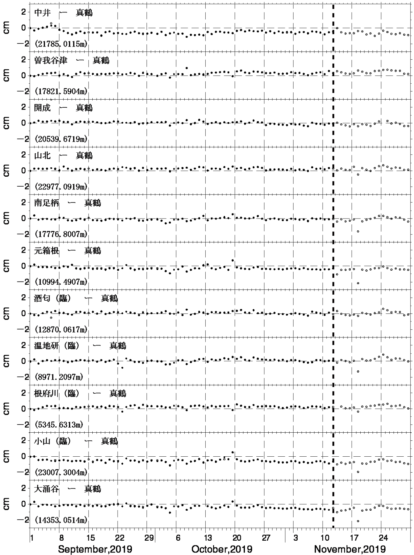
図4 GPS測量観測結果 (2019年09月01日~2019年11月30日) 真鶴観測点を中心とした、各観測点の基線長変化。●は精密暦、○は超速報暦による解を示す。
