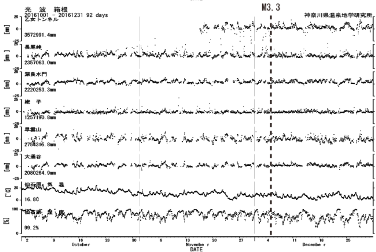
図5 光波測量観測結果 (2016年10月01日~2016年12月31日) 上: 小田原観測網、下: 箱根観測網
