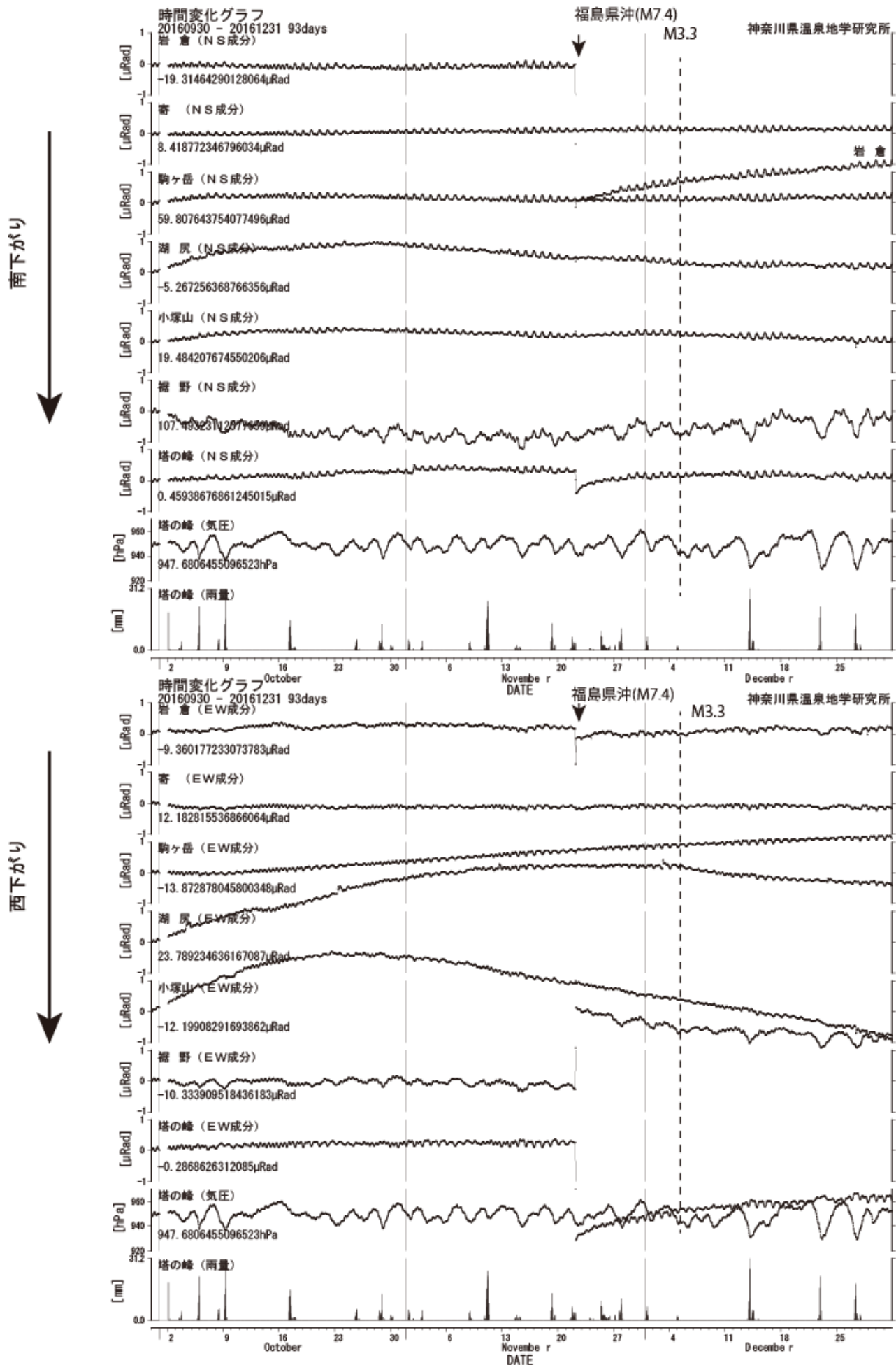
図3 傾斜計記録(2016年9月30日から2016年12月31日) 上:南北成分 下:東西成分
