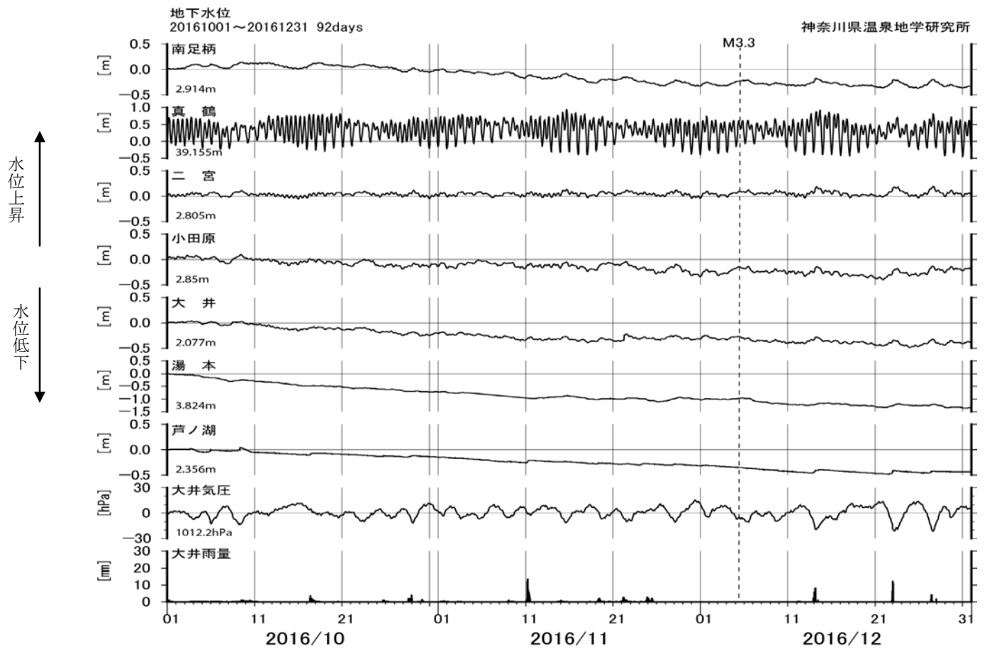
図6 地下水位観測結果(2016年10月~12月)
