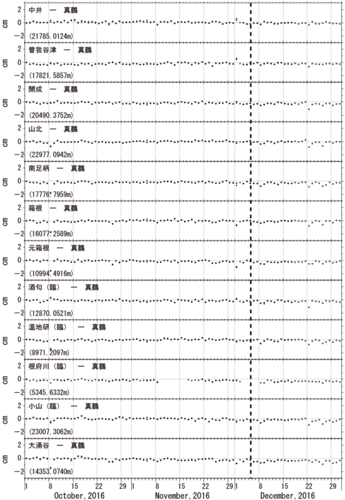
図4 GPS測量観測結果 (2016年10月01日~2016年12月31日)
