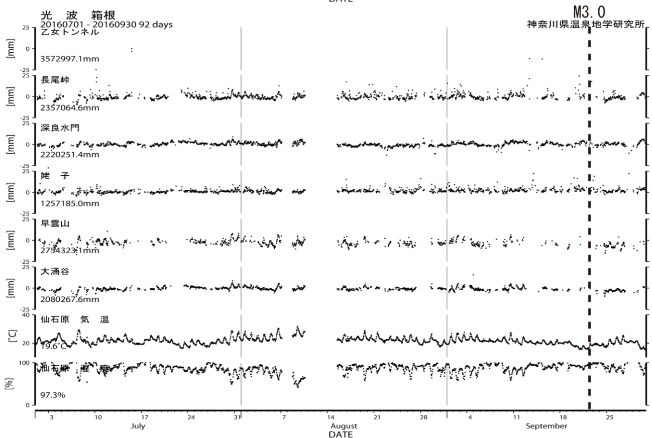
図5 光波測量観測結果 (2016年07月01日~2016年09月30日)
