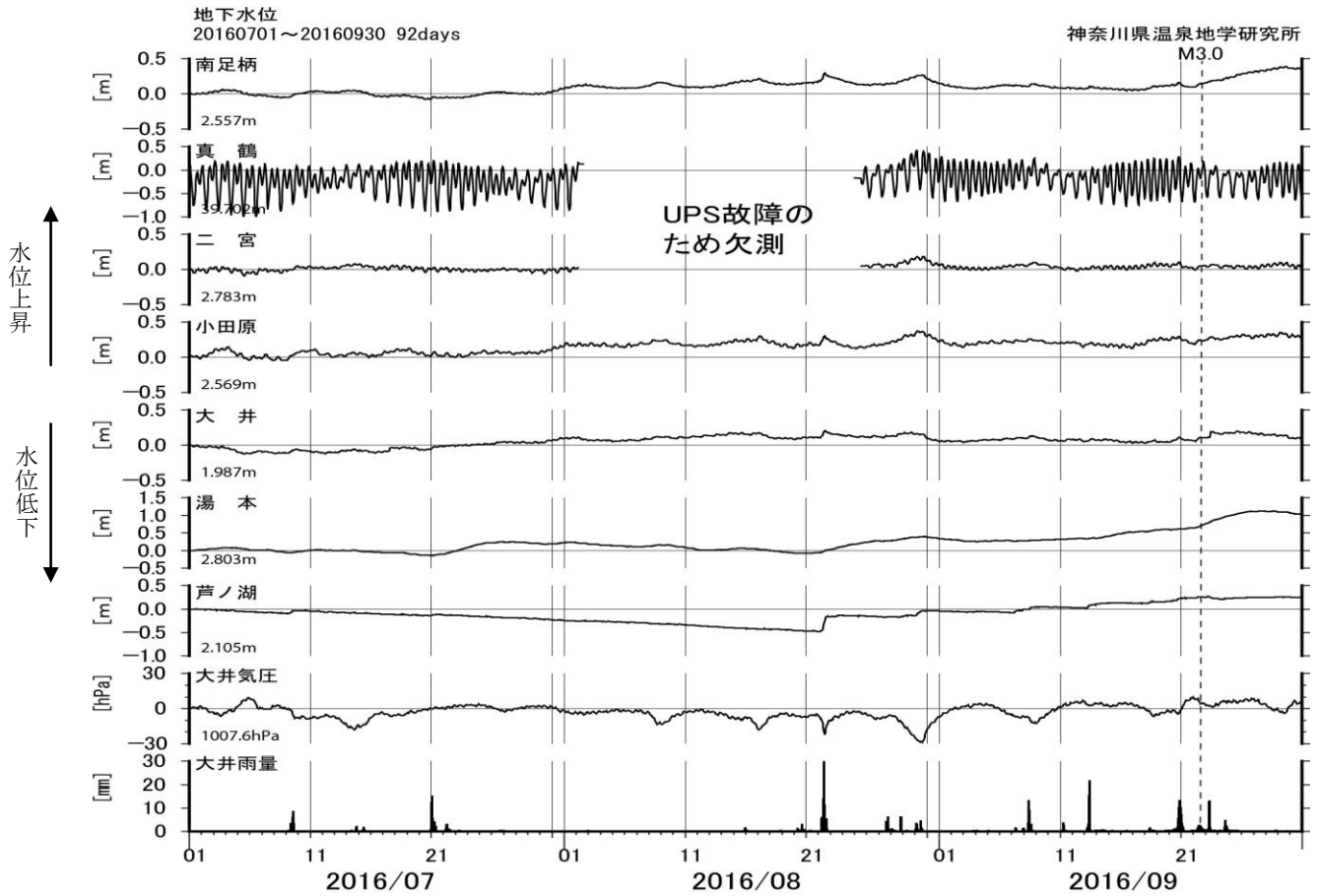
図6-1 地下水位観測結果(2016年7月~9月)
