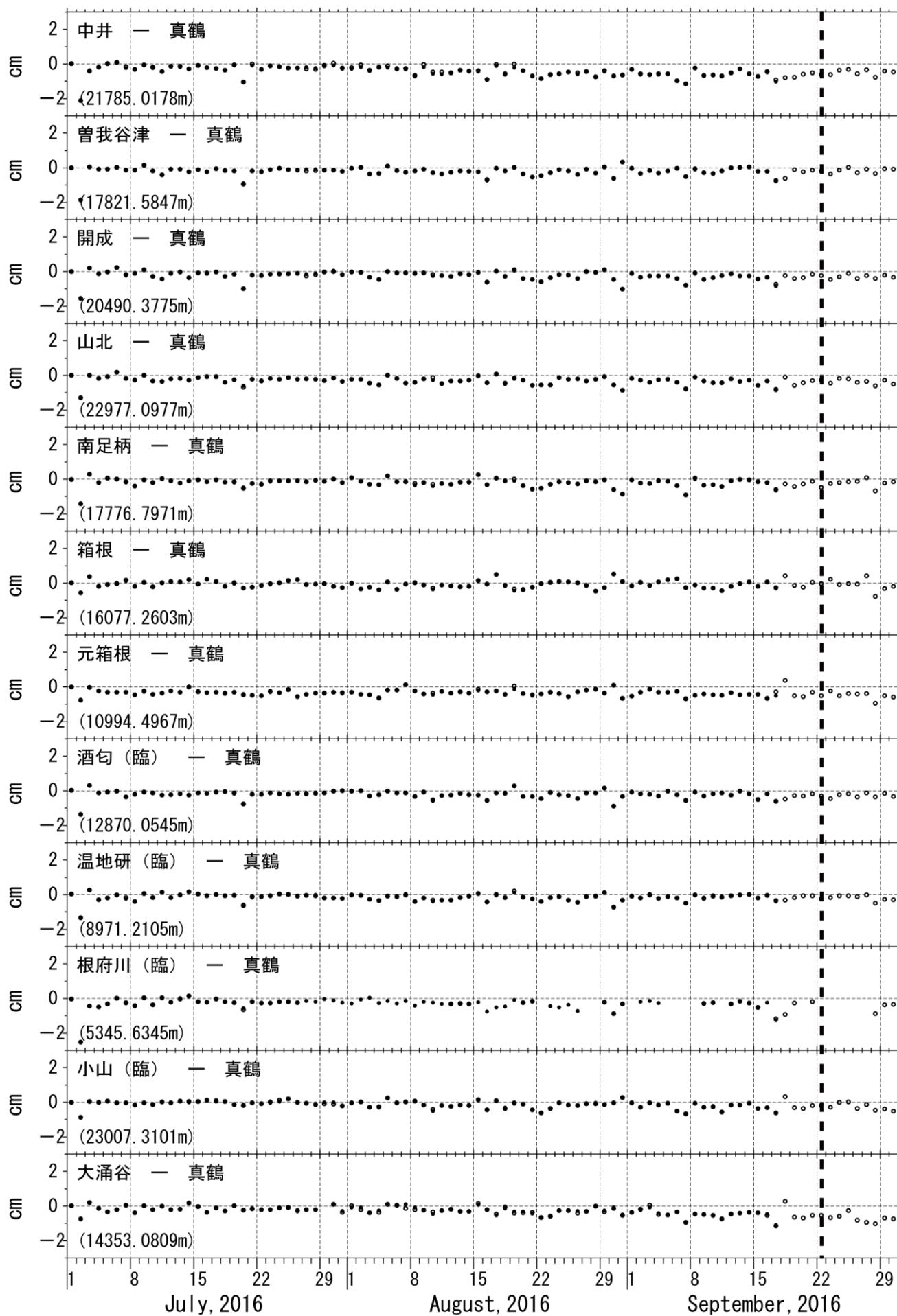
図4 GPS測量観測結果 (2016年07月01日~2016年09月30日)
