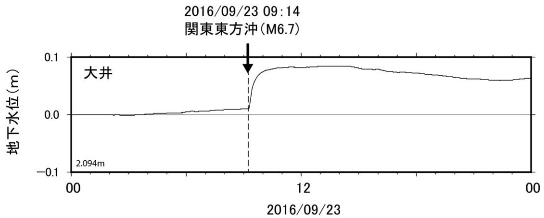
図6-2 地震の影響とみられる水位変化(2016年9月23日)
