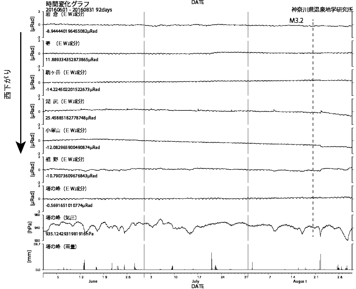
図3 傾斜計記録(2016年6月1日から2016年8月31日) 上:南北成分 下:東西成分
