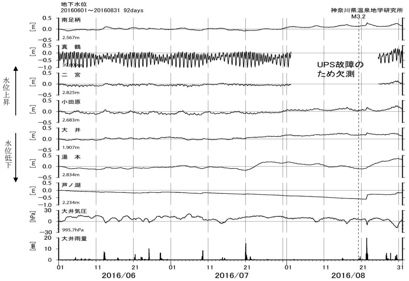
図6 地下水位観測結果(2016年6月~8月)
