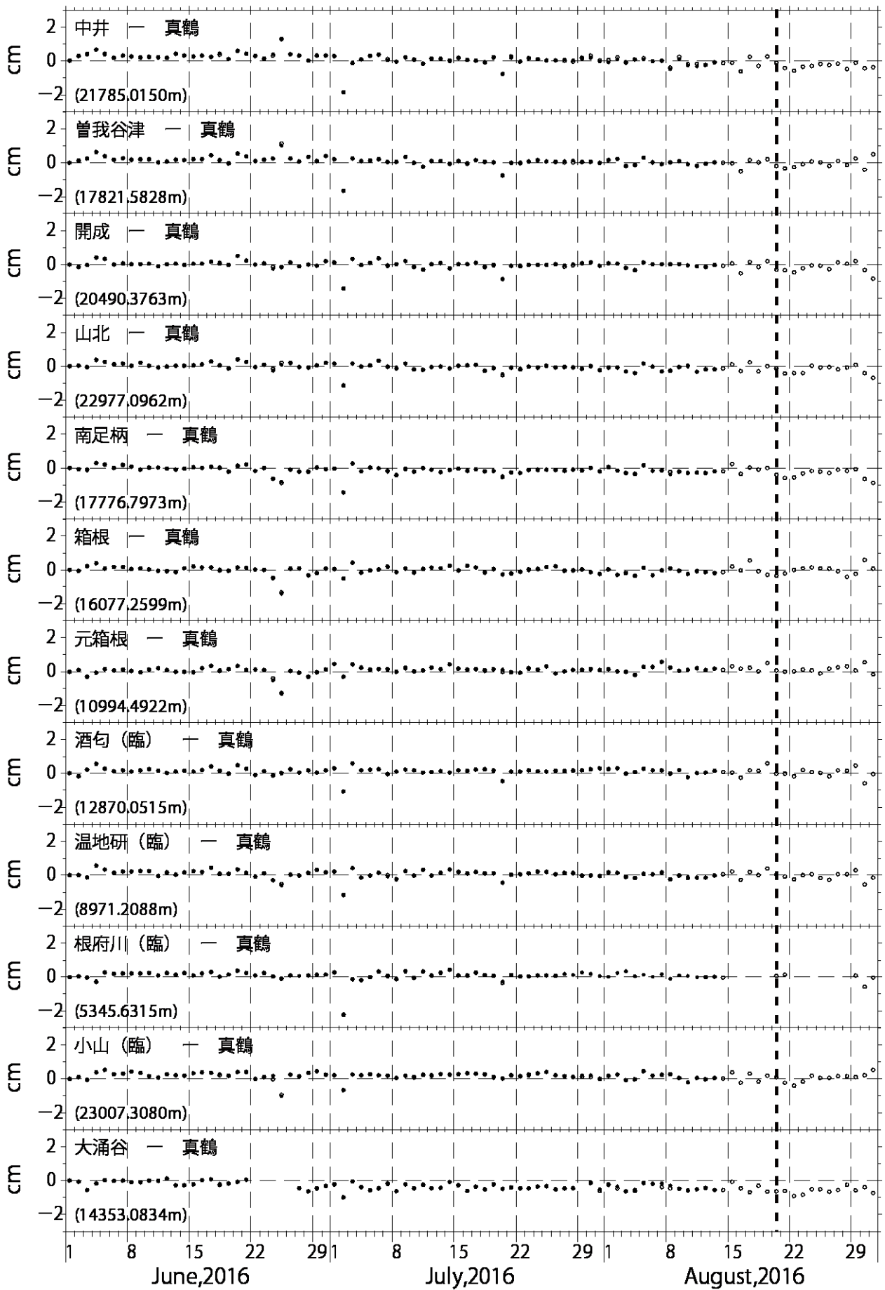
図4 GPS測量観測結果 (2016年06月01日~2016年08月31日)
