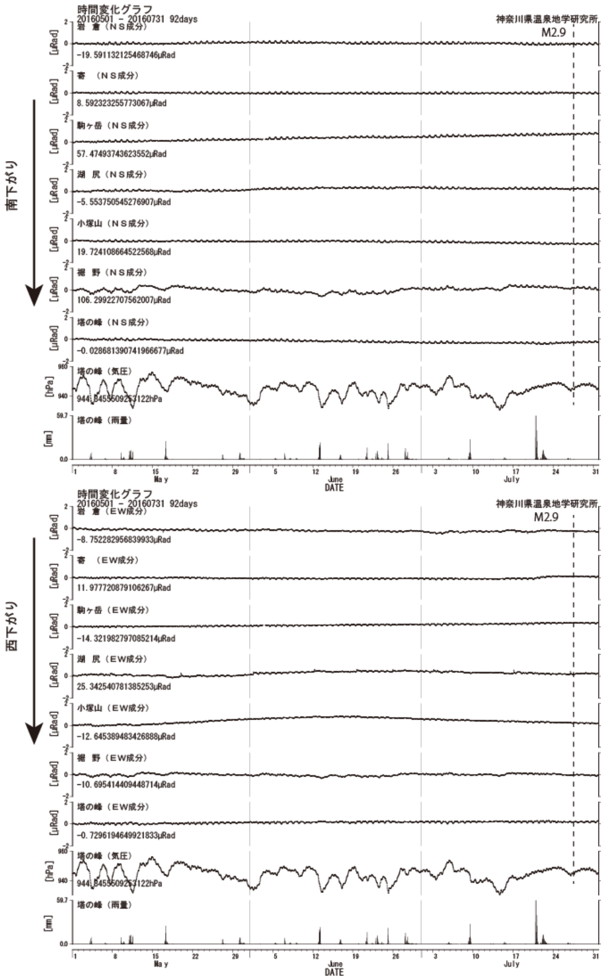
図3 傾斜計記録(2016年5月1日から2016年7月31日) 上:南北成分 下:東西成分
