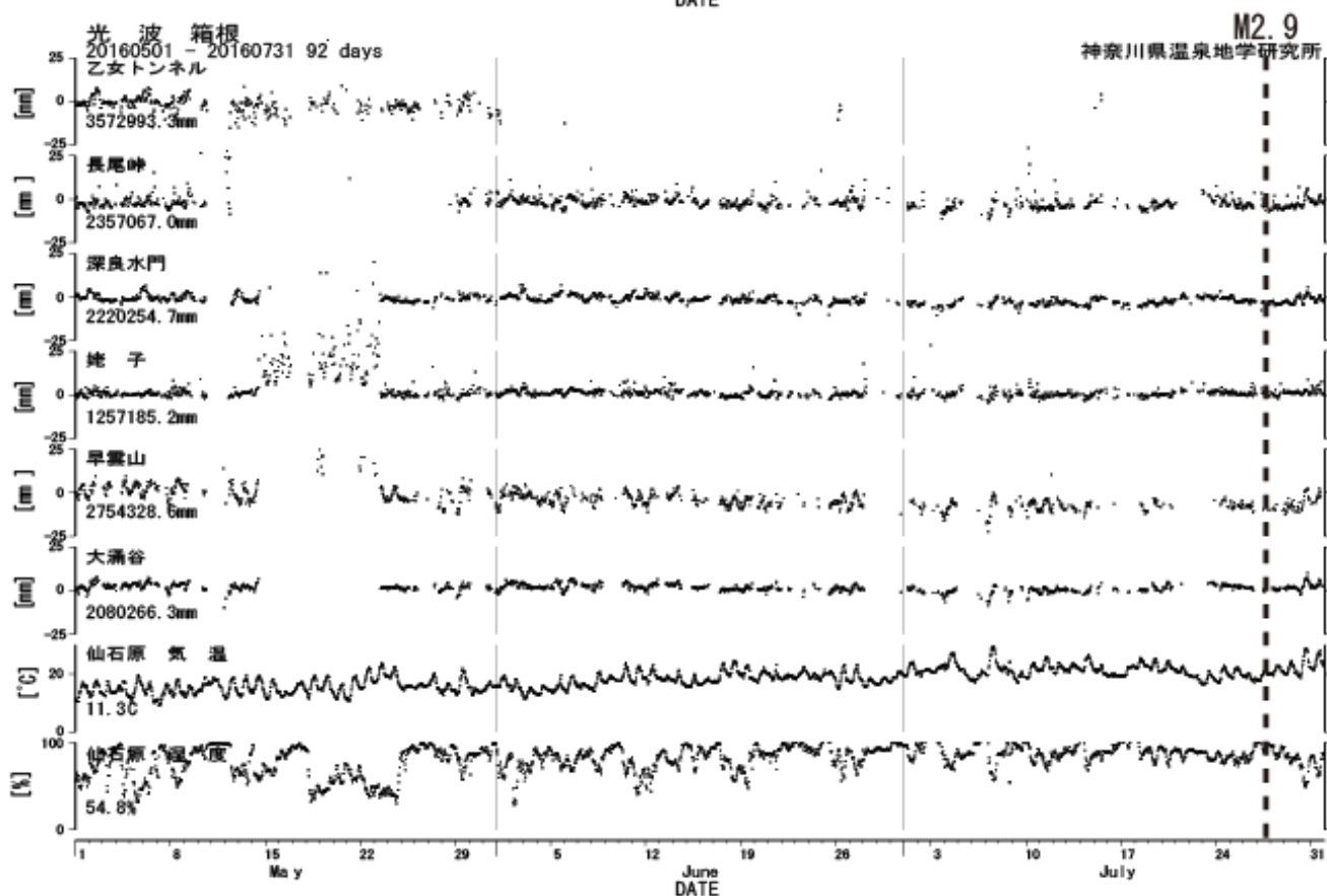
図5 光波測量観測結果 (2016年05月01日~2016年07月31日) 上: 小田原観測網、下: 箱根観測網
