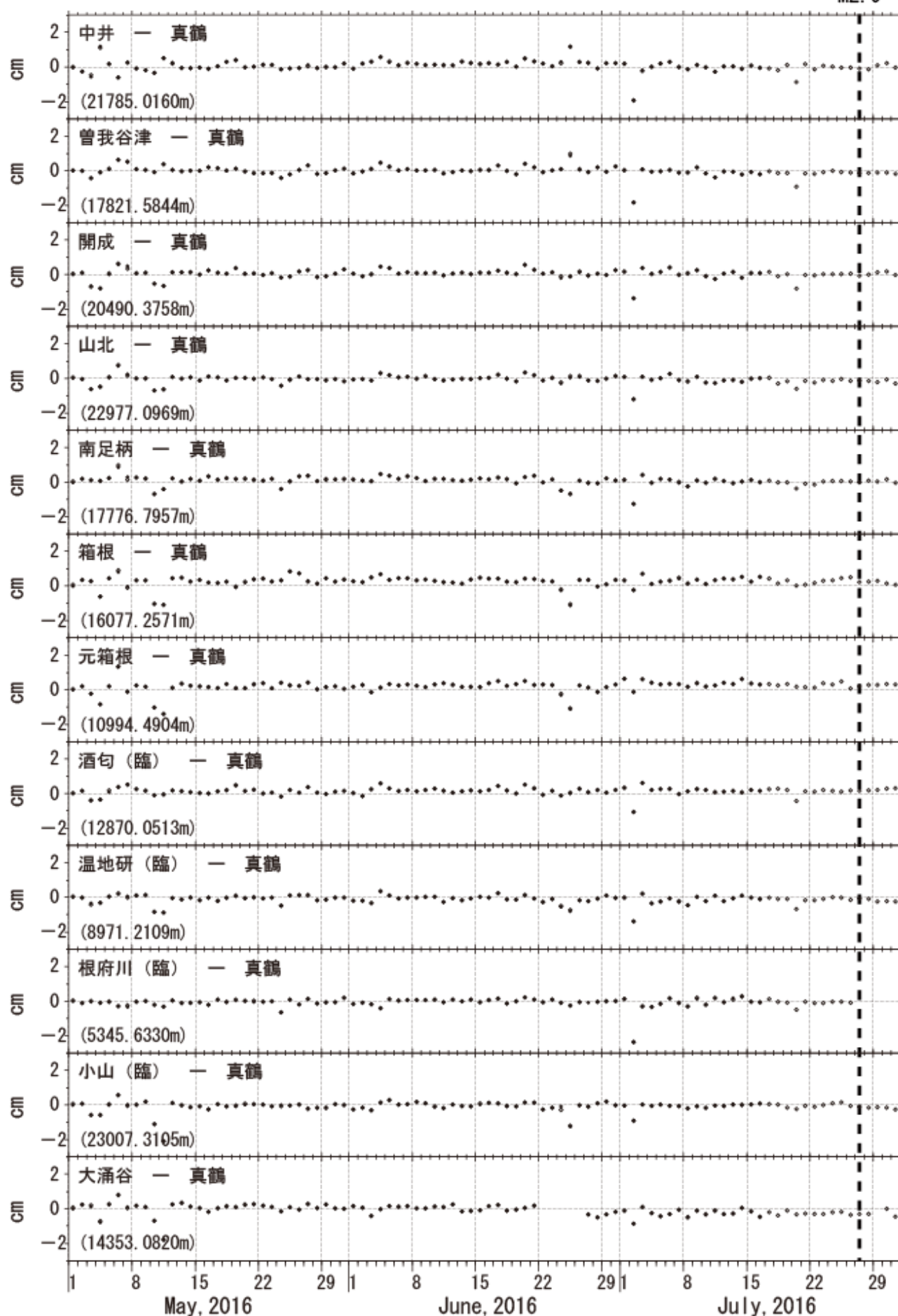
図4 GPS測量観測結果 (2016年05月01日~2016年07月31日)
