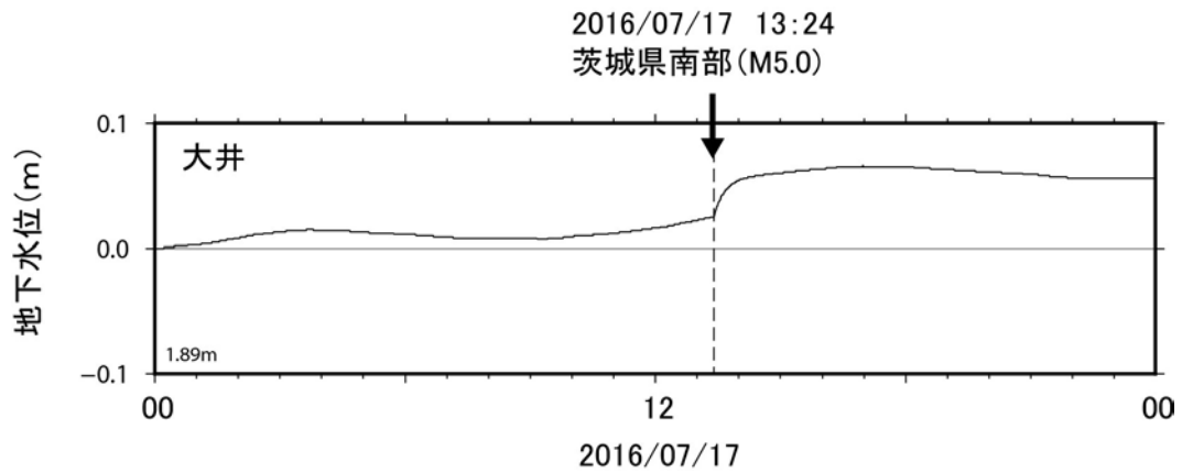
図6-2 地震の影響とみられる水位変化(2016年7月17日)
