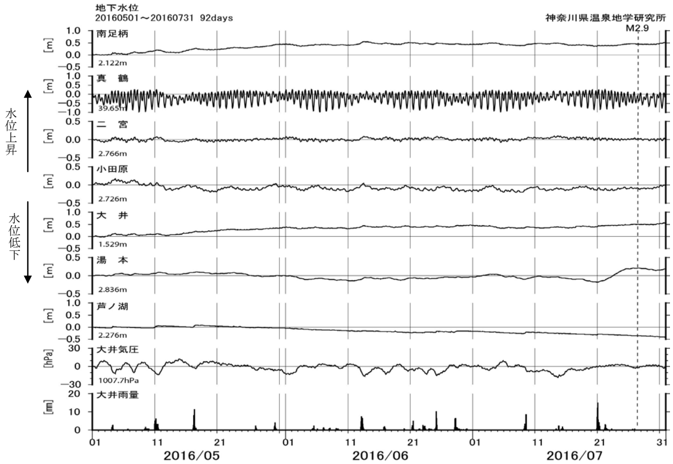
図6-1 地下水水位観測結果(2016年5月~7月)
