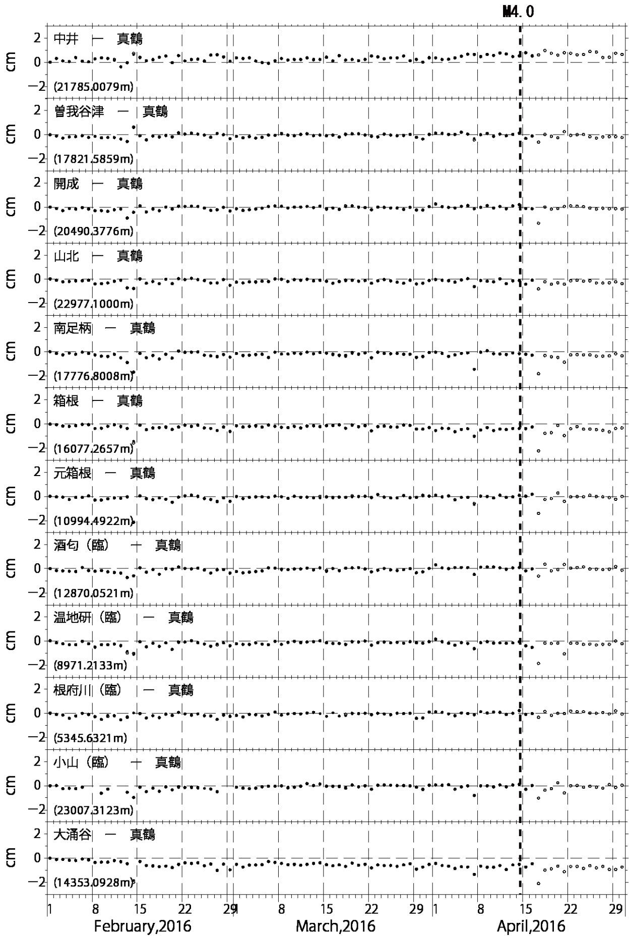
図4 GPS測量観測結果（2016年02月01日～2016年04月30日） 真鶴観測点を中心とした、各観測点の基線長変化。●は精密暦、○は超速報暦による解を示す。 小山観測点は、（独）防災科学技術研究所との共同研究による観測点である。
