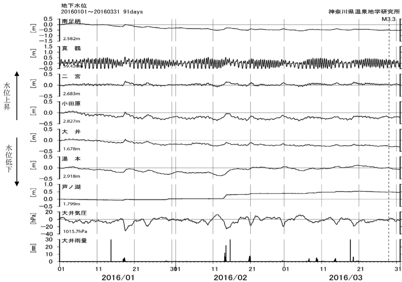
図6 地下水位観測結果(2016年1月~2016年3月)
