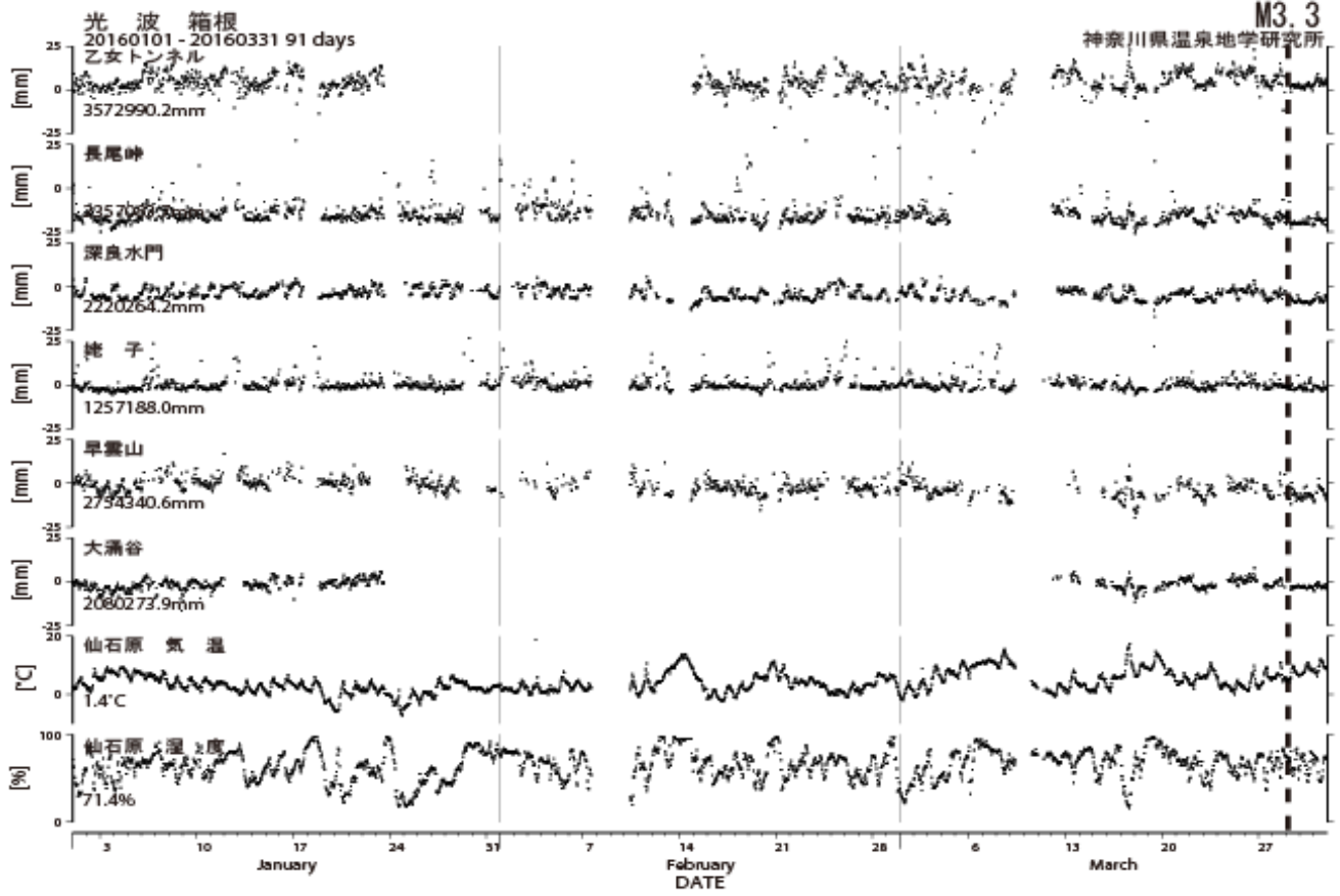
図5 光波測量観測結果（2016年01月01日～2016年03月31日） 上：小田原観測網、下：箱根観測網
