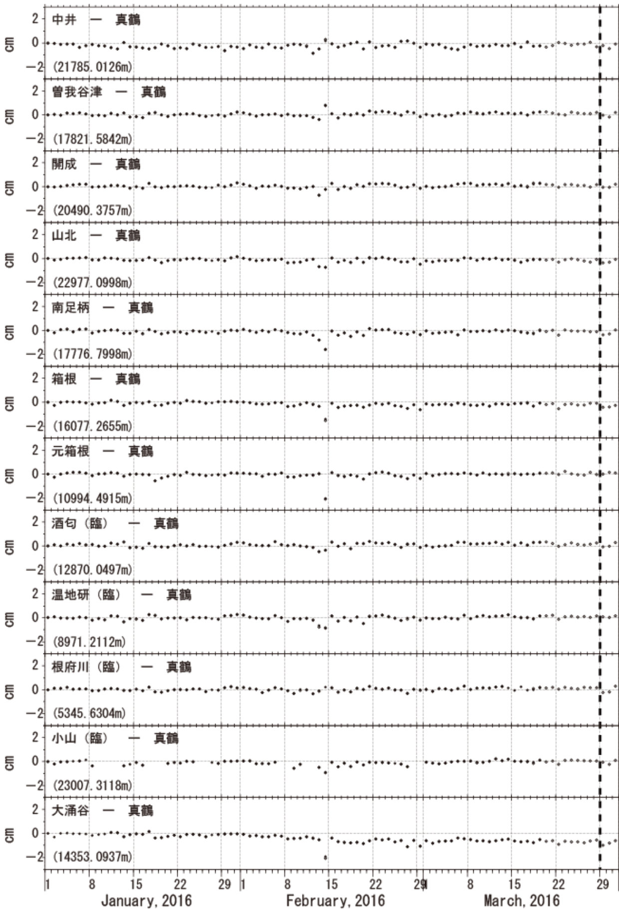
図4 GPS測量観測結果（2016年01月01日～2016年03月31日）
