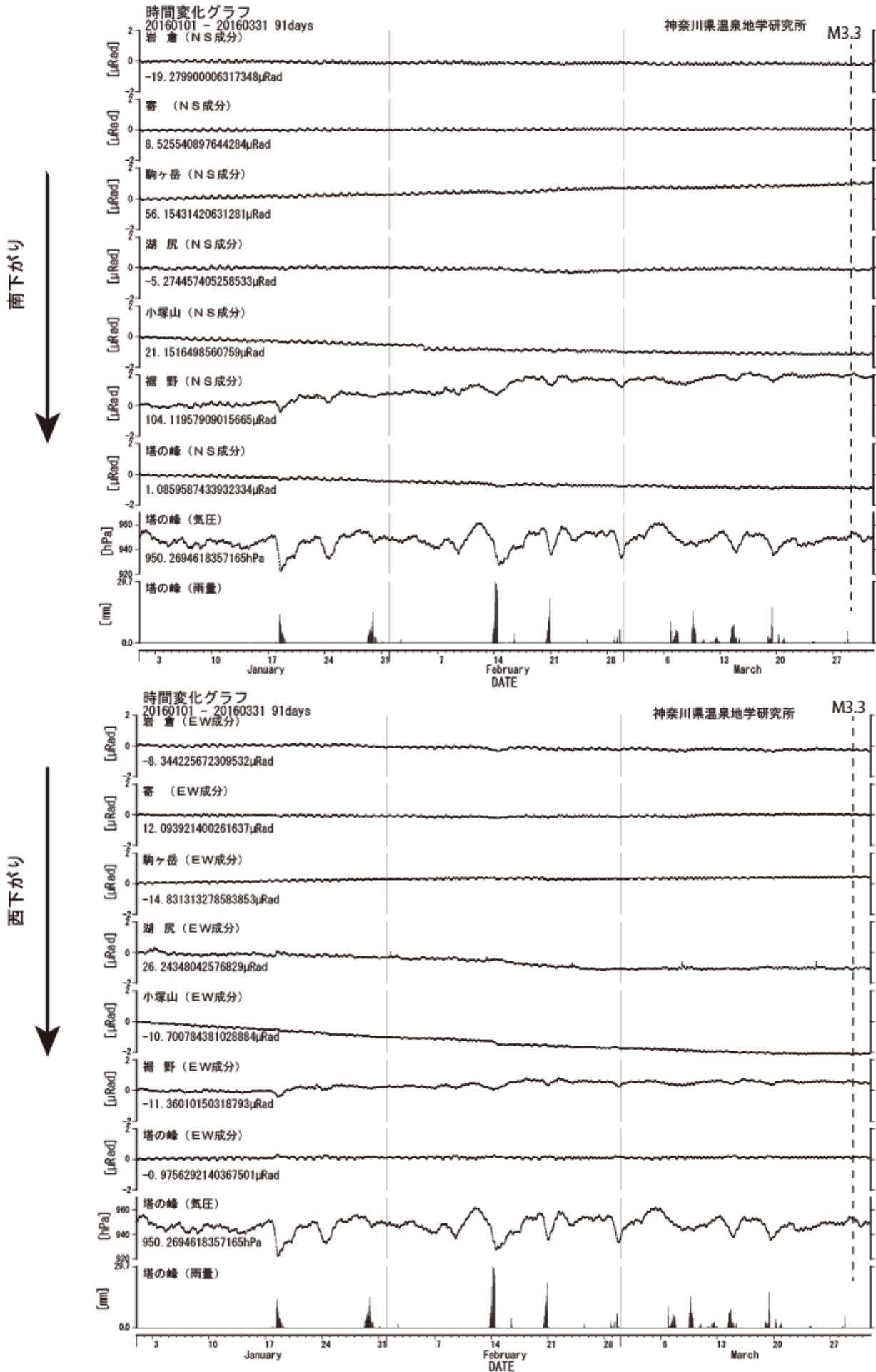
図3 傾斜計記録(2016年1月1日から2016年3月31日) 上:南北成分 下:東西成分
