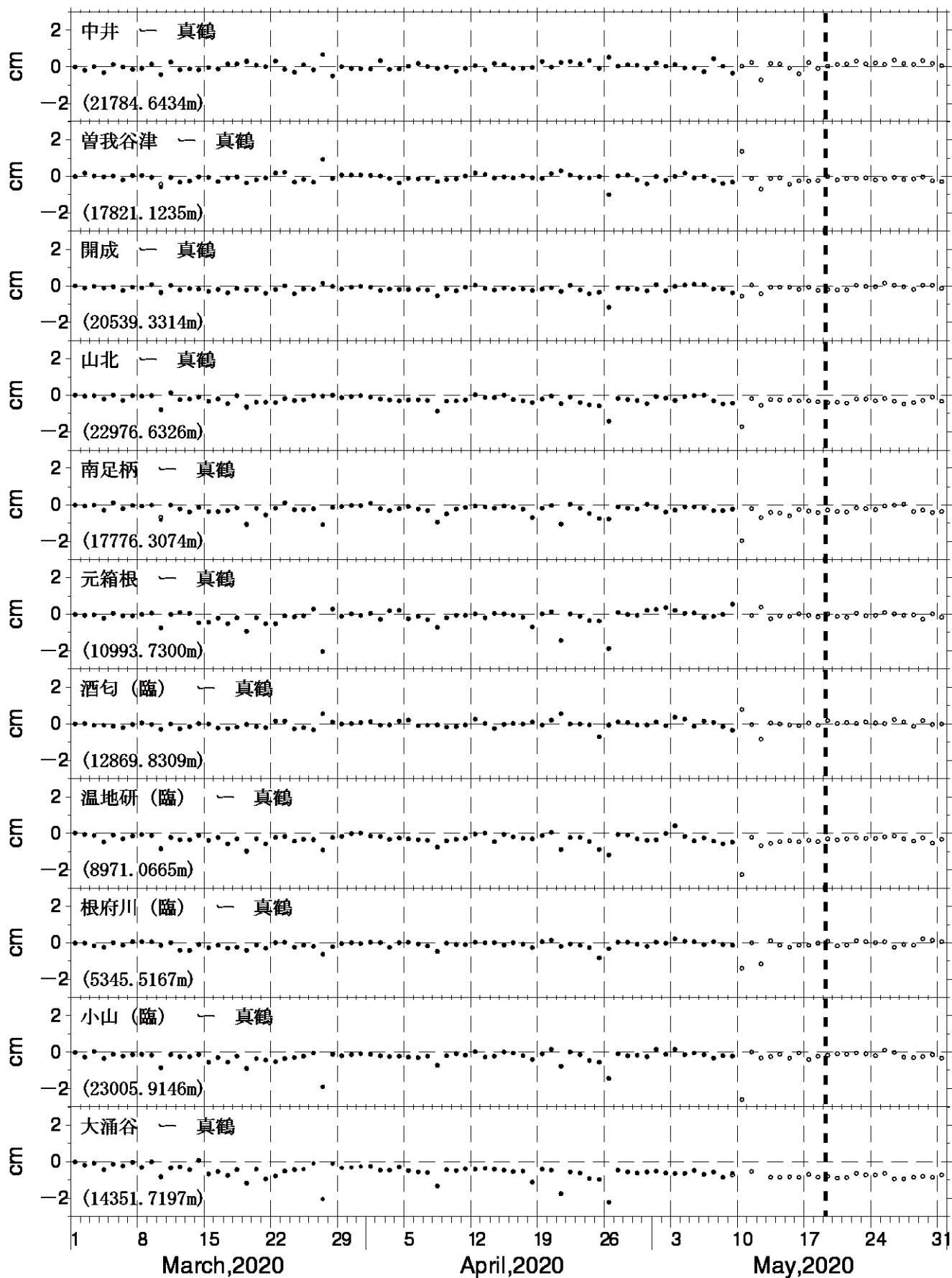
図4 GPS測量観測結果 (2020年03月01日~2020年05月31日) 真鶴観測点を中心とした、各観測点の基線長変化。●は精密暦、○は速報暦による解を示す。
