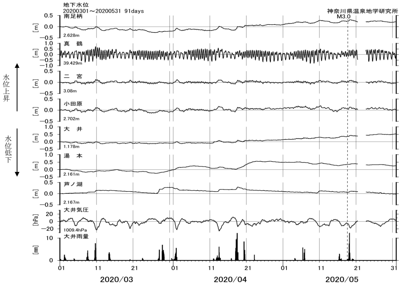
図6-1 地下水水位観測結果(2020年04月01日~2020年05月31日)
