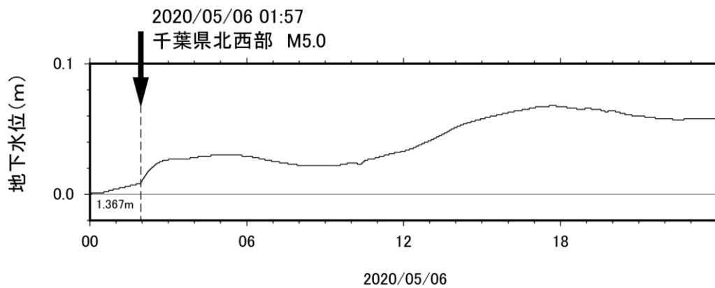
図6-2 地震にともなう地下水水位変化(2020年05月06日)
