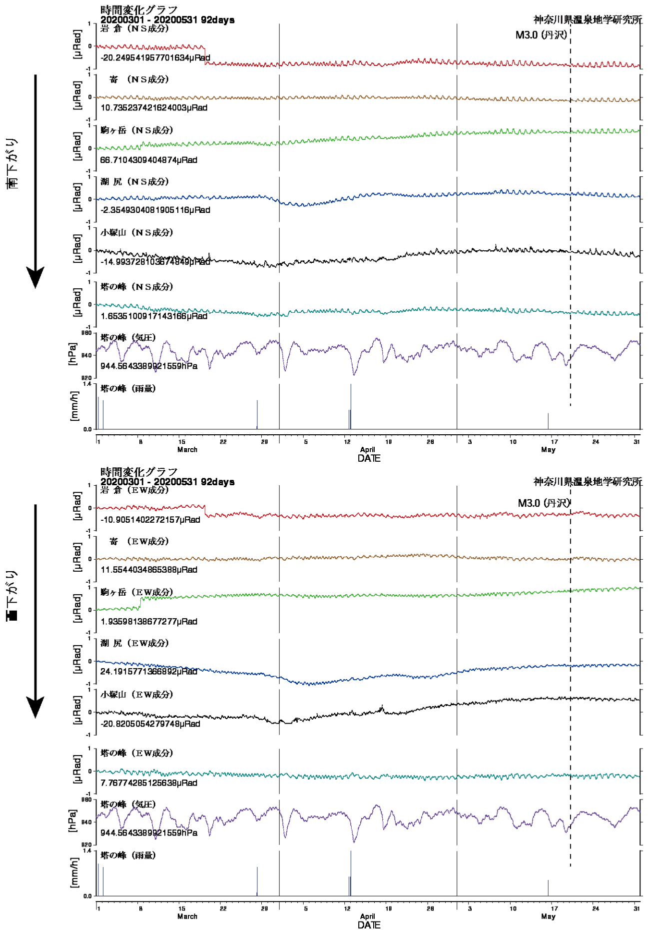
図3 傾斜計記録(2020年03月01日から2020年5月31日) 上:南北成分 下:東西成分 裾野観測点は、3月2日から機器更新のため欠測。
