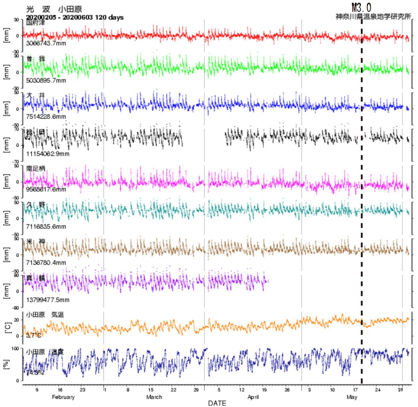
図5 光波測量（小田原観測網）観測結果（2020年02月05日～06月03日）
