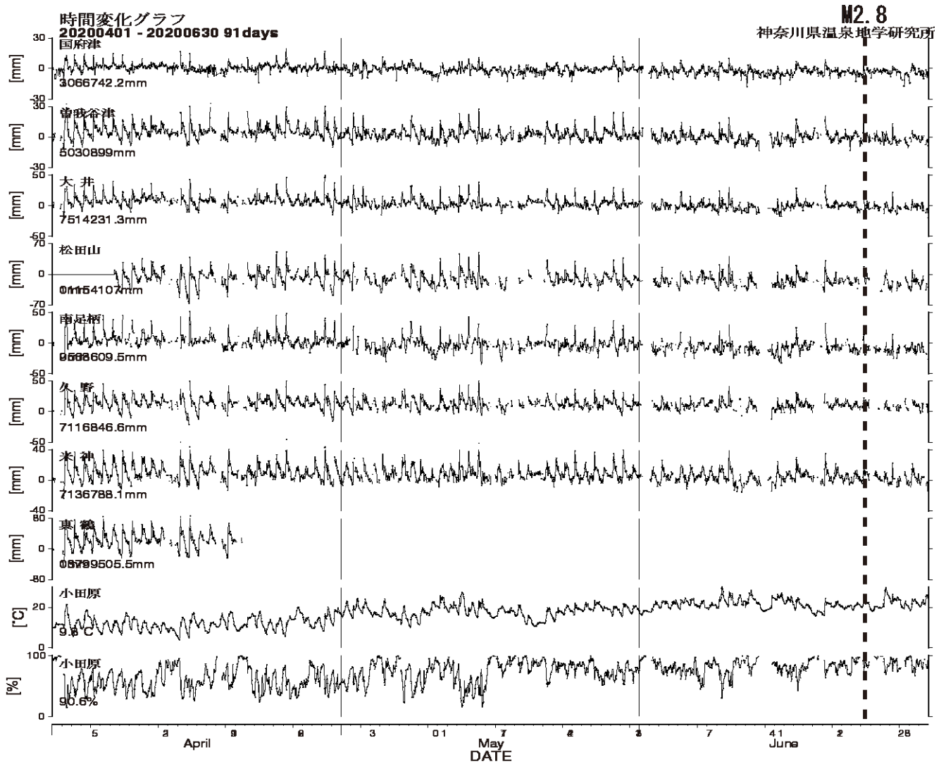
図5 光波測量（小田原観測網）観測結果（2020年04月01日～06月30日）
