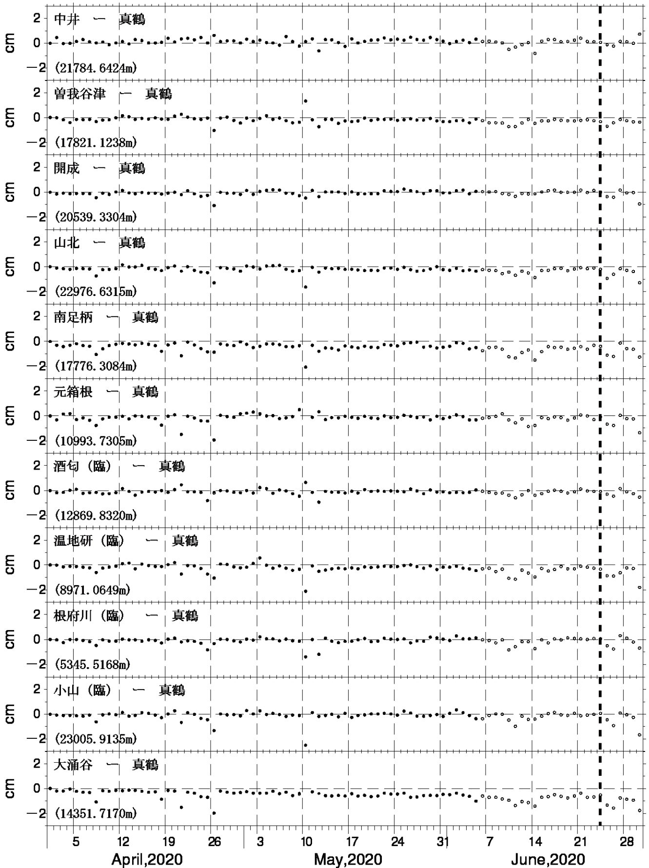
図4 GNSS測量観測結果 (2020年04月01日~2020年06月30日) 真鶴観測点を中心とした、各観測点の基線長変化。●は精密暦、○は速報暦による解を示す。
