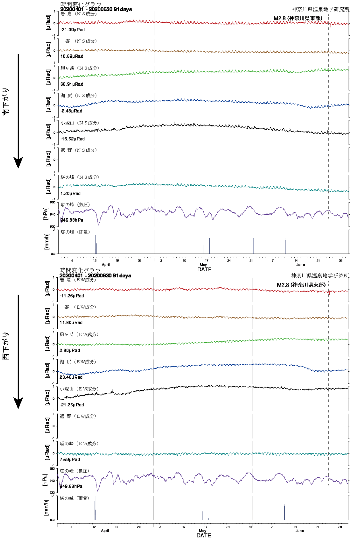
図3 傾斜計記録(2020年04月01日から2020年6月30日) 上:南北成分 下:東西成分 裾野観測点は、3月2日から機器更新のため欠測。
