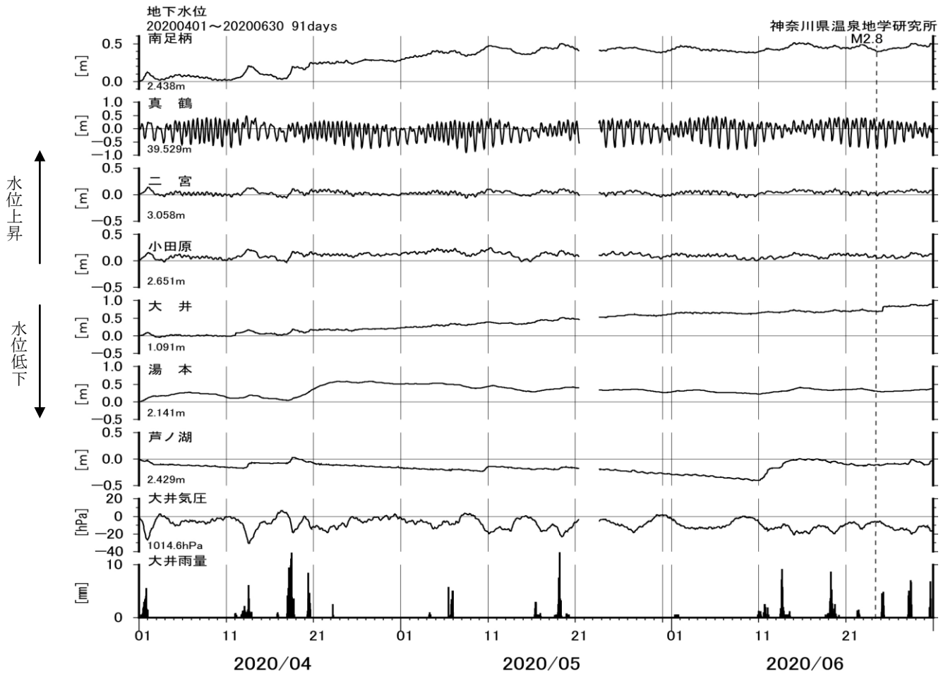
図6-1 地下水位観測結果(2020年04月01日~2020年06月30日)
