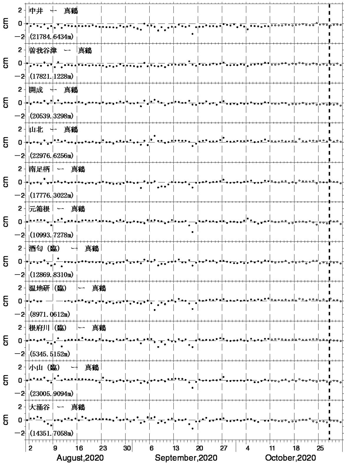
図4 GNSS測量観測結果(2020年08月01日~2020年10月31日) 真鶴観測点を中心とした、各観測点の基線長変化。●は精密暦、○は速報暦による解を示す。
