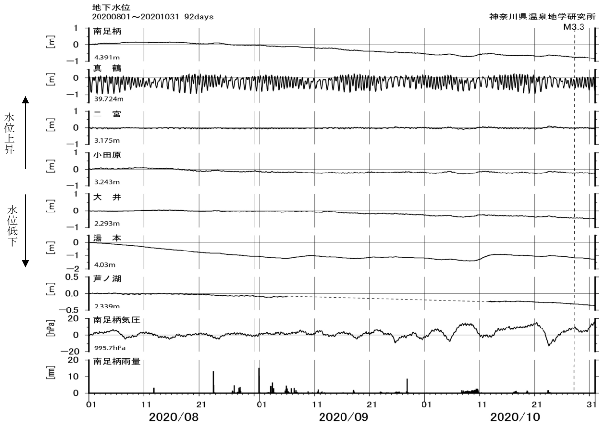
図6 地下水位観測結果(2020年08月01日～2020年10月31日)
