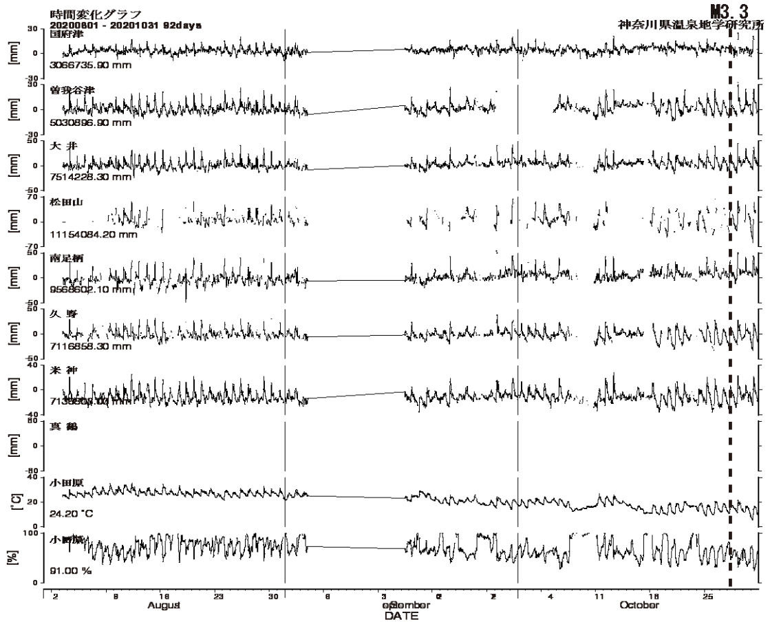
図5 光波測量（小田原観測網）観測結果（2020年08月01日～10月31日） 真鶴基線は欠測
