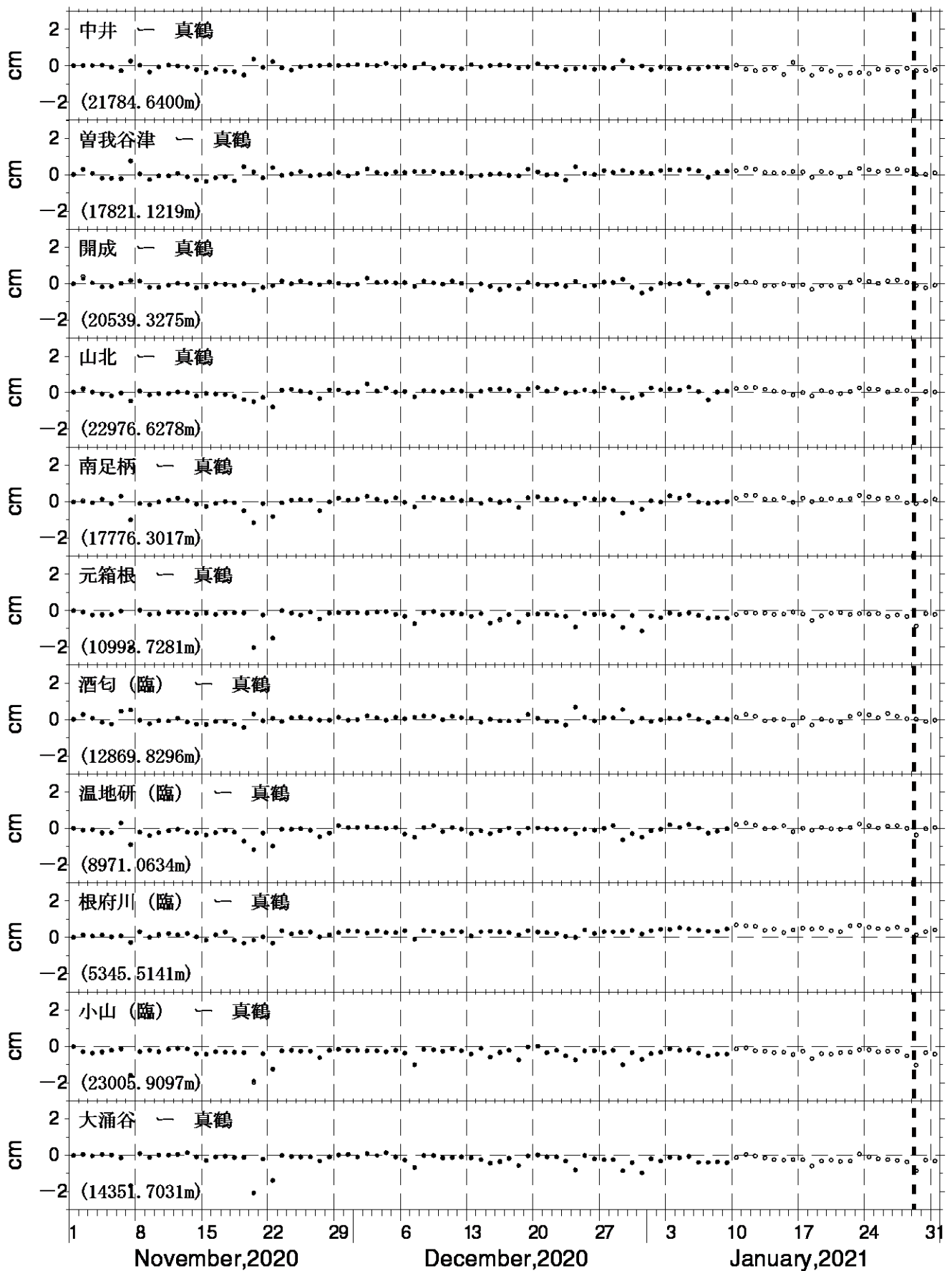
図4 GNSS測量観測結果 (2020年11月01日～2021年01月31日)
