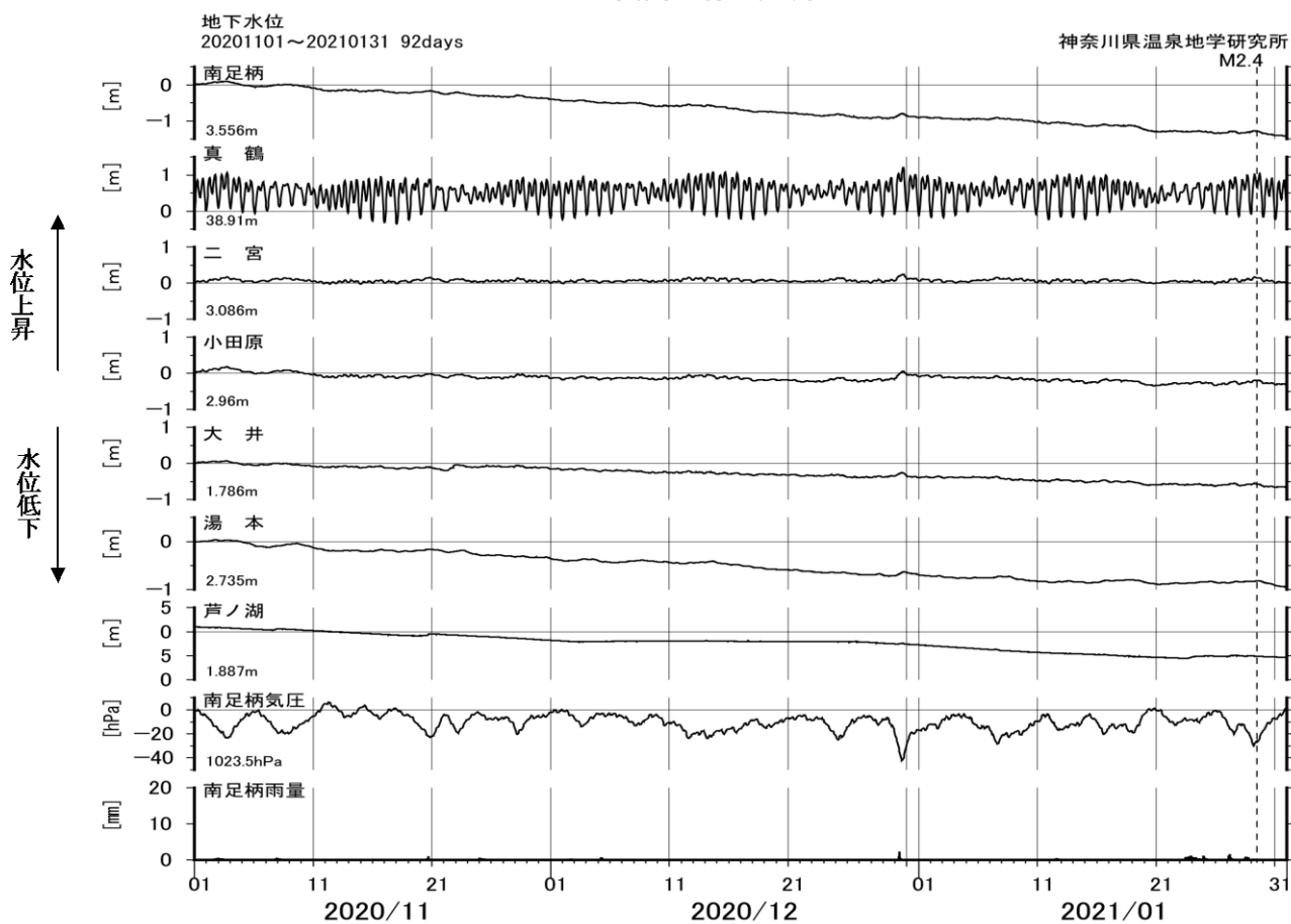
図6 地下水位観測結果（2020年11月01日～2021年1月31日）
