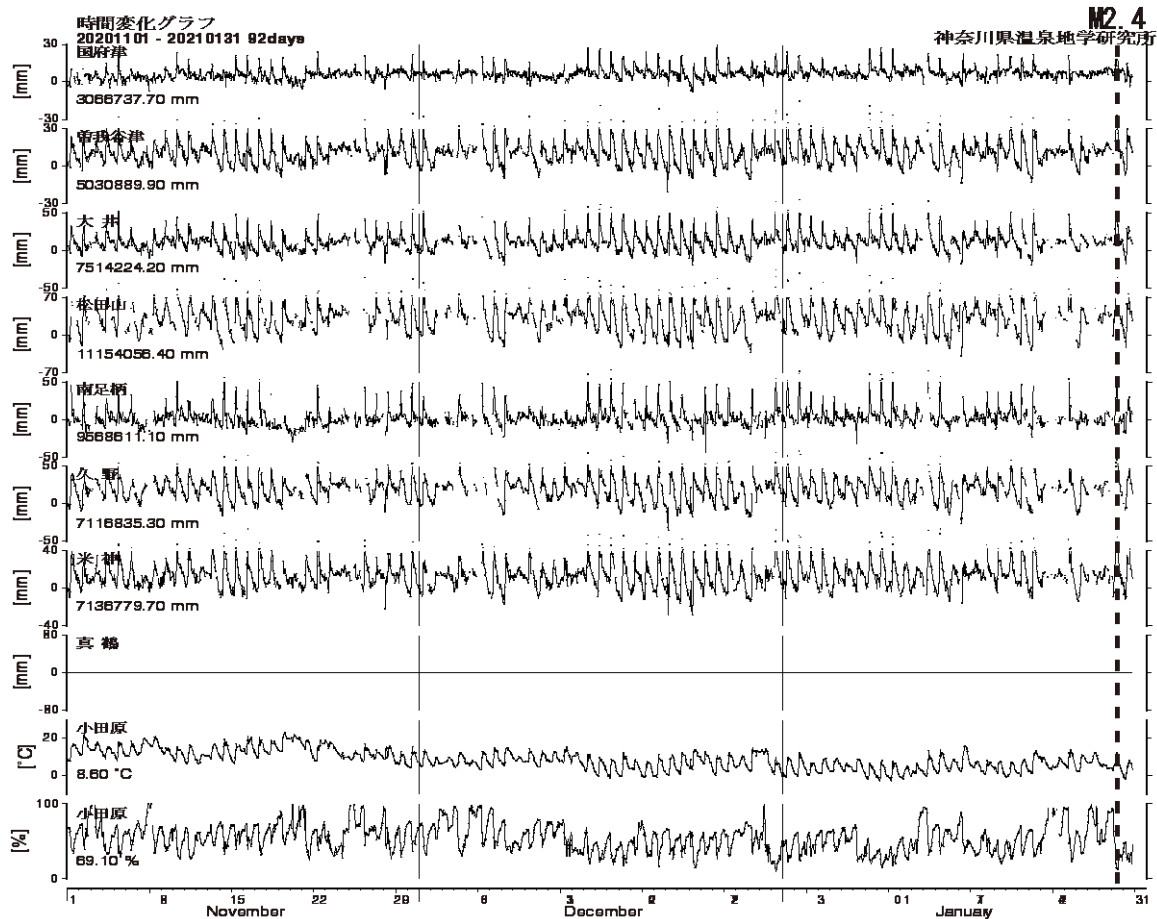
図5 光波測量（小田原観測網）観測結果（2020年11月01日～2021年01月31日） 真鶴基線は欠測
