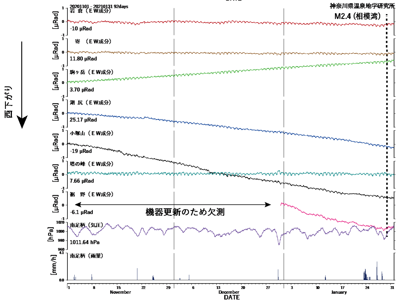
図3 傾斜計記録 (2020年11月01日から2021年01月31日)
