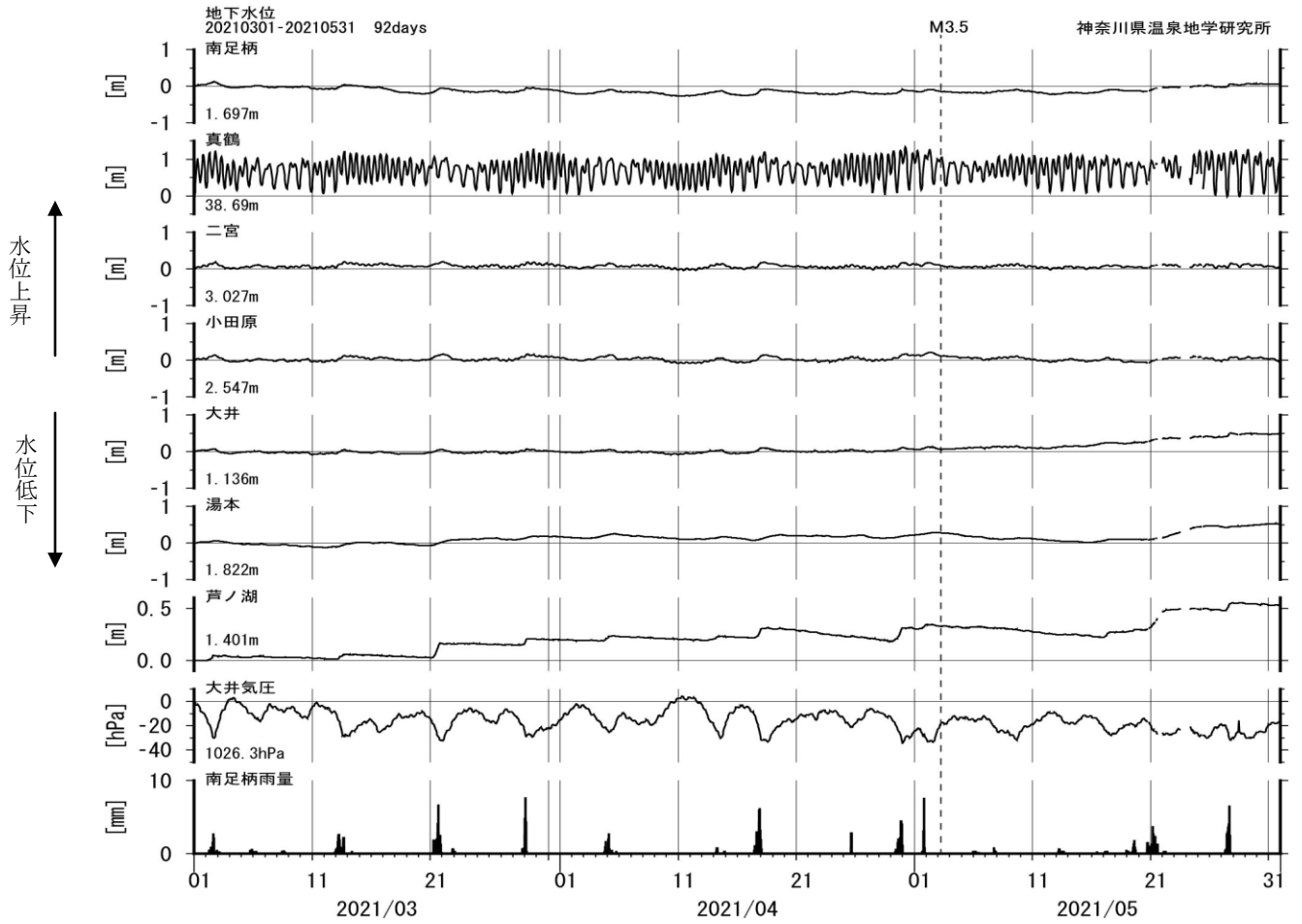
図6-1 地下水水位観測結果(2021年03月01日~2021年05月31日)
