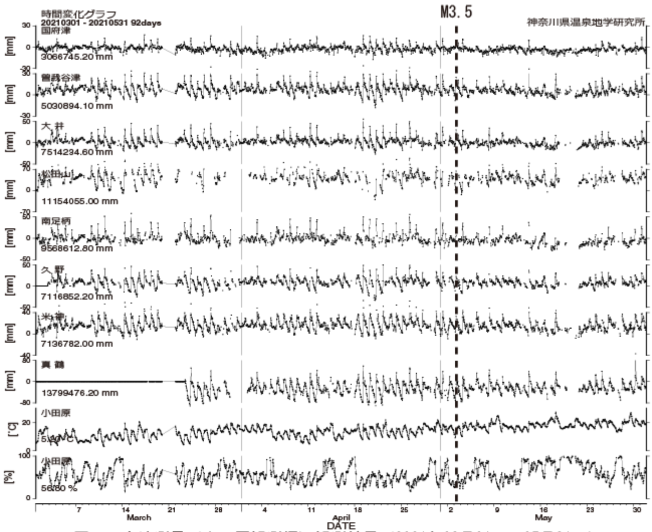
図5 光波測量（小田原観測網）観測結果（2021年03月01日～05月31日）
