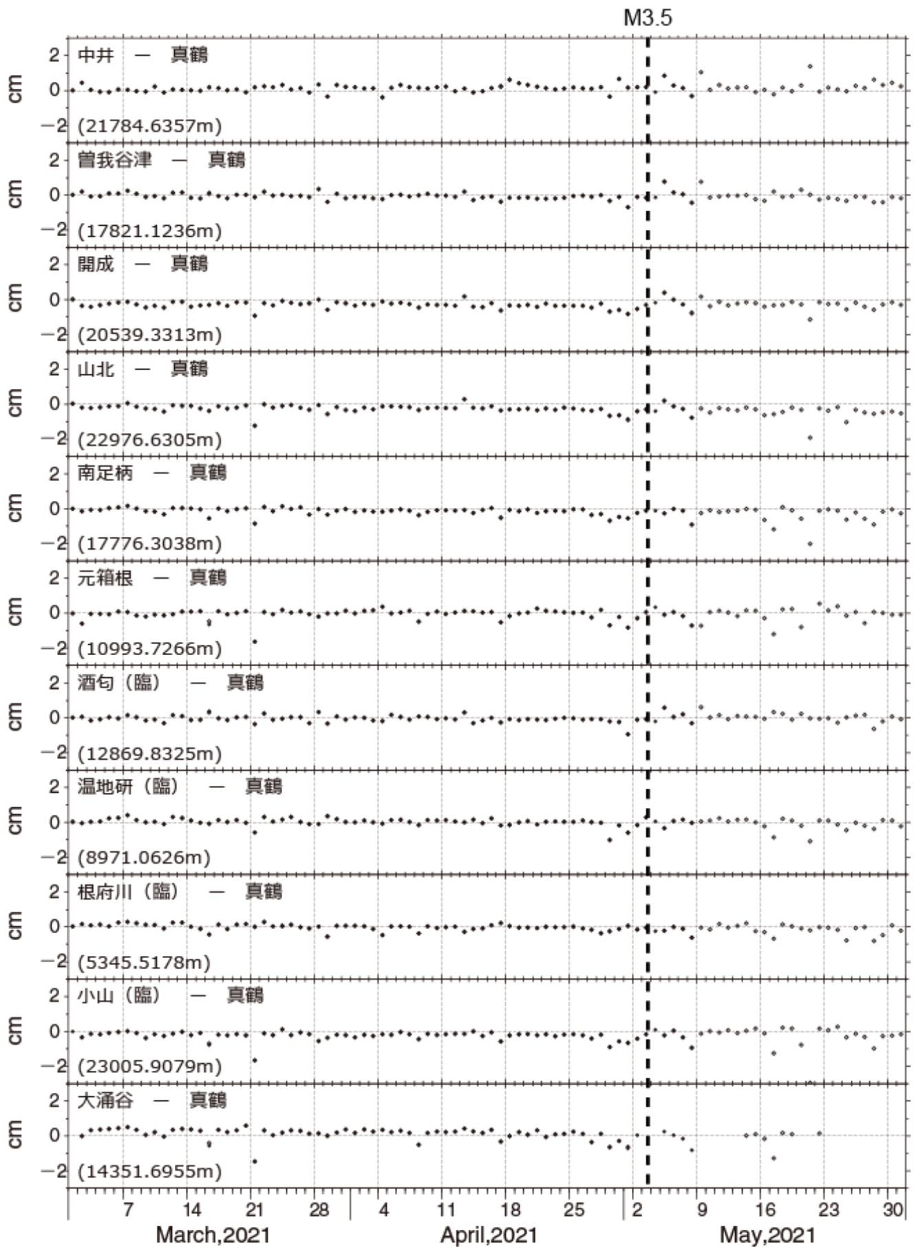
図4 GNSS測量観測結果 (2021年03月01日~2021年05月31日) 真鶴観測点を中心とした、各観測点の基線長変化。 ●は精密層、○は速報層による解を示す。
