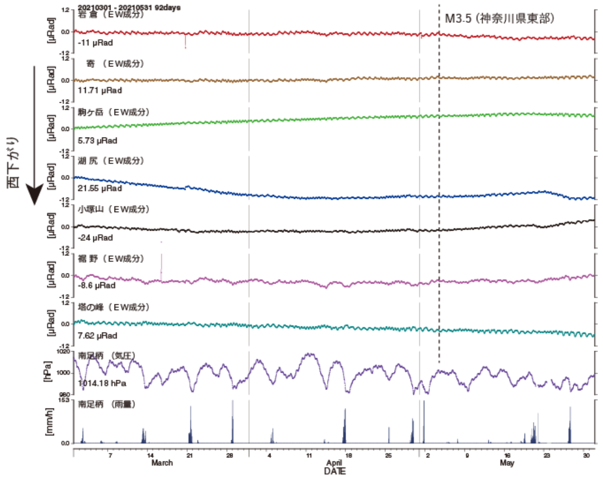
図3 傾斜計記録 (2021年03月01日から2021年05月31日) 3月20日18時09分 (宮城県沖) の地震によるステップは補正済み。
