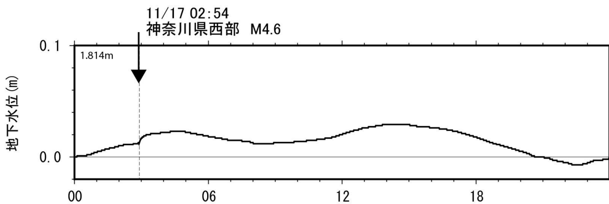
図6-2 地震にともなう地下水水位変化(大井観測井 2021年11月17日)
