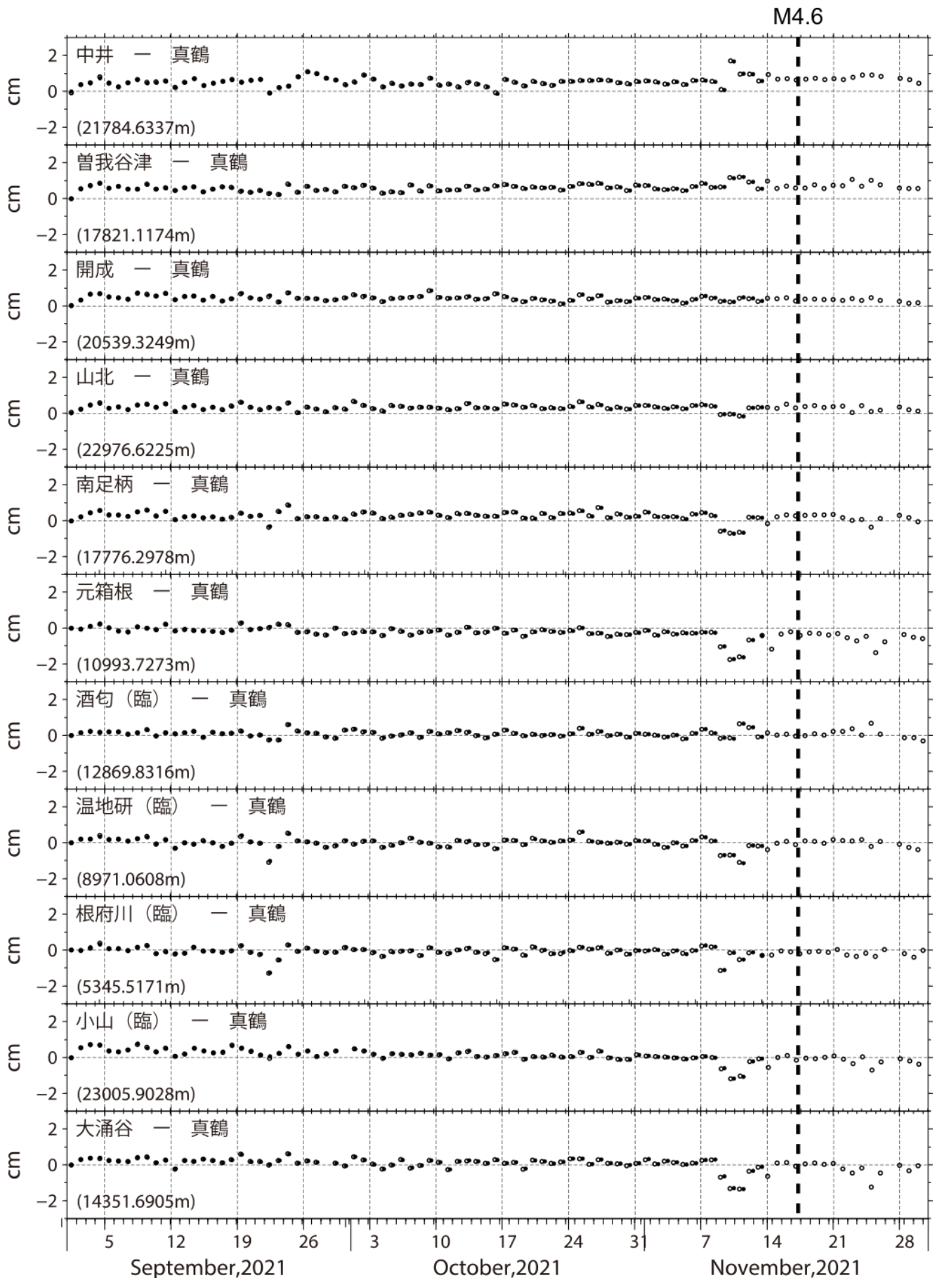
図4 GNSS測量観測結果（2021年09月01日～2021年11月30日）
