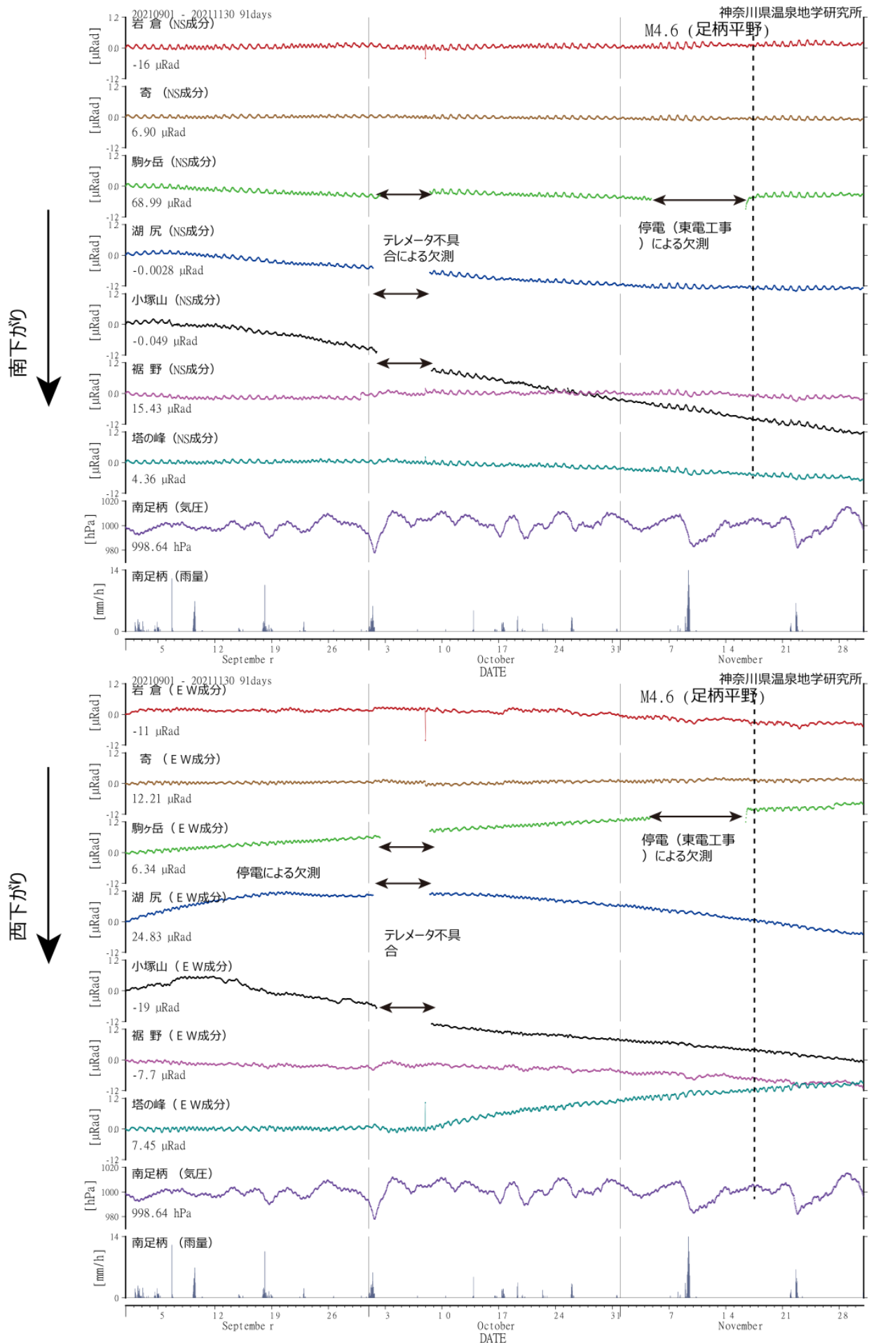
図3 傾斜計記録 (2021年09月01日から2021年11月30日)
