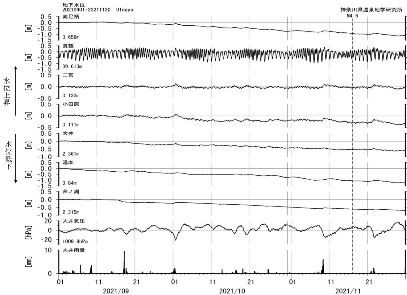
図6-1 地下水水位観測結果(2021年09月01日~2021年11月30日)
