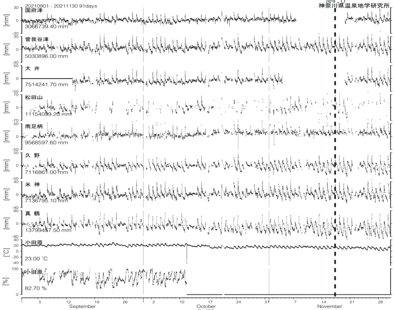
図5 光波測量 (小田原観測網) 観測結果 (2021年09月01日~11月30日)
