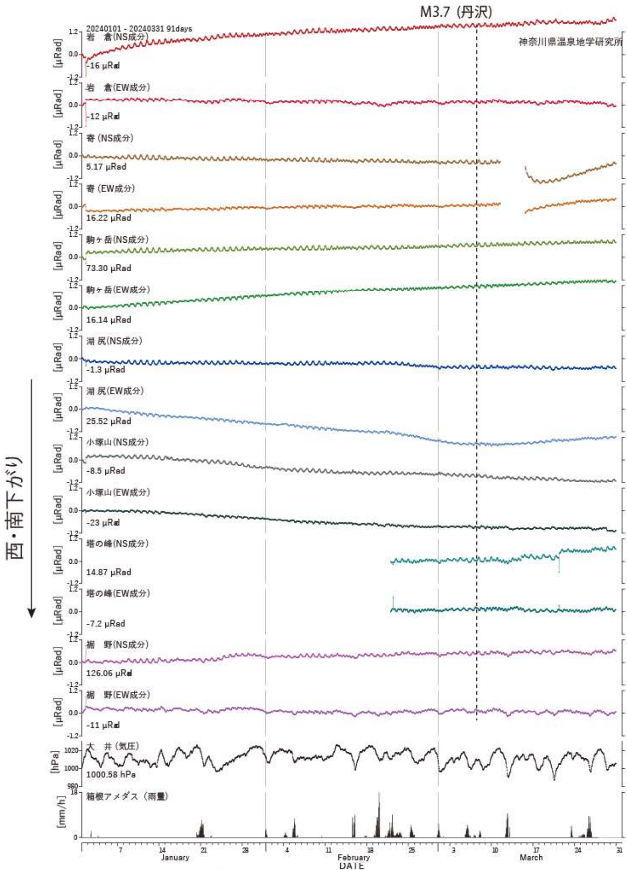
図3 傾斜計記録 (2024年01月01日から2024年03月31日) 寄観測点は3月15-18日にセンサーの入れ替え工事を実施。 塔の峰観測点は8月下旬以降地上制御装置故障のため欠測。2月22日より復旧。
