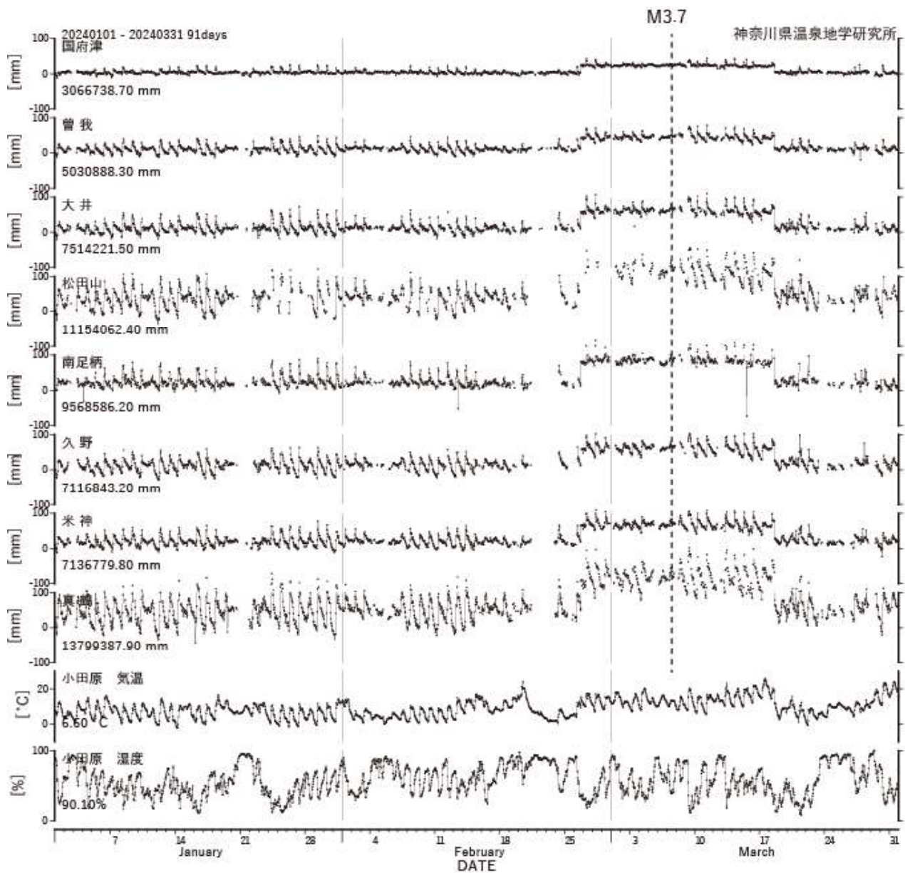
図5 光波測量(小田原観測網)観測結果(2024年01月01日~2024年03月31日) 2月26日・3月18日に全点にステップ状の変動が見られる。 原因は特定できていないが、地殻変動を捉えたものではない。
