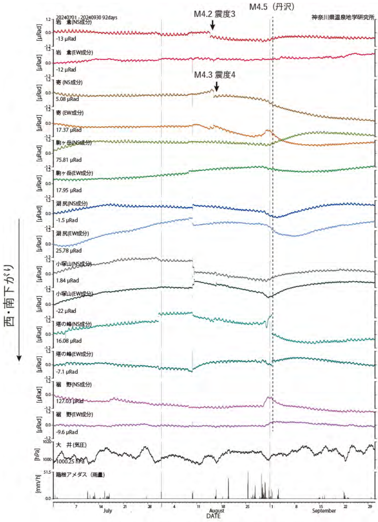
図3 傾斜計記録 (2024年07月01日から2024年09月30日)
