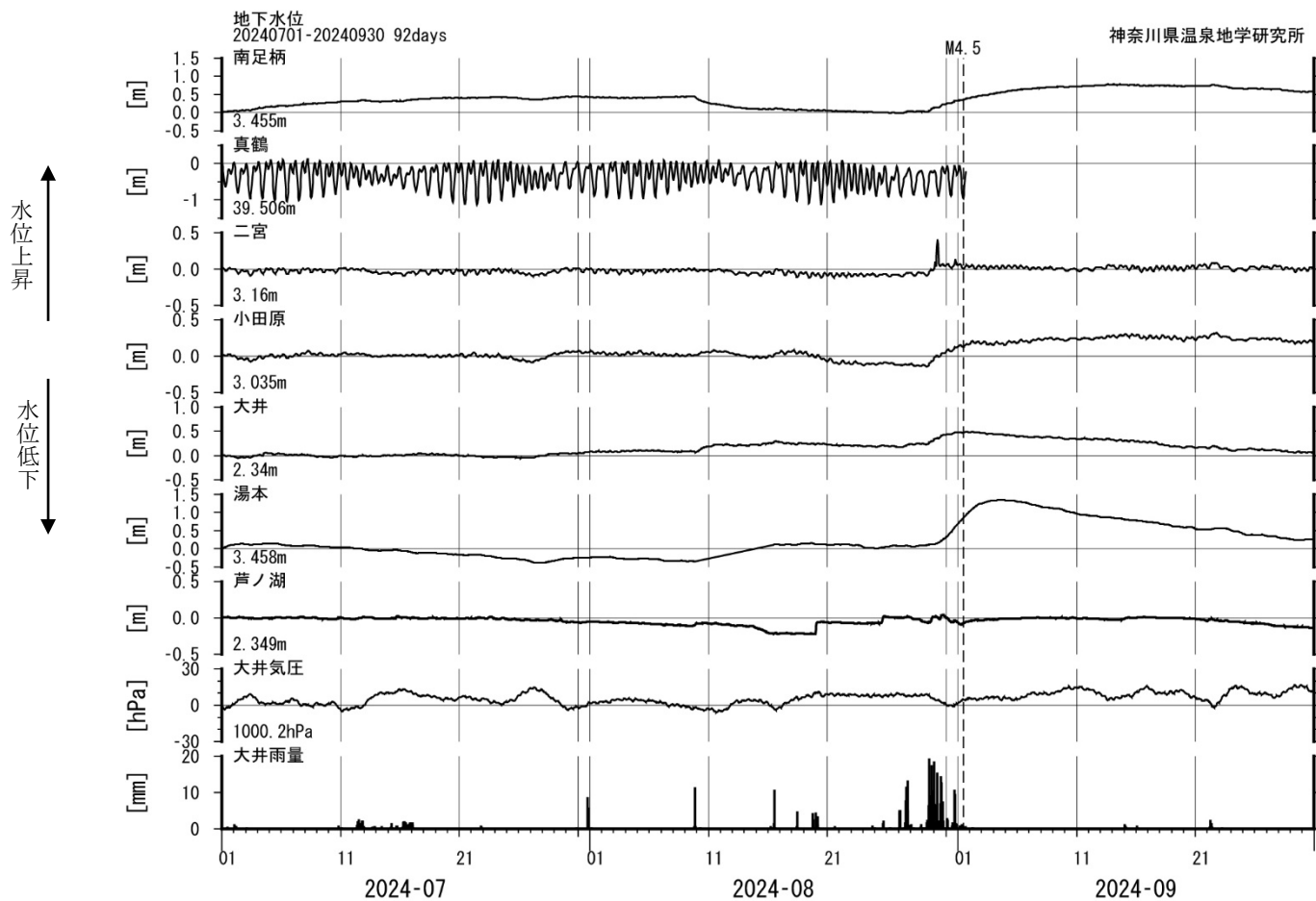
図6 地下水位観測結果(2024年07月01日~2024年09月30日)
