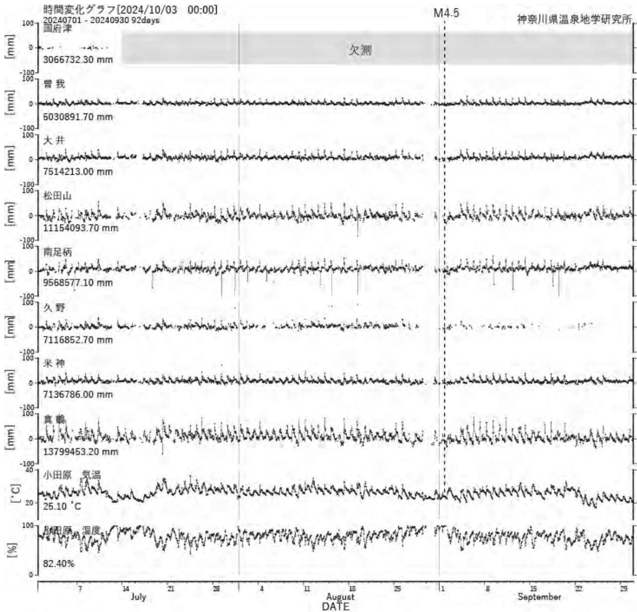
図5 光波測量(小田原観測網)観測結果(2024年07月01日～2024年09月30日)
