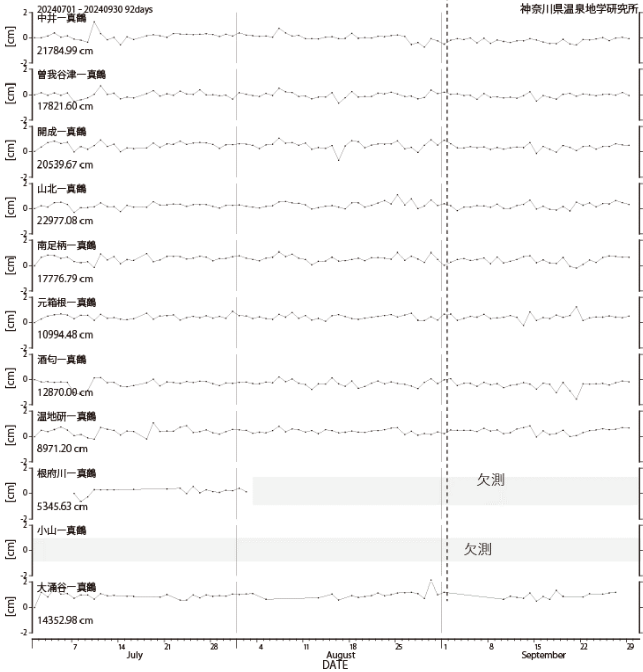
図4 GNSS測量観測結果(2024年07月01日～2024年09月30日) 真鶴観測点を基準とした、各観測点の基線長変化。 根府川・小山は通信に不具合のため一部欠測。
