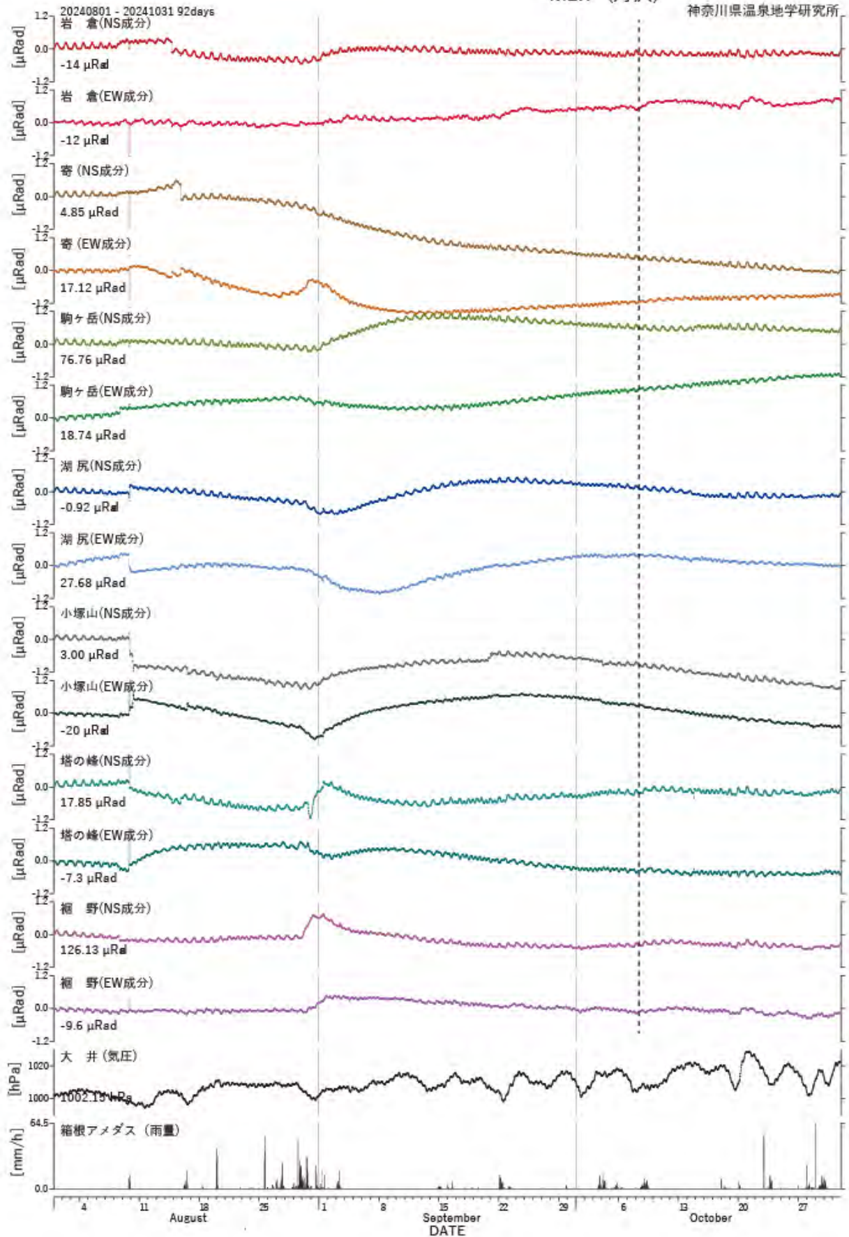
図3 傾斜計記録(2024年08月01日から2024年10月31日)
