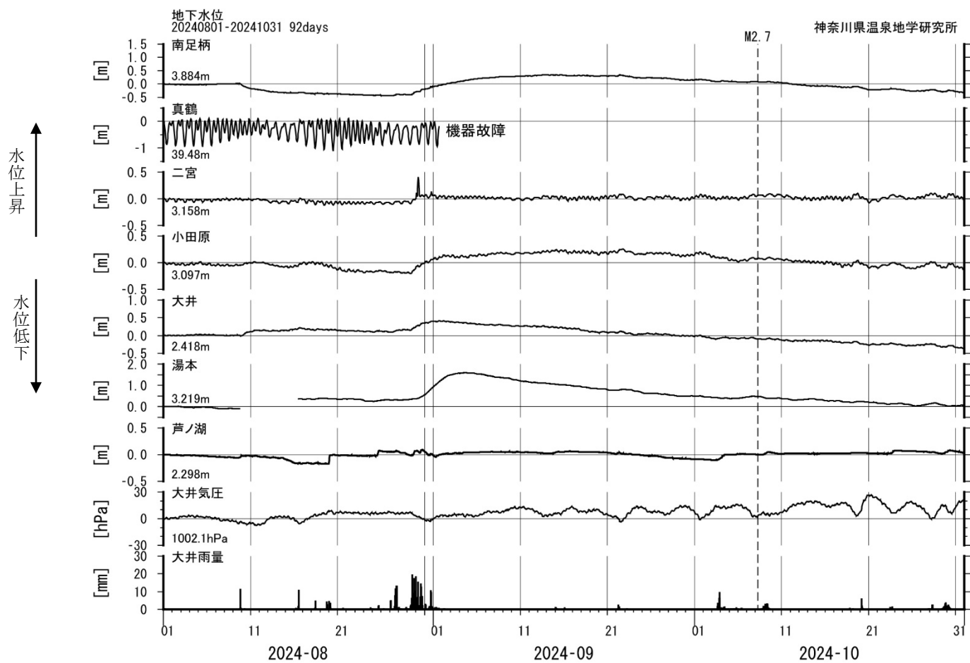
図6 地下水位観測結果(2024年08月01日～2024年10月31日)
