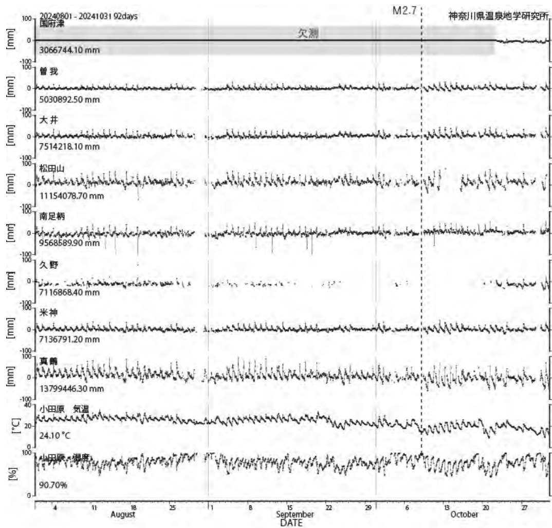
図5 光波測量(小田原観測網)観測結果(2024年08月01日～2024年10月31日)
