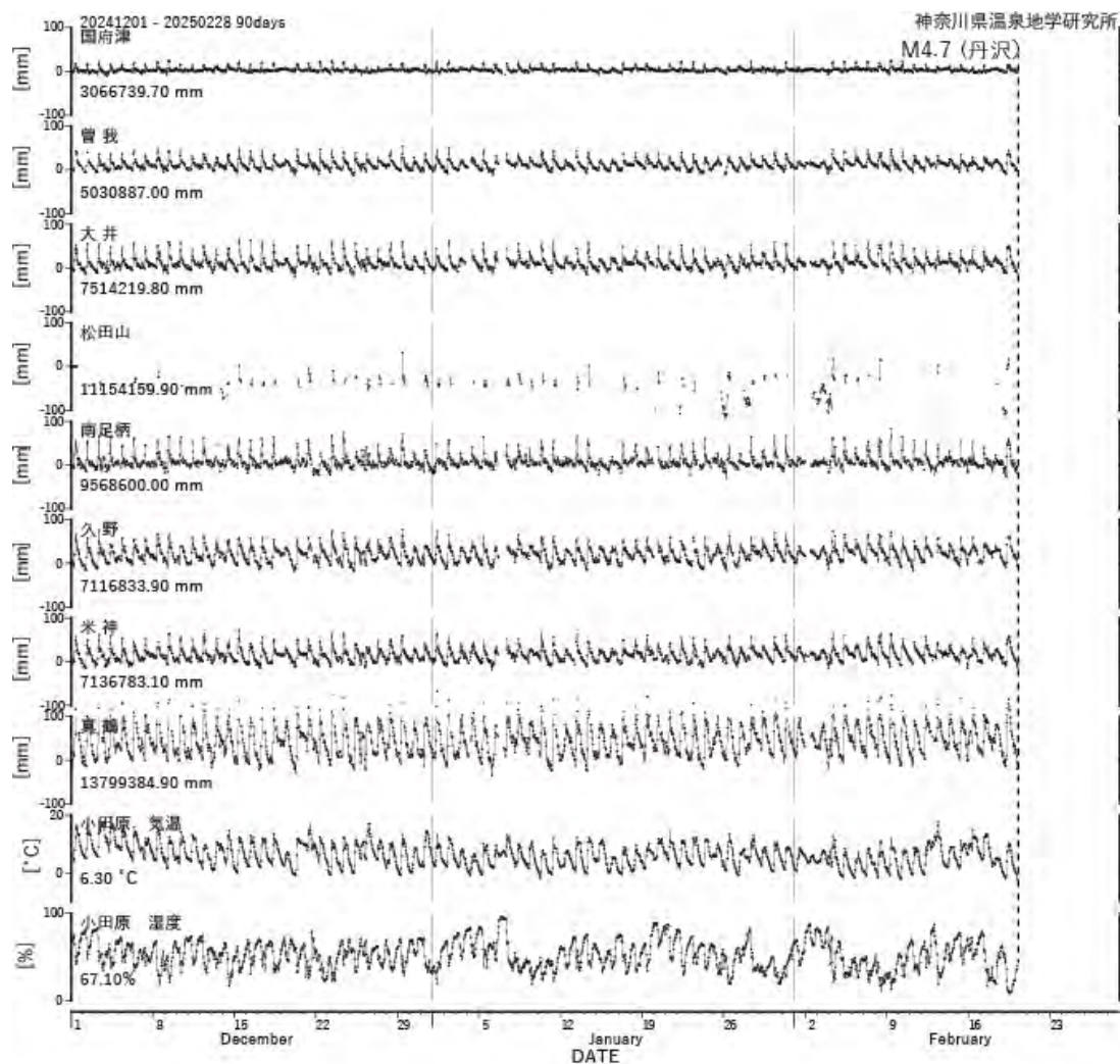
図5 光波測量(小田原観測網)観測結果(2024年12月01日～2025年02月28日) 2025年2月20日以降は欠測。
