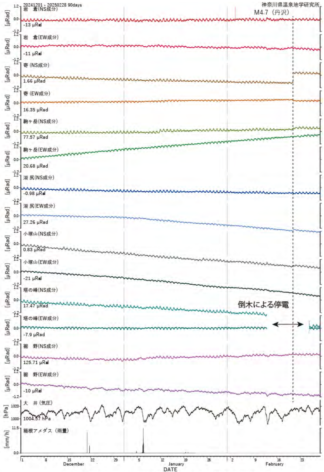
図3 傾斜計記録 (2024年12月01日から2025年02月28日)
