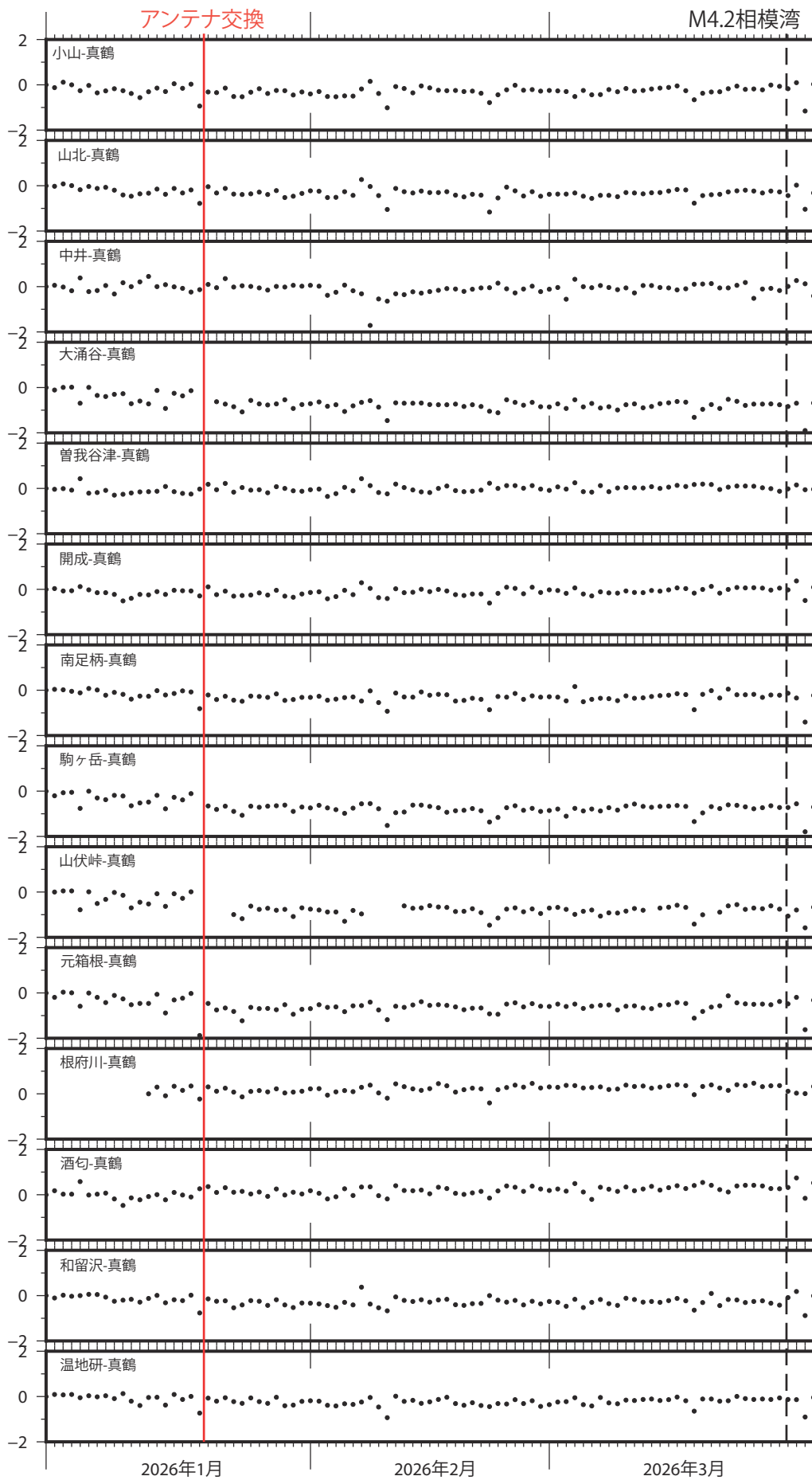
図4 GNSS測量観測結果(2026年1月1日~2026年3月31日) 真鶴観測点を基準とした、各観測点の基線長変化。
