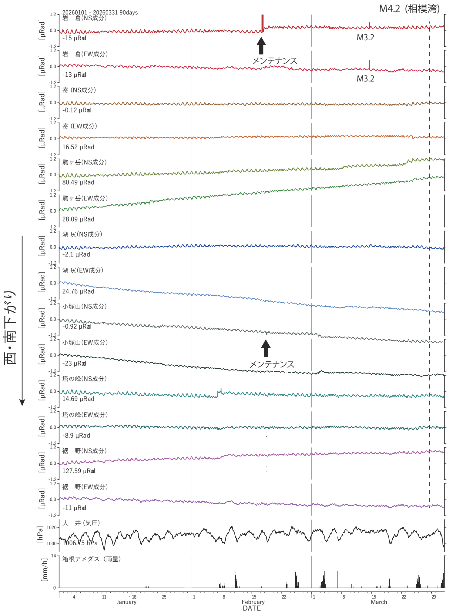
図3 傾斜計記録 (2026年01月01日から2026年03月31日)
