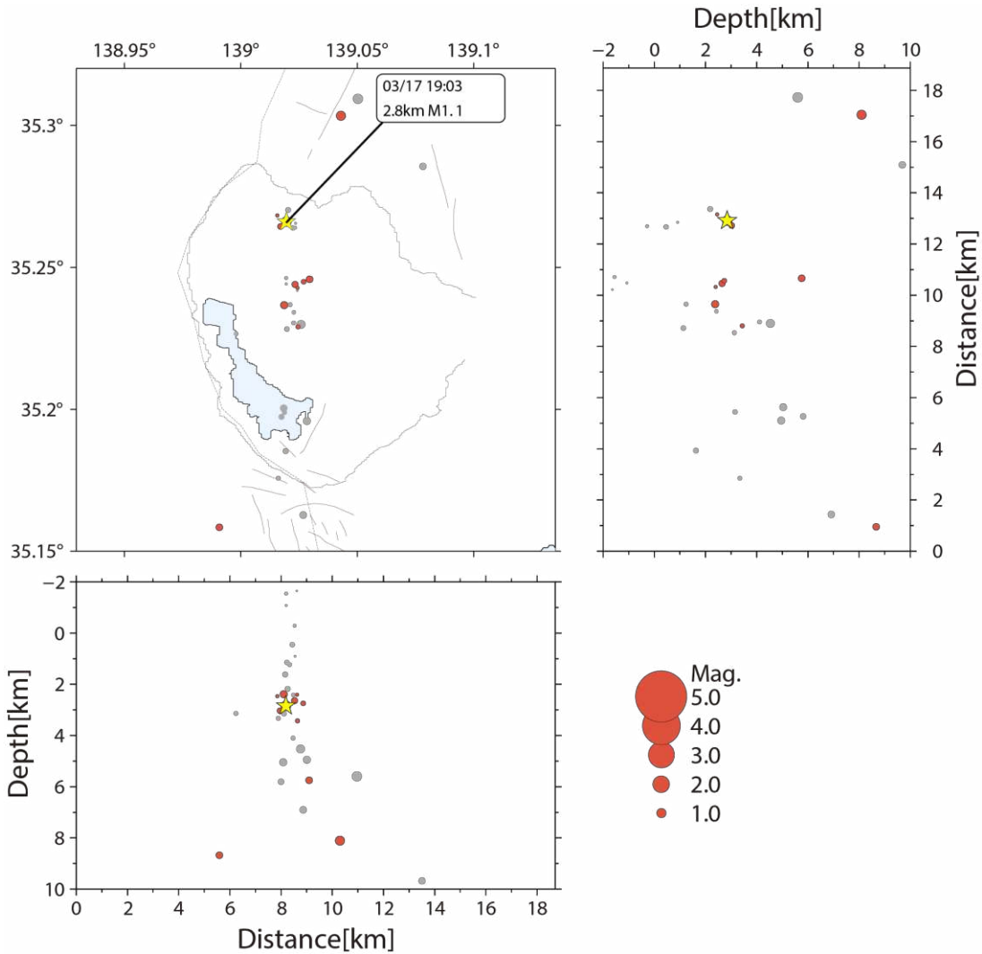
図 1-2 箱根火山の今月の地震活動。赤の丸印で 2026 年 3 月に発生した地震の震源を示しております。灰色の丸印で 2026 年 1 月と 2 月に発生した地震の震源を示しております。丸印の大きさはマグニチュードに対応します。星印で 2026 年 3 月に図の領域で発生した最大規模の地震の震源を示しております。（震源決定は、当所データの他に東京大学地震研究所、防災科学技術研究所および気象庁の地震波形データを利用しています。）
