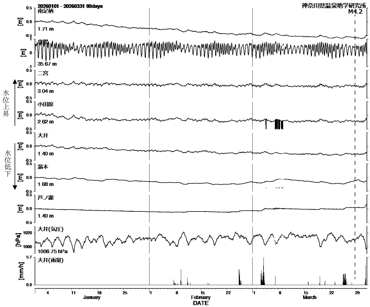
図5 地下水位観測結果(2026年01月01日~03月31日)
