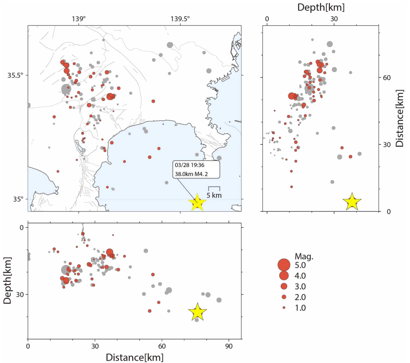
図 1-1 神奈川県とその周辺地域の今月の地震活動。赤の丸印で 2026 年 3 月に発生した地震の震源を示しております。灰色の丸印で 2026 年 1 月と 2 月に発生した地震の震源を示しております。丸印の大きさはマグニチュードに対応します。星印で 2026 年 3 月に図の領域で発生した最大規模の地震の震源を示しております。（震源決定は、当所データの他に東京大学地震研究所、防災科学技術研究所および気象庁の地震波形データを利用しています。）
