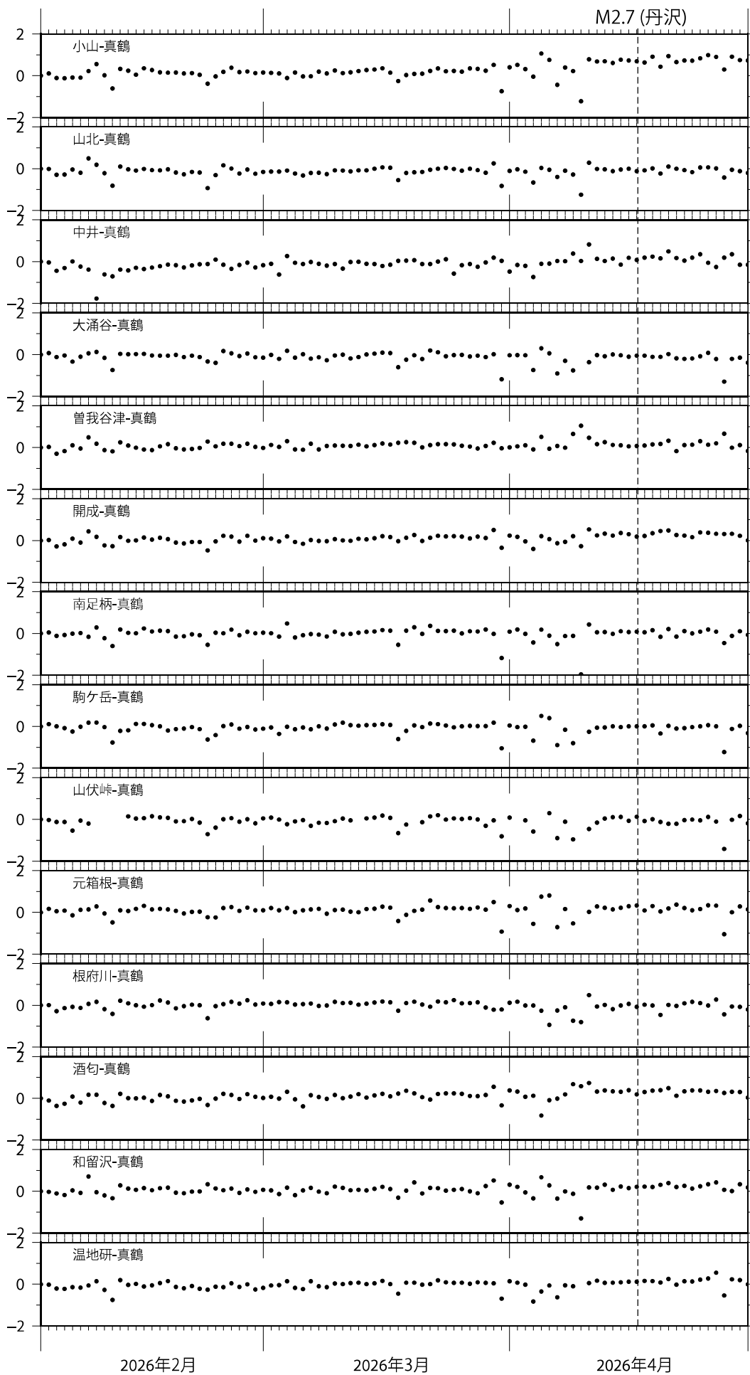
図4 GNSS測量観測結果(2026年2月1日~2026年4月30日) 真鶴観測点を基準とした、各観測点の基線長変化。
