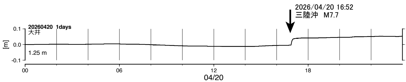
図 5 - 2 コサイスマミックな水位の変化 (2026年04月20日、大井観測点)
