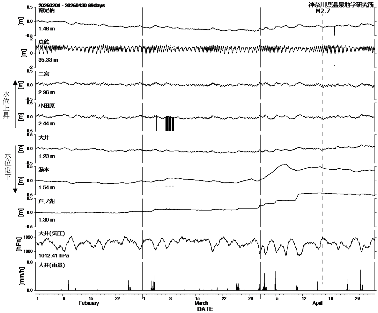
図 5 - 1 地下水位観測結果 (2026年02月01日~04月30日)
