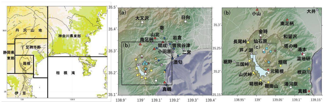
図 2-1 表 1 に対応する地域区分 (深はさ 50 km まで)
