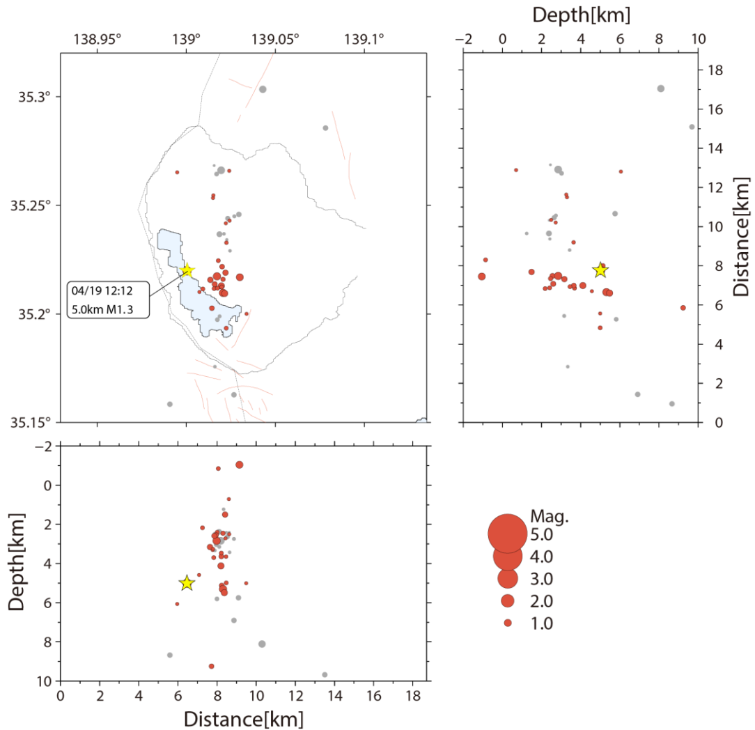
図 1-2 箱根火山の今月の地震活動。赤の丸印で 2026 年 4 月に発生した地震の震源を示しております。灰色の丸印で 2026 年 2 月と 3 月に発生した地震の震源を示しております。丸印の大きさはマグニチュードに対応します。星印で 2026 年 4 月に図の領域で発生した最大規模の地震の震源を示しております。(震源決定は、当所データの他に東京大学地震研究所、防災科学技術研究所および気象庁の地震波形データを利用しています。)
