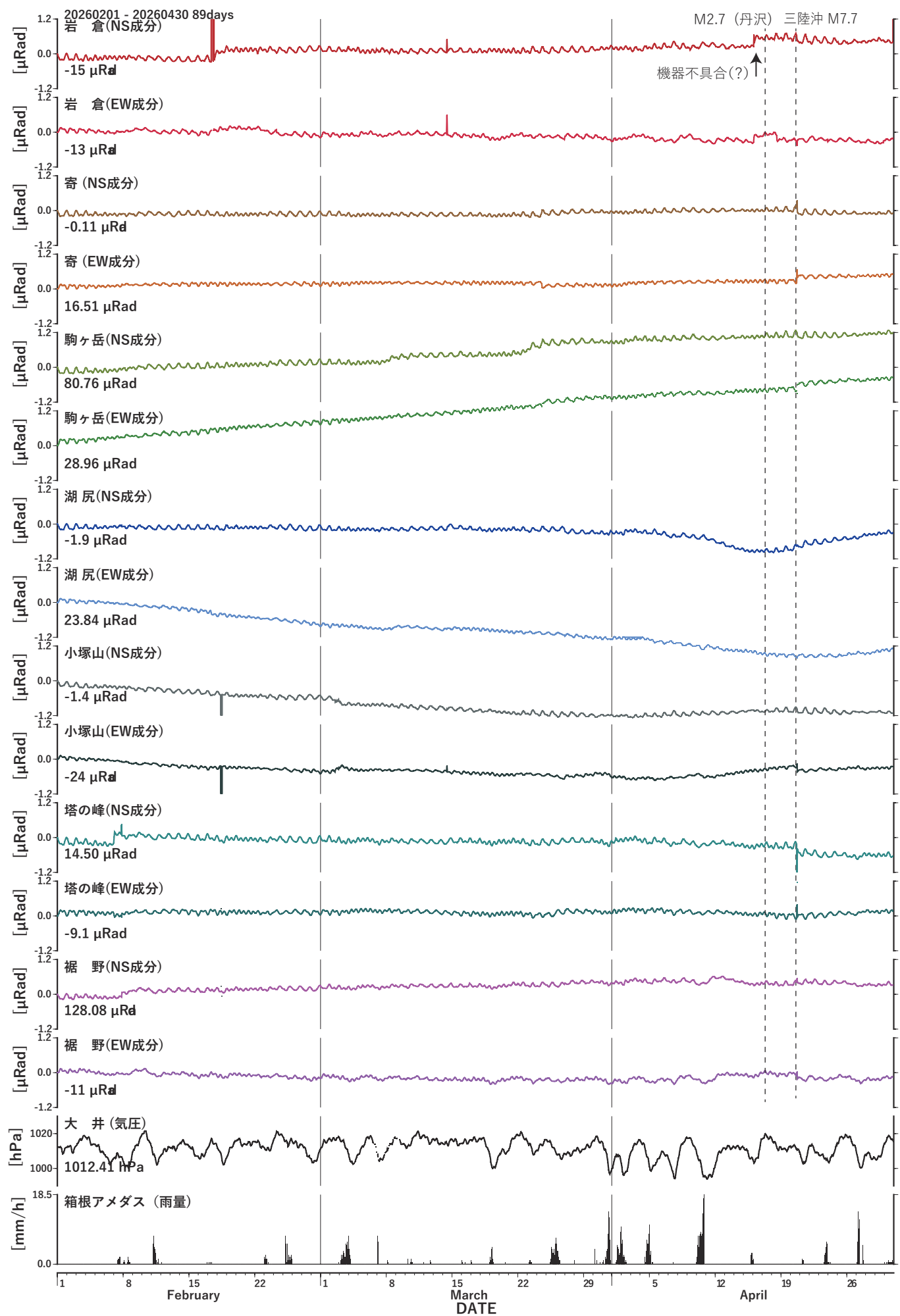
図3 傾斜計記録(2026年02月01日から2026年04月30日)
