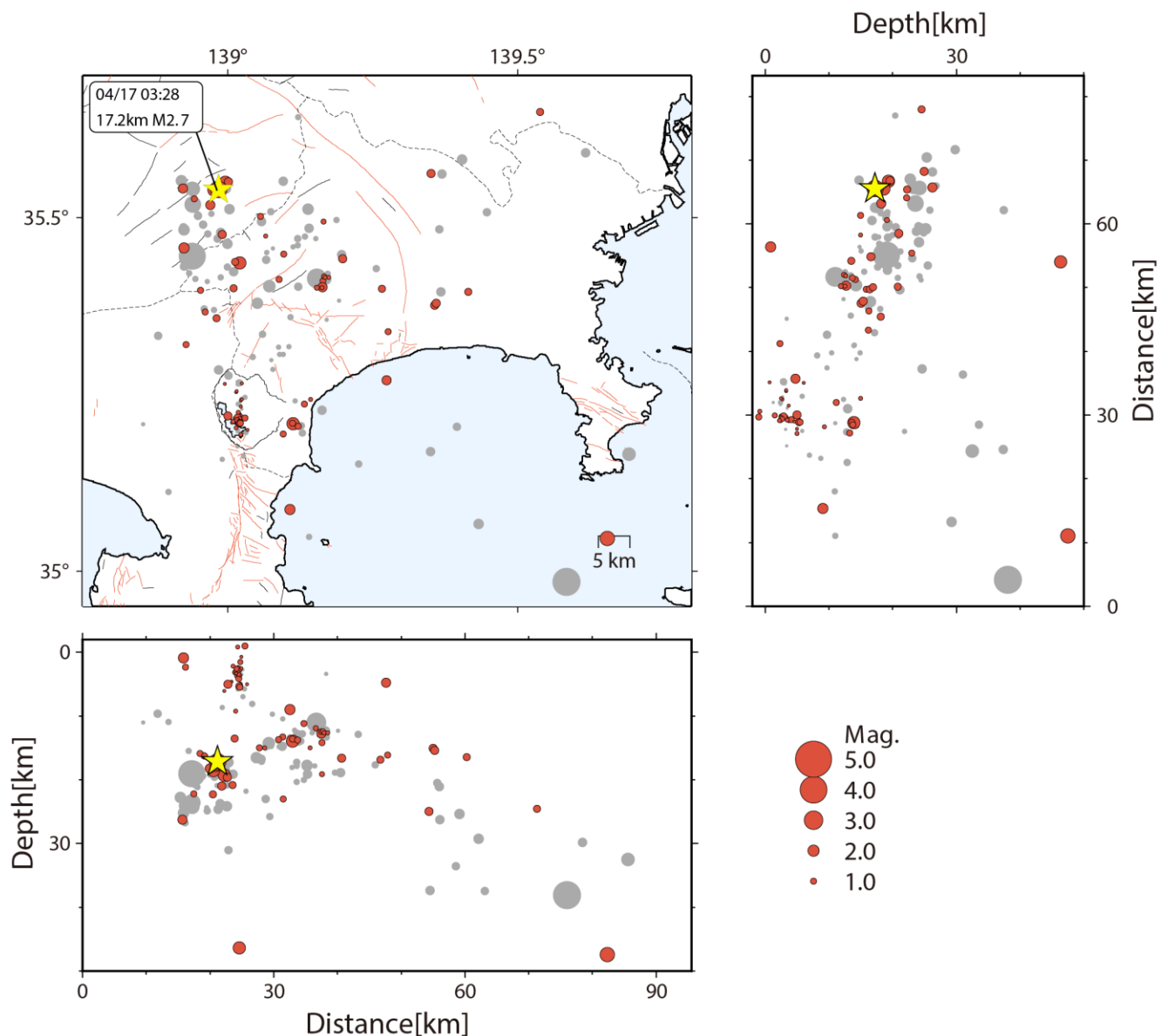
図 1-1 神奈川県とその周辺地域の今月の地震活動。赤の丸印で 2026 年 4 月に発生した地震の震源を示しております。灰色の丸印で 2026 年 2 月と 3 月に発生した地震の震源を示しております。丸印の大きさはマグニチュードに対応します。星印で 2026 年 4 月に図の領域で発生した最大規模の地震の震源を示しております。（震源決定は、当所データの他に東京大学地震研究所、防災科学技術研究所および気象庁の地震波形データを利用しています。）
