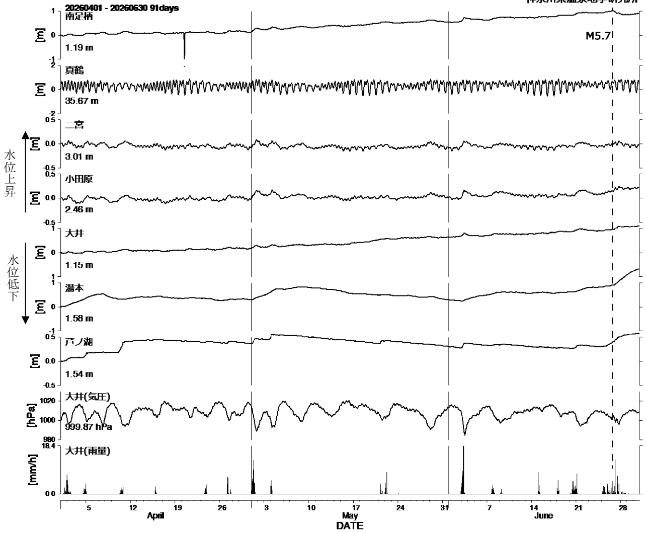
図 5 - 1 地下水水位観測結果 (2026年04月01日~06月30日)
