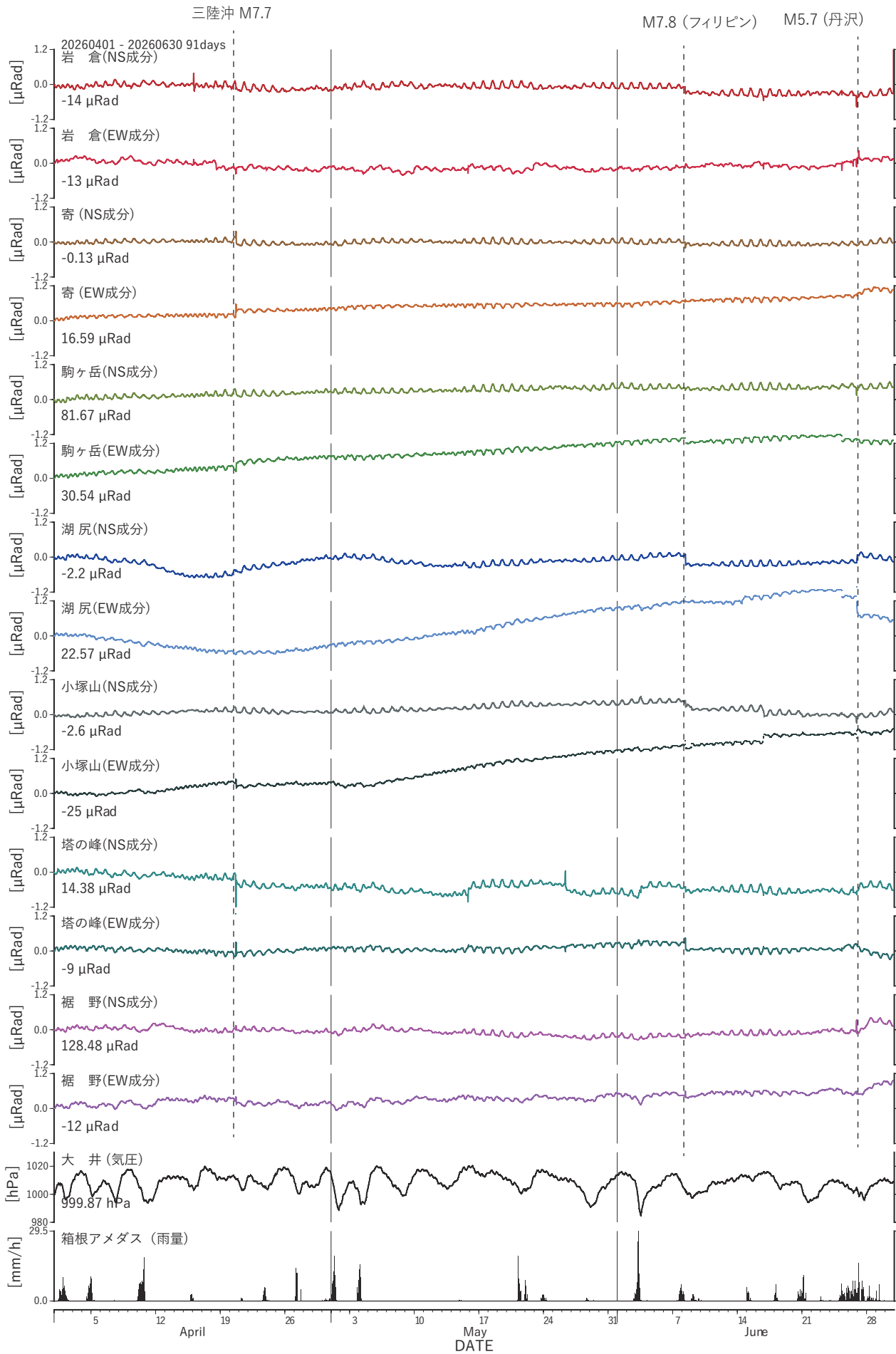
図3 傾斜計記録(2026年04月01日から2026年06月30日)
