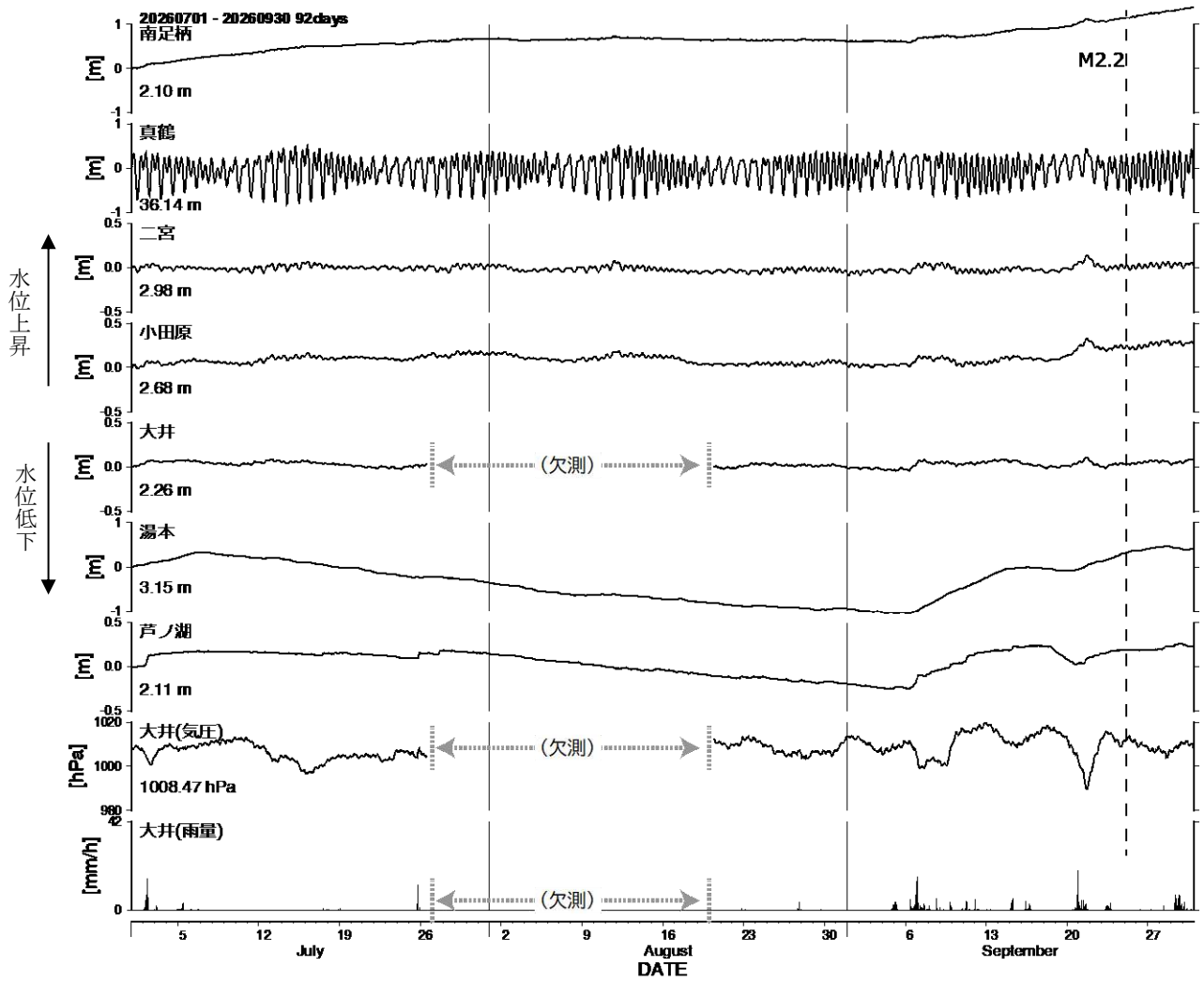
図5 地下水位観測結果(2026年07月01日~09月30日)
