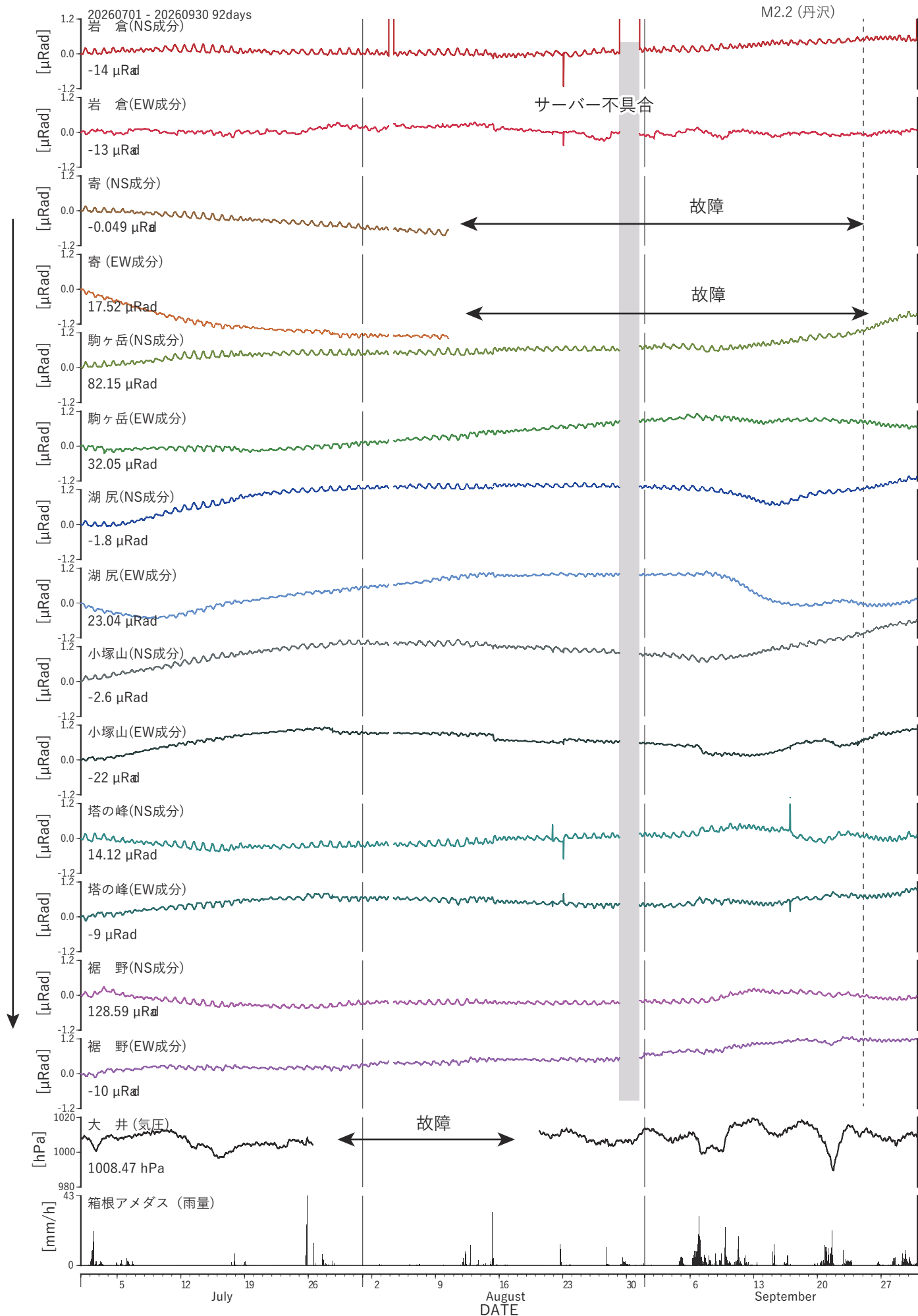
図3 傾斜計記録(2026年07月01日から2026年09月30日)
