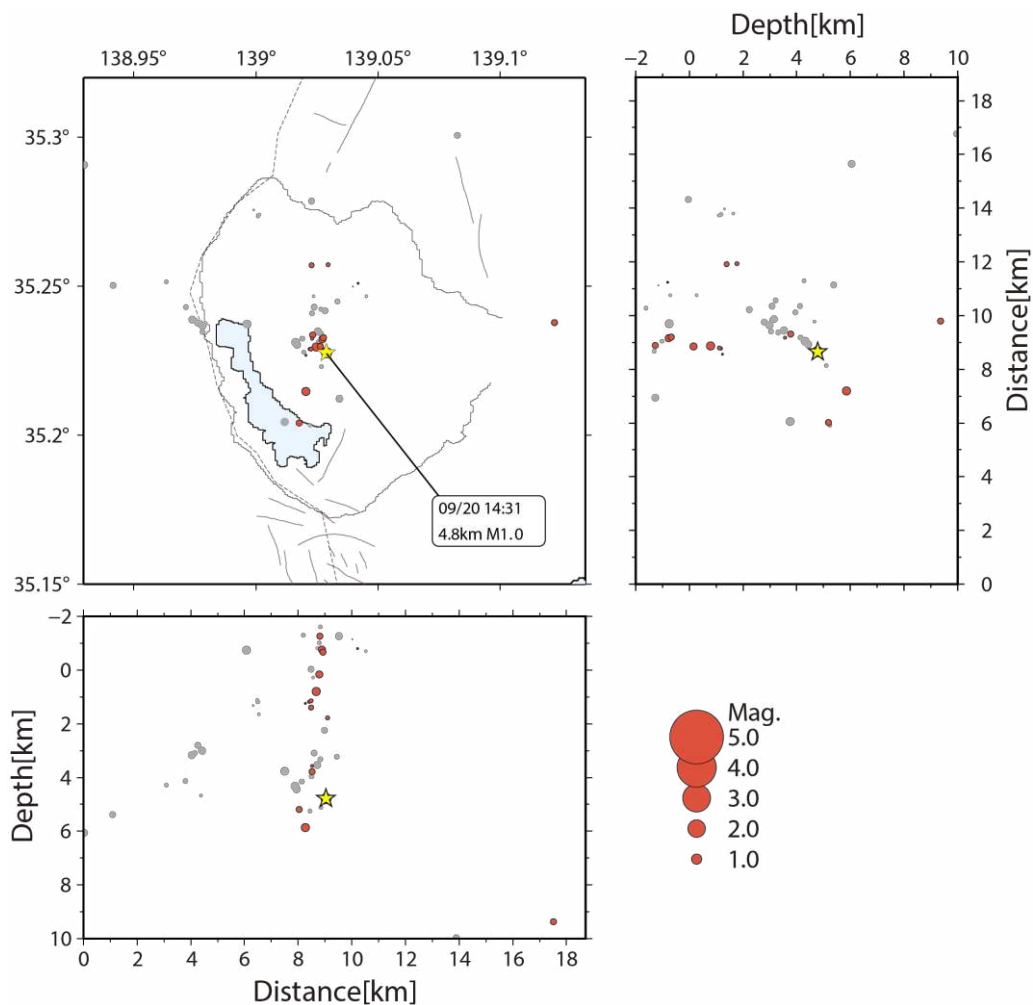
図 1-2 箱根火山の今月の地震活動。赤の丸印で 2026 年 9 月に発生した地震の震源を示しております。灰色の丸印で 2026 年 7 月と 8 月に発生した地震の震源を示しております。丸印の大きさはマグニチュードに対応します。星印で 2026 年 9 月に図の領域で発生した最大規模の地震の震源を示しております。（震源決定は、当所データの他に東京大学地震研究所、防災科学技術研究所および気象庁の地震波形データを利用しています。）
