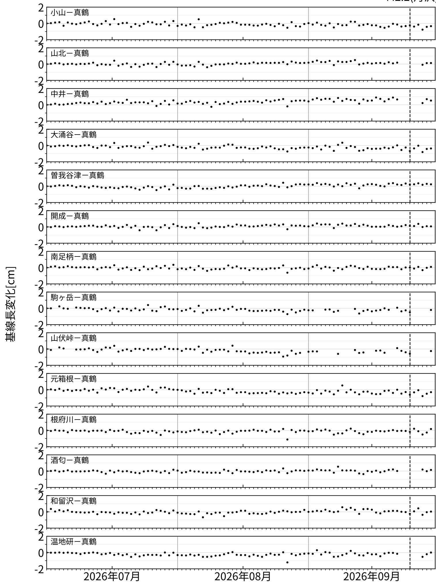
図4 GNSS測量観測結果（2026年7月1日～2026年9月30日）
