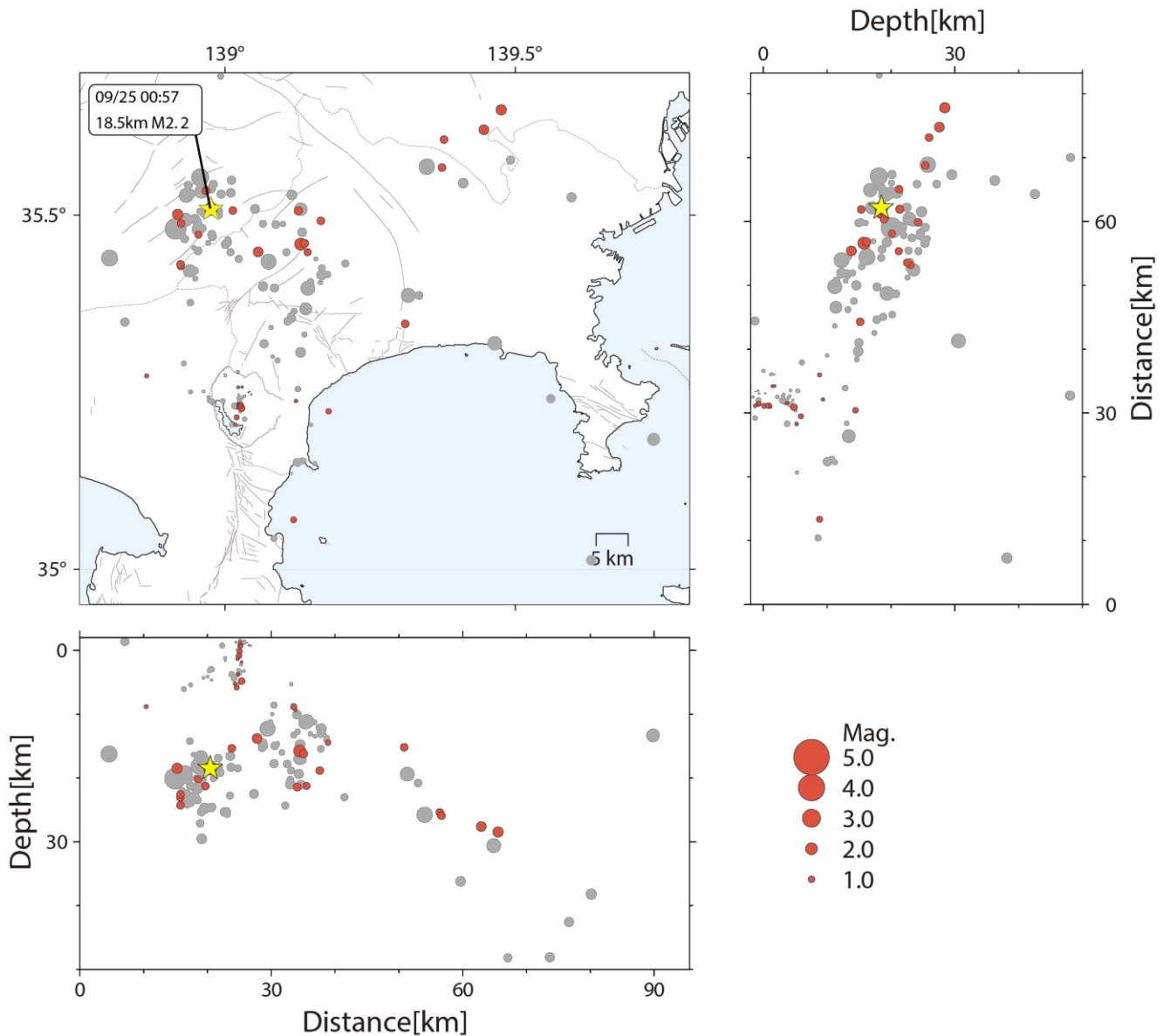
図 1-1 神奈川県とその周辺地域の今月の地震活動。赤の丸印で 2026 年 9 月に発生した地震の震源を示しております。灰色の丸印で 2026 年 7 月と 8 月に発生した地震の震源を示しております。丸印の大きさはマグニチュードに対応します。星印で 2026 年 9 月に図の領域で発生した最大規模の地震の震源を示しております。（震源決定は、当所データの他に東京大学地震研究所、防災科学技術研究所および気象庁の地震波形データを利用しています。）
